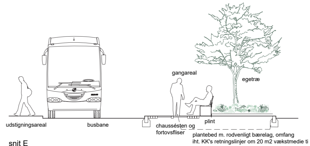
snit E
