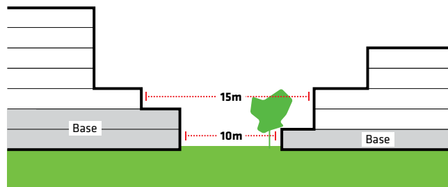
fig. 5.2.d: Indbyrdes minimumsafstande mellem stueetager og øvre etager. i byggefelt A-C.
