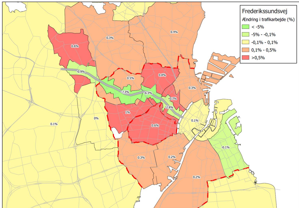
Figur 28 Ændringer i trafikarbejdet som følge af busløsningen på Frederikssundsvej
