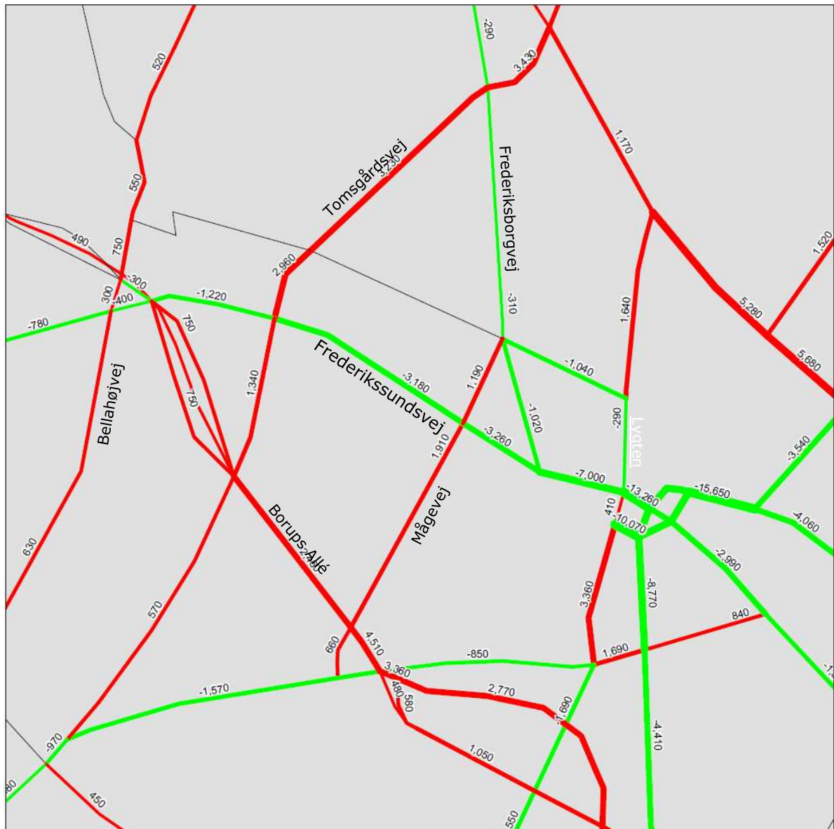
Figur 26 Differensbelastninger mellem udgangssituationen og projektforslaget på Frederikssundsvej på indre strækning . Grøn: Aflastning, Rød: Merbelastning. Biler/døgn.
