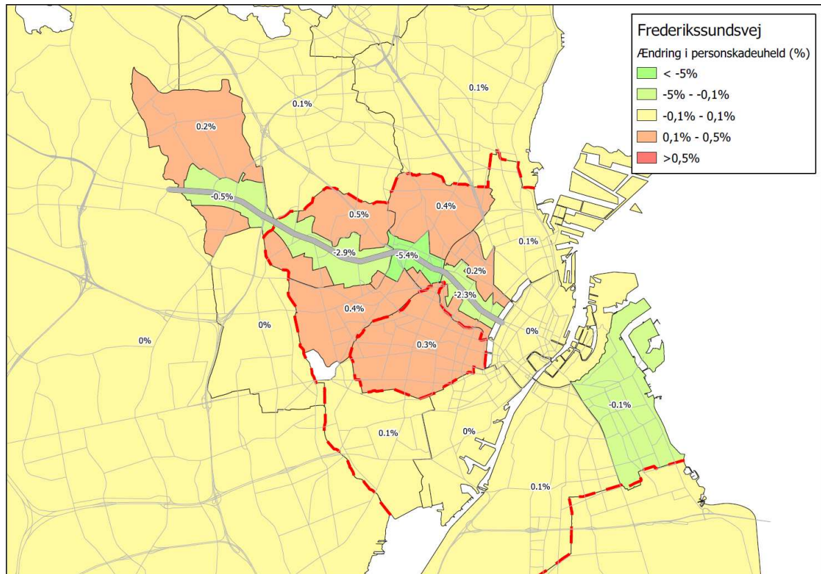
Figur 31 Ændring i personskadeuheld
