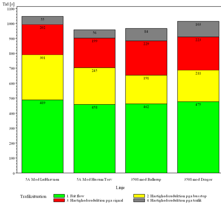
Figur 24 Rejsetidens bestanddele for busserne, her vist i en eftermiddagssituation i eksisterende situation.
