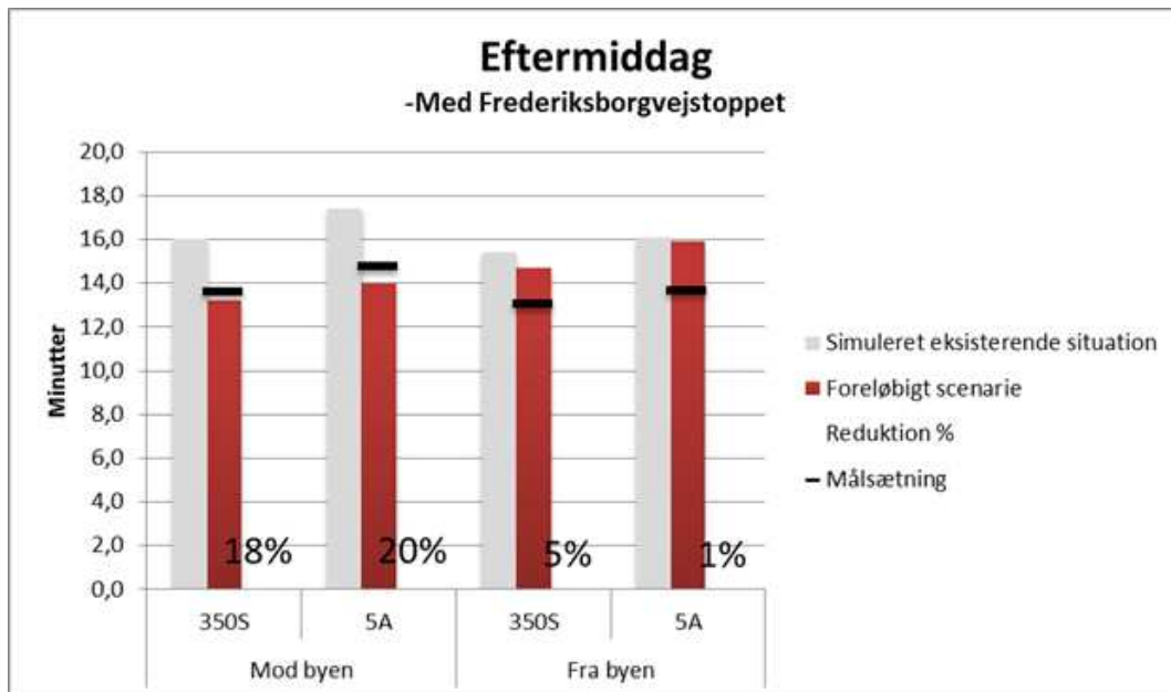
Figur 20 Resultater for rejsetid – eftermiddag.
