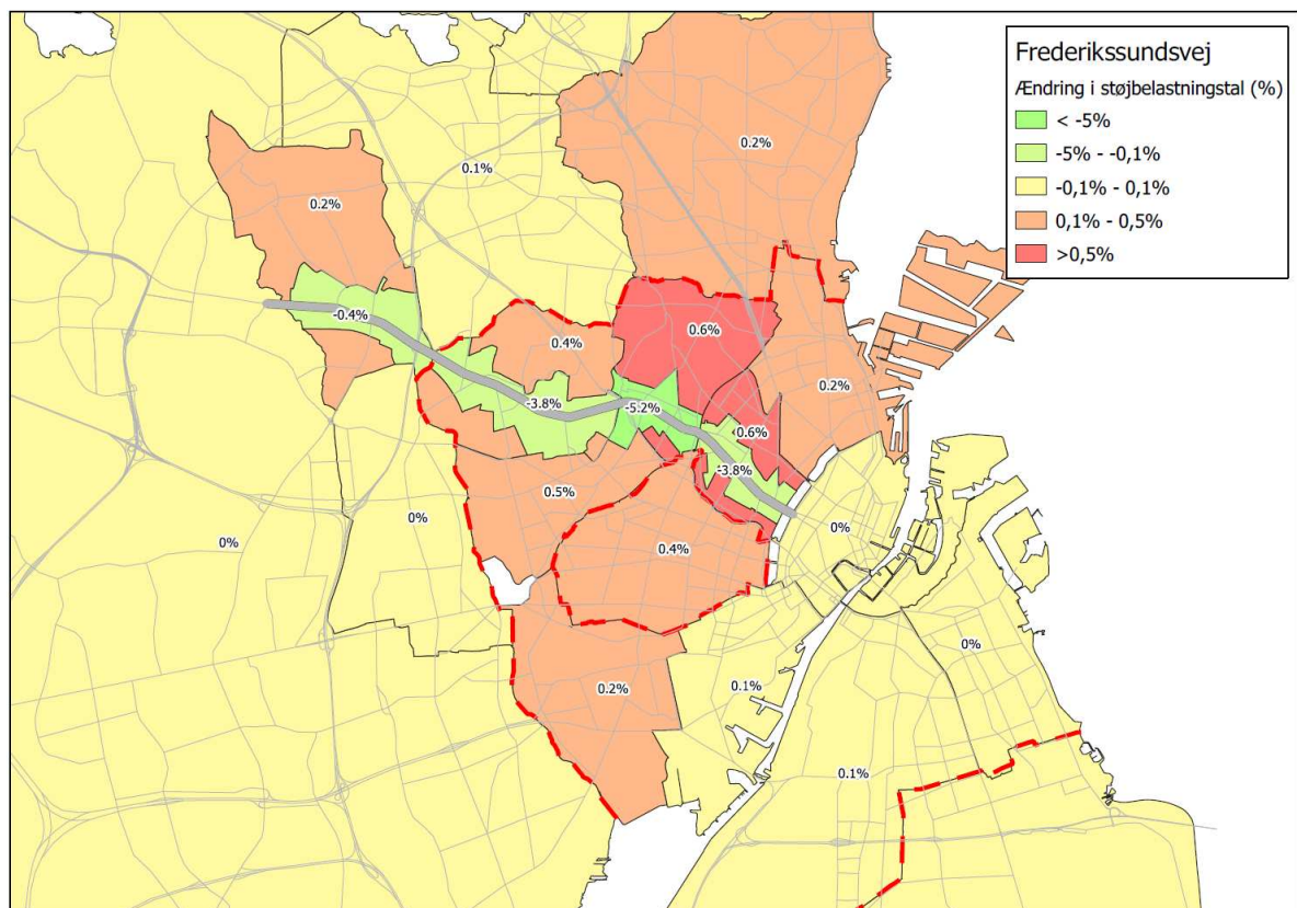
Figur 29 Ændring i støjbelastningstal
