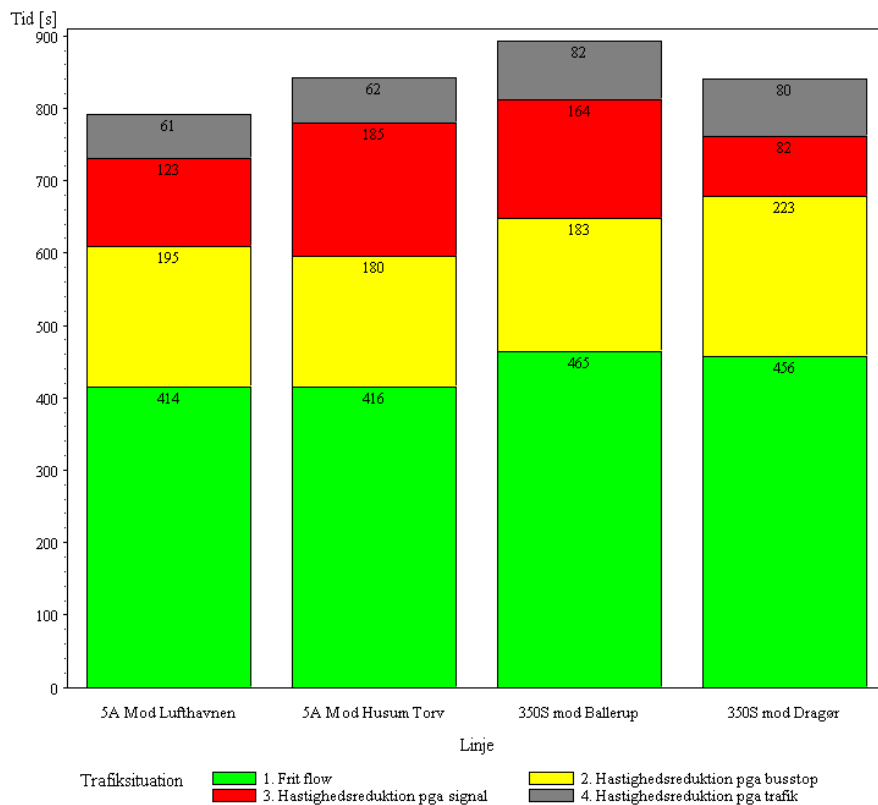
Figur 25 Rejsetidens bestanddele for busserne, her vist i en eftermiddagssituation for projektforslaget
