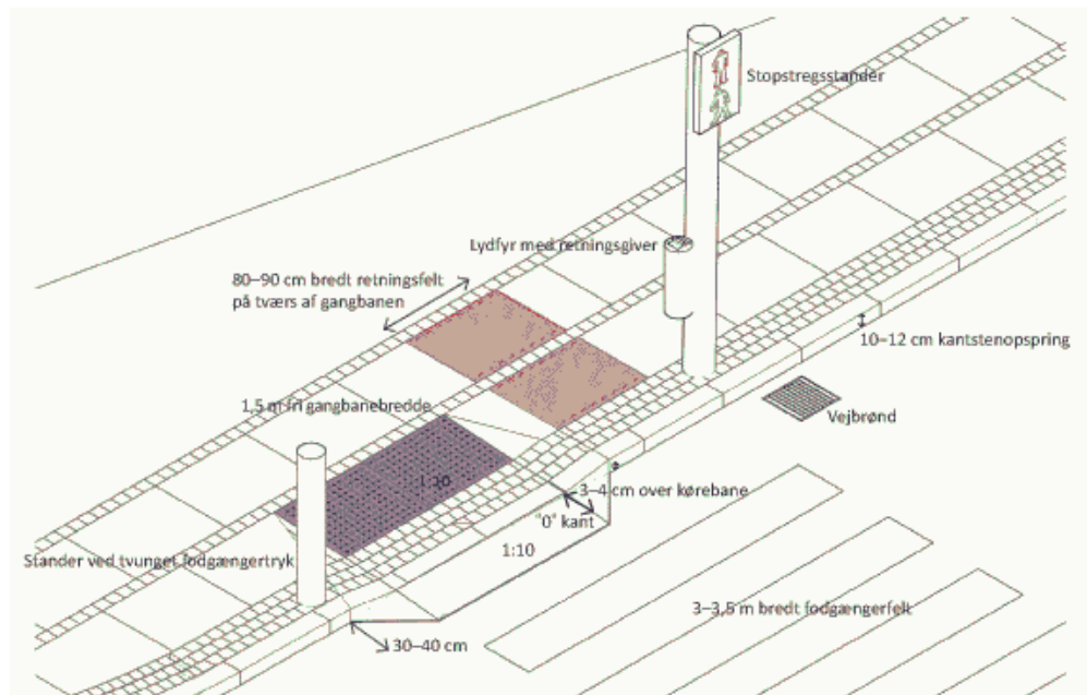
Figur 16 Principtegning af opmærksomhedsfelt og retningsfelt ved fodgængerovergang, Færdselsarealer for Alle 2013.
