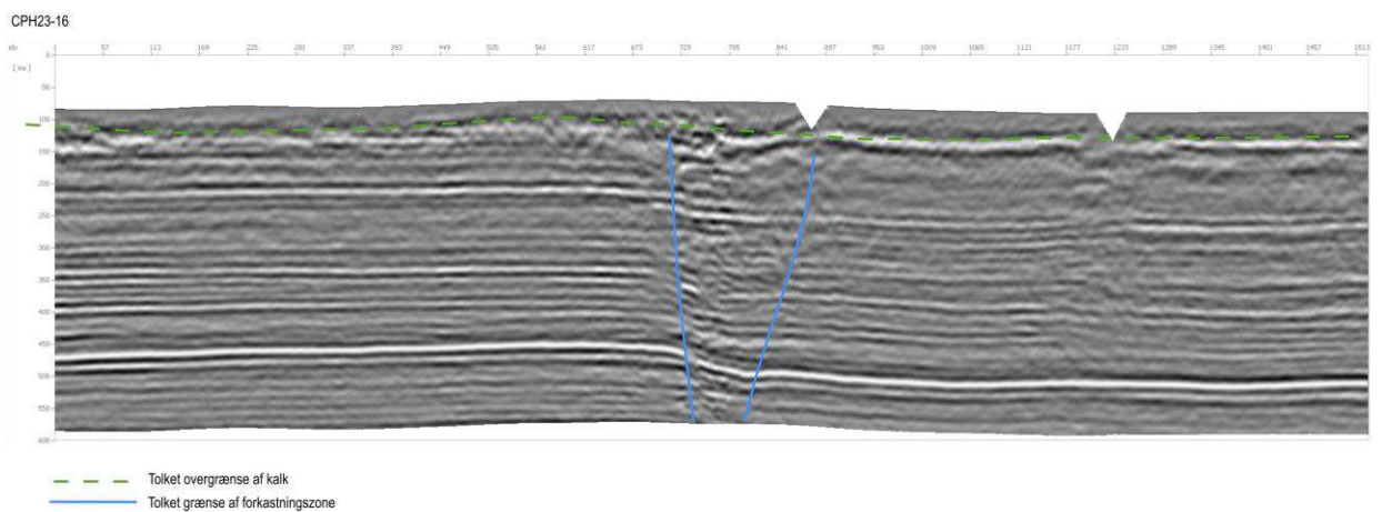
Figur 6. De reprocesserede seismiske linjer med indtegnede tolkninger af Carlsbergforkastningen (blå linjer) og overgrænsen af kalk (grøn stiplede linje).
