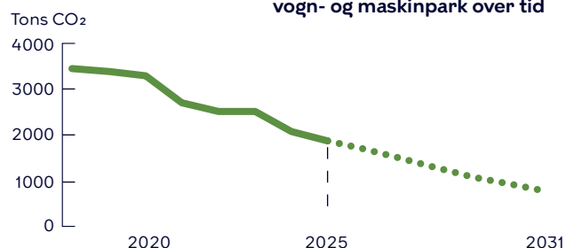
Figur 34 CO 2 -udledning i Københavns Kommunes vogn- og maskinpark over tid
