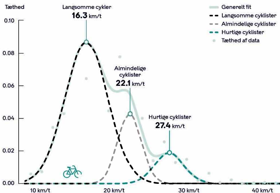
Figur 13 Hastighedsfordeling for cyklister. Grafen viser tætheden af cyklisteres hastigheder (km/t) opdelt i tre grupper: langsomme, almindelige og hurtige cyklister
