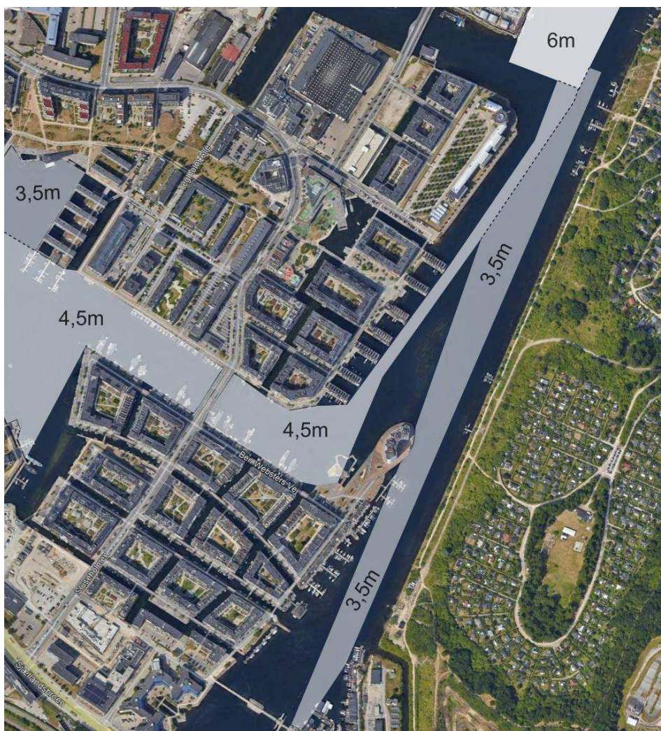
Figur 3-5 Garanteret sejldybder i Teglværkshavnen
