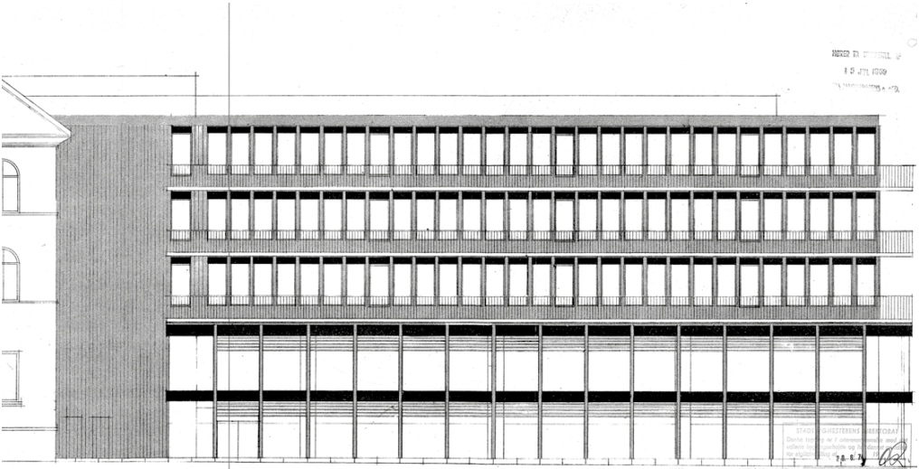
Bremerholm 33 set fra Laksegade - oprindelig facadetegning 1969
