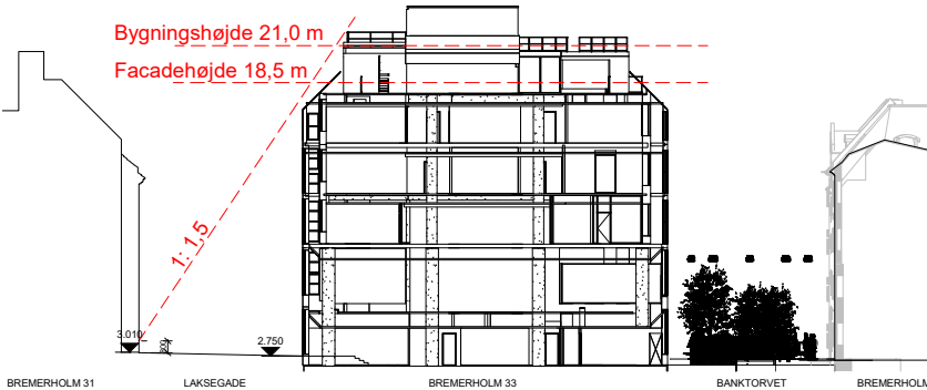
Bremerholm 33 - tværsnit - nuværende forhold
