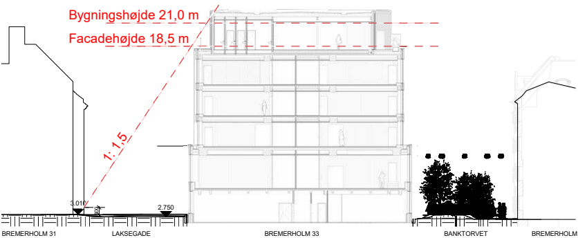
Bremerholm 33 - tværsnit - fremtidige forhold
