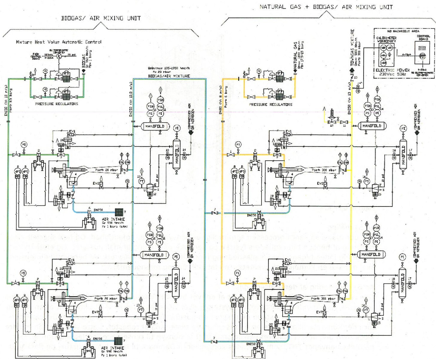
Figur 5: Nyt biogasproduktionsanlæg
