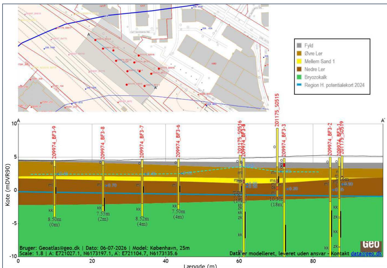
Figur 1 Geologisk profil fra GeoAtlas Live med borer og pejlinger vist. Det terrænnære grundvandspejl er markeret med turkis stiplede linje. Det forventede potentiale for det primære grundvandspejl er vist med blå linje.
