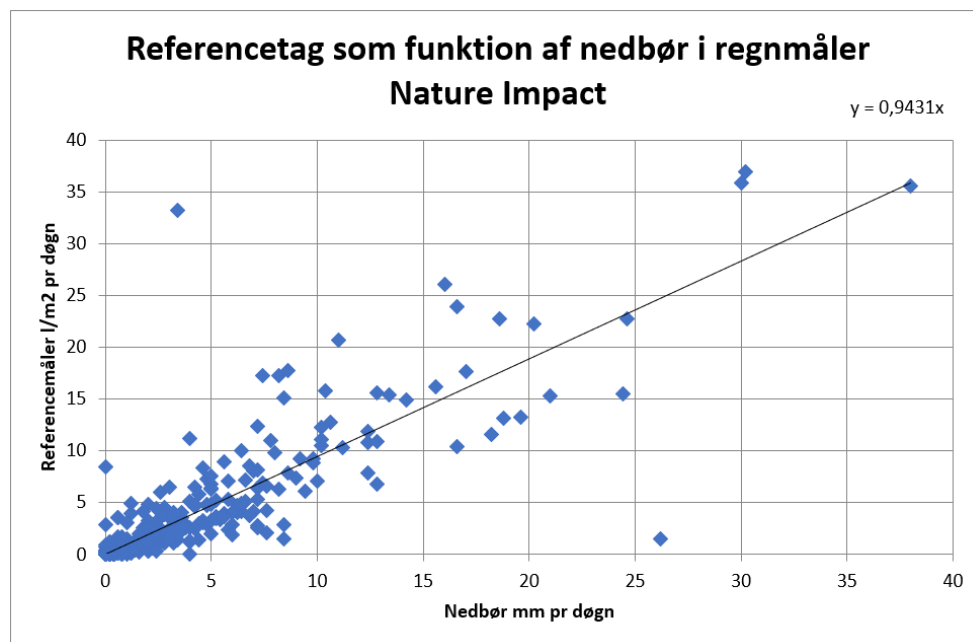
Figur 3-5 Døgnaflstrømning fra referencetaget hos Nature Impact som funktion af døggnedbøren.
