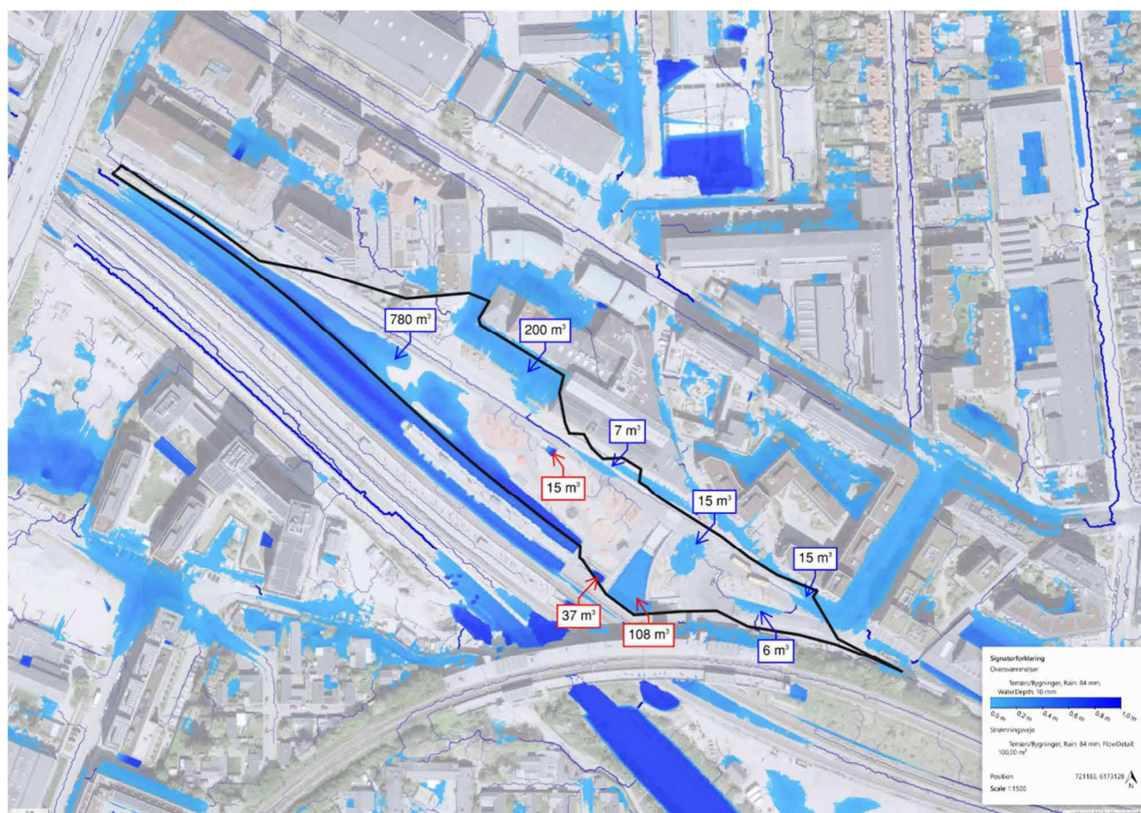
Figur 12 – Scalgoanalyse ekstremregn, opmagasinerings eksisterende forhold
