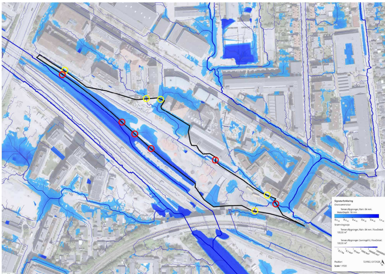
Figur 7 – Scalgoanalyse ekstremregn, strømningsveje eksisterende forhold
