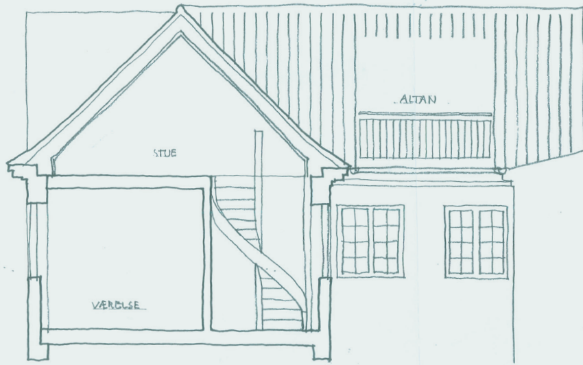
SNIT I FORHUS
