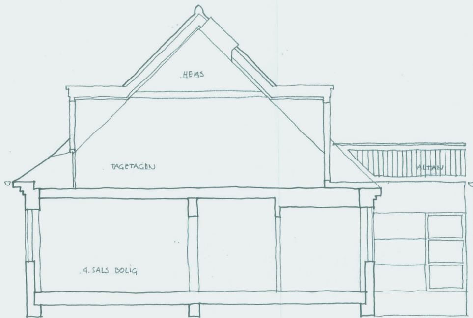
SNIT I HOVEDBYGNING
