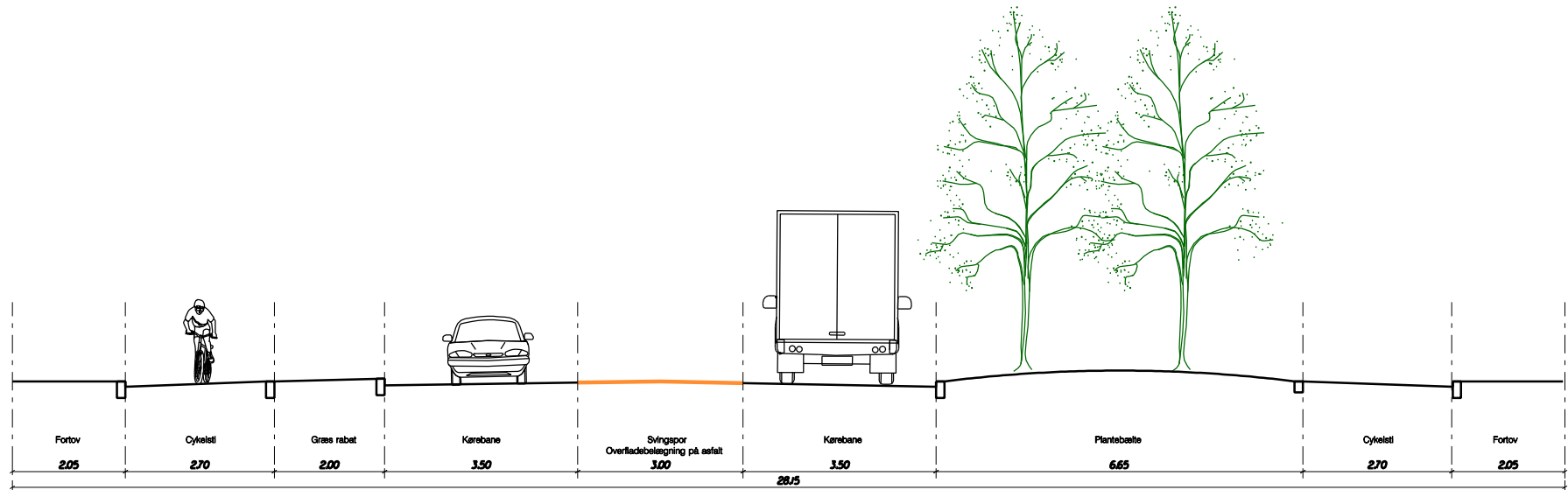
Fremtidigt tværprofil
