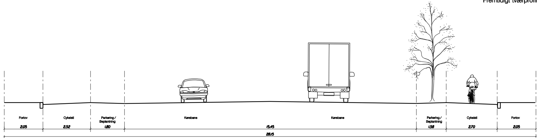
Eksisterende tværprofil
