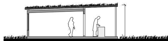
Principsnit 1:100
