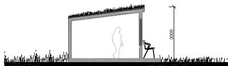
Principsnit 1:100.
