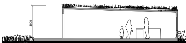
Principsnit 1:100
