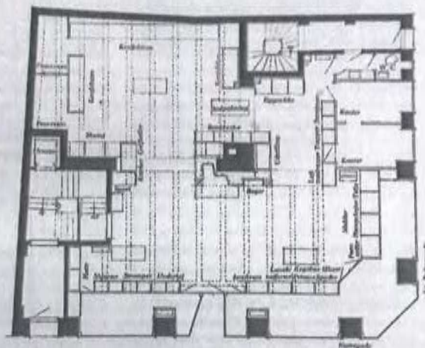
Sven Risom: Forretningsbygning paa Nørregade (Hjørnet af Skt. Peders Stræde) Plan af Butik i Stueetage 1:100
