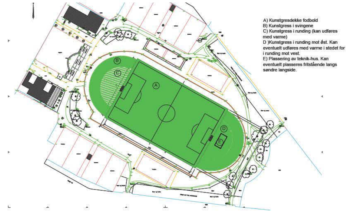
Figur 8b: Sommerdrift
