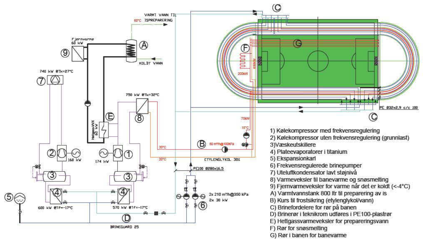
Figur 4b: Principskema over kuldeanlæg og brine, med banevarme
