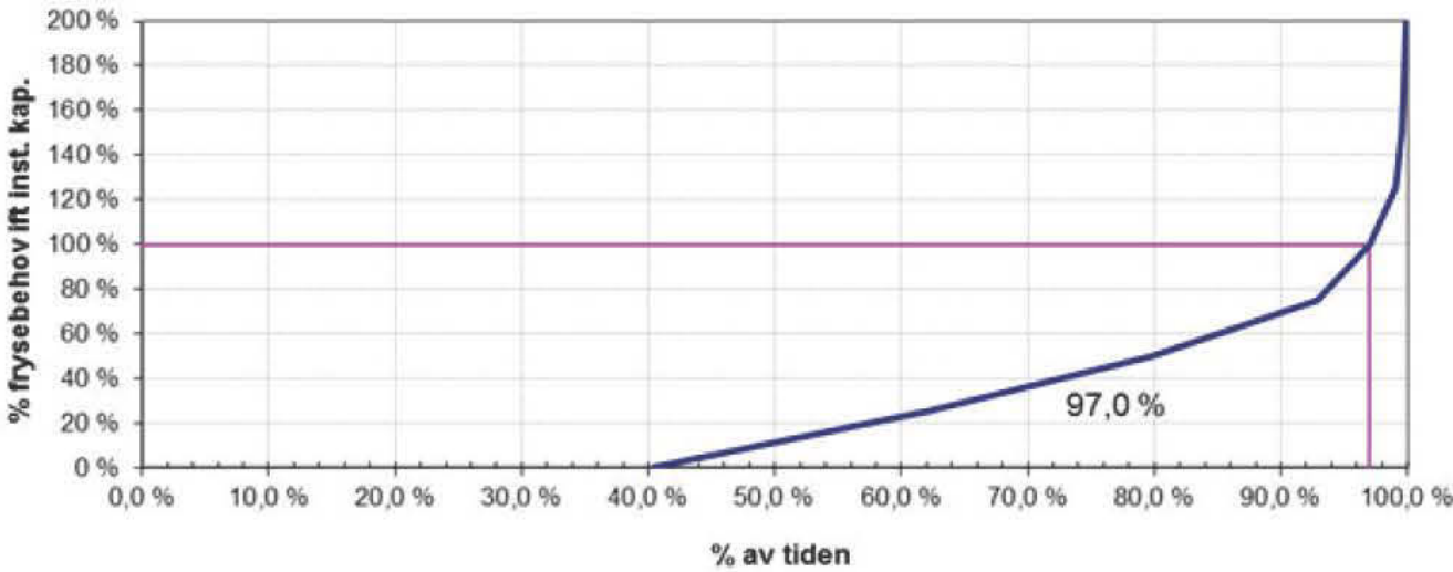
Figur 5b: Installeret frysekapacitet på 250W/m² for at holde banen frosset. Mindst 97% af tiden vil det være tilstrækkeligt i et normalår. Forudsat drift fra 1. november til 28. februar (=100% tid).
