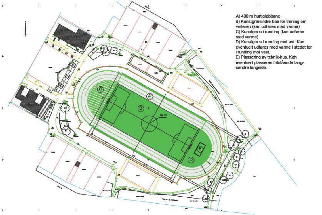
Figur 8a: Vinterdrift
