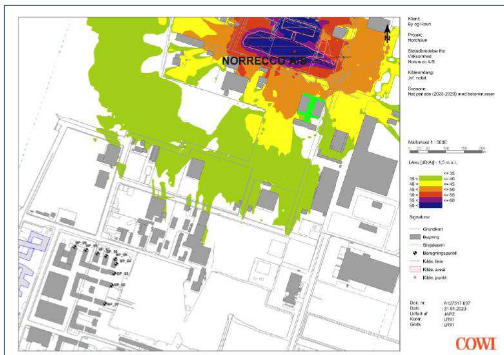
Figur 6-5 Støjudbredelseskort for ekstern støj fra virksomheden Norrecco – natperiode (2023-2029) med betonknuser (COWI, Vurdering af støj for Svanemølleholm Øst, 2024).
