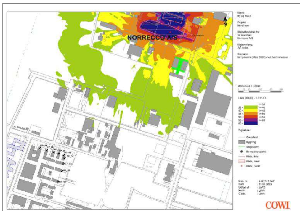
Figur 6-6 Støjudbredelseskort for ekstern støj fra virksomheden Norrecco – natperiode (efter 2029) med betonknuser (COWI, Vurdering af støj for Svanemølleholm Øst, 2024).
