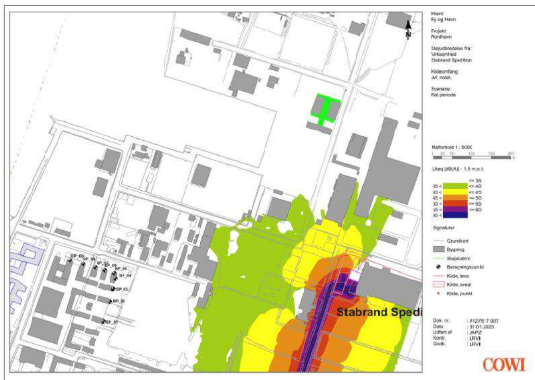
Figur 6-8 Støjdbredelseskort for ekstern støj fra virksomheden Stabrand Spedition ApS – natperiode (COWI, Vurdering af støj for Svanemølleholm Øst, 2024).
