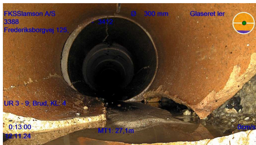
Billede 3. Brud på kloakrør
