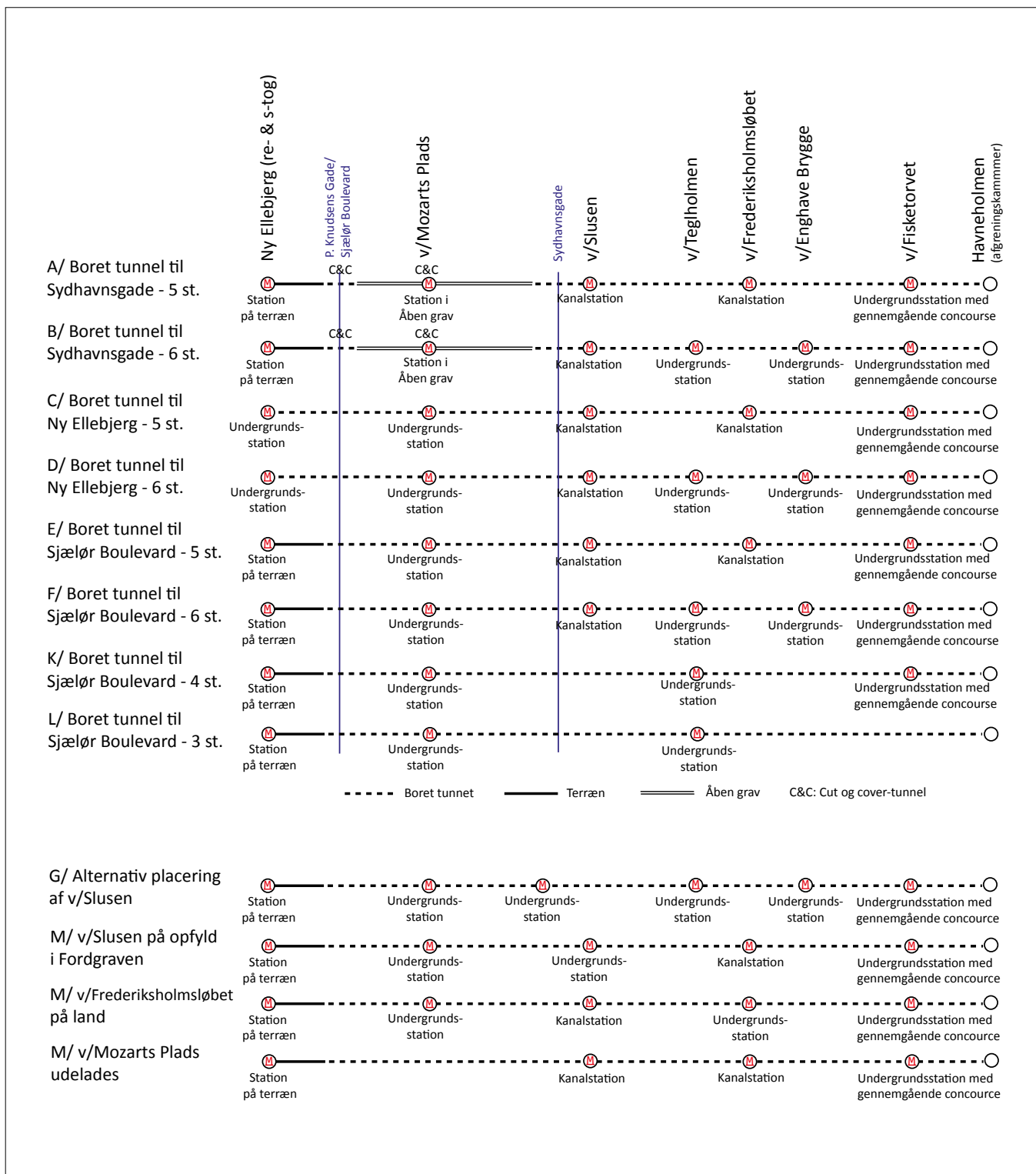
Figur 5.5 Oversigt over udredningen scenarier A-F og K-L med angivelse af antal stationer og stations-typer samt skitsering af længden af den borede tunnel.
