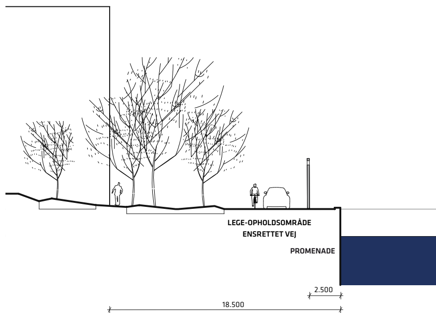
Snit L-L
