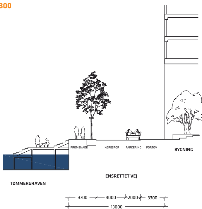
Snit C-C
