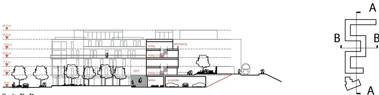
Snit B-B
