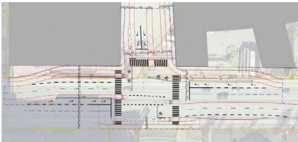
Figur 3-5 Ny krydsudformning for det signalregulerede kryds ved Belvederekanalen/Vasbygade. I krydset er der tilføjet svingbaner på Vasbygade ind til Jernbanebyen, og desuden tilføjet en ligeud cykelsti. Krydsudformningen anvendes i Scenario 2035.
