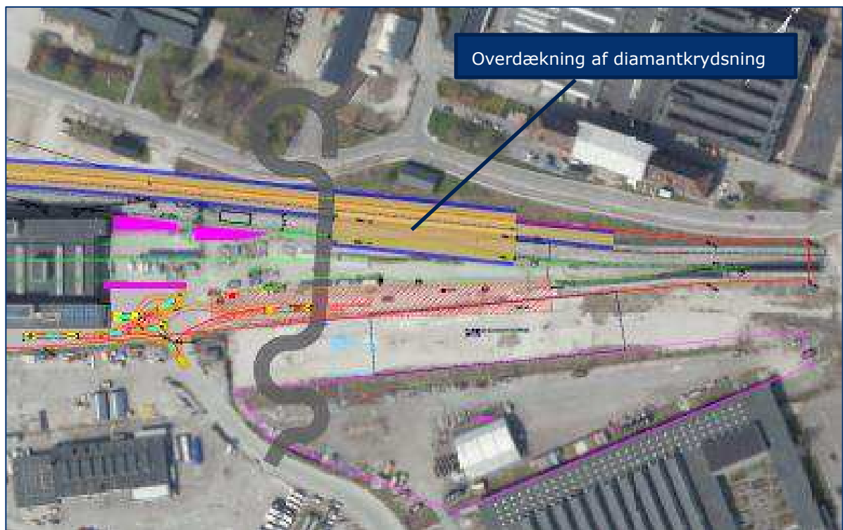
Figur 13-5. Placering af overdækning af diamantkrydsning.
