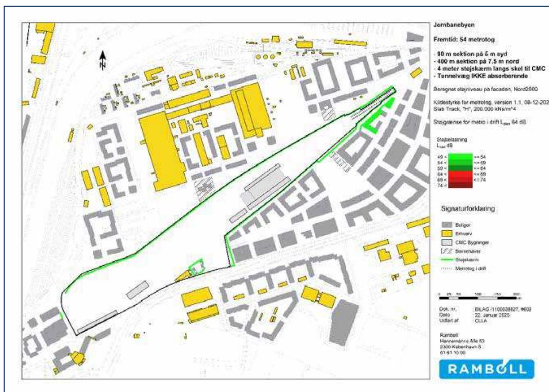
Figur 21-1. Støj i driftsfasen for metrotog som kører med 40 km/t ned mod tunnelåbning og 40 km/t op fra tunnelåbning. Støjgrænse for metro i drift er L_{den} 64 dB for boliger.
