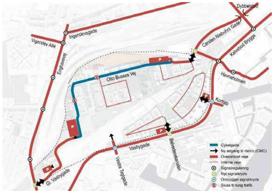
Figur 1-7 Vejnet til trafikberegningen i OTM.
