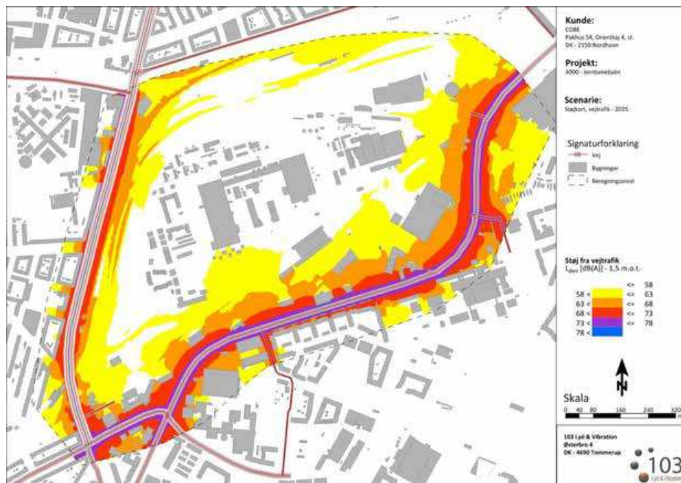
Figur 10-12 Støjbreddelseskort for vejtrafikstøj – basisscenarie 2035 uden udvikling af Jernbanebyen. (Kort: 103 Rådgivende Ingeniører).
