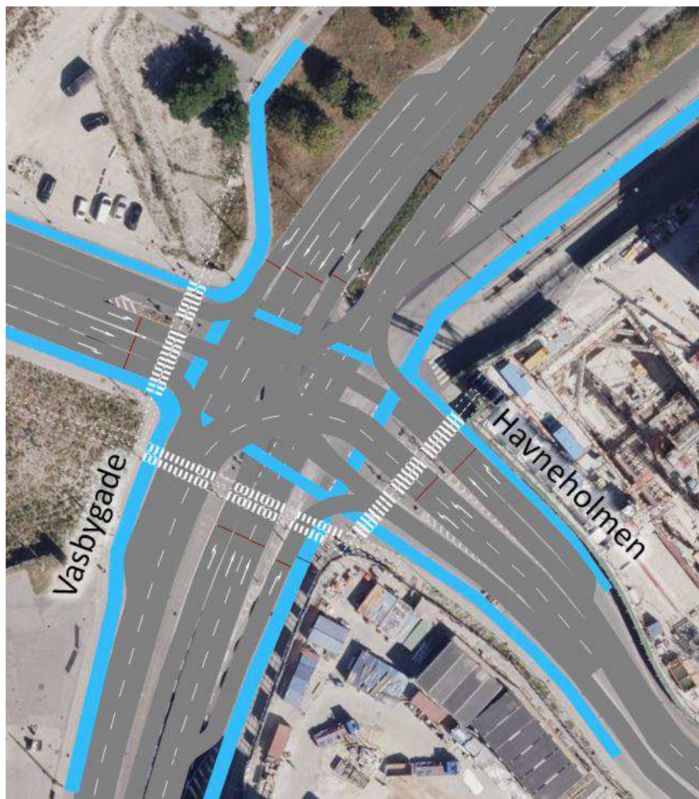
Figur 6-14 Krydset Vasbygade/Havneholmen i Basis 2019 (Udklip fra VISSIM-modellen). Samtlige resultater for krydset kan ses i Bilag C.11.
