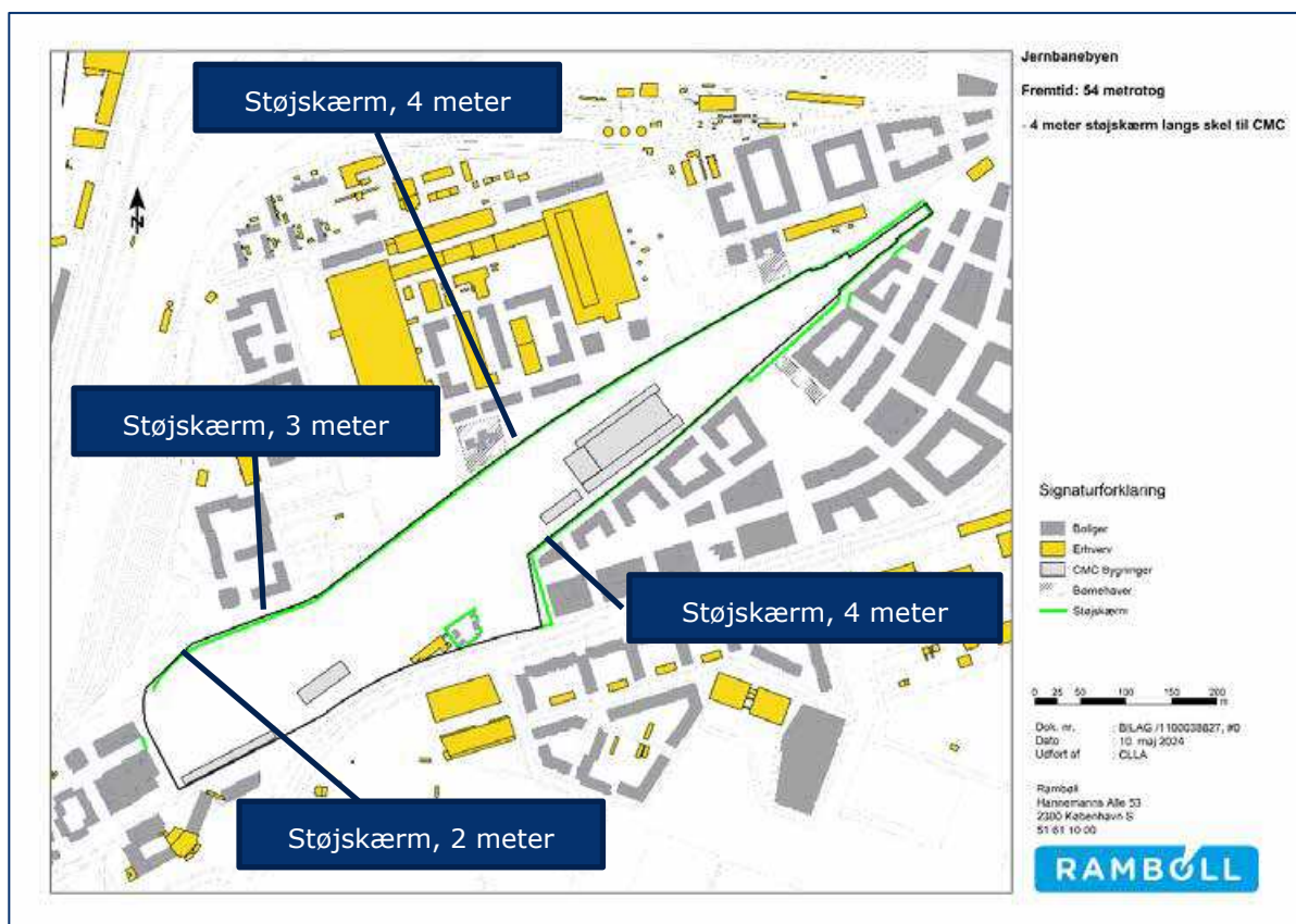
Figur 13-1. Placering af 4 meter høje støjskærme (grøn line). Der er forudsat, at skærmene placeres ved skel til naboejendomme. Skærmens topkote skal være 4,0 meter over nærmeste skinneoverkant. Mod sydvest falder støjskærmens højde til henholdsvis 3 meter og 2 meter.
