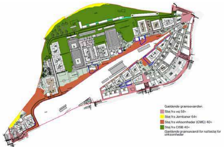
Figur 7-1 Jernbanebyen. Oversigtskort over støjudbredelse af støj i delområderne fra veje, jernbaner, CMC og andre virksomheder. Der er kun vist støjudbredelse for områder, hvor støjniveauet er beregnet over Miljøstyrelsens vejledende grænseværdier for støj på udendørs opholdsarealer.
