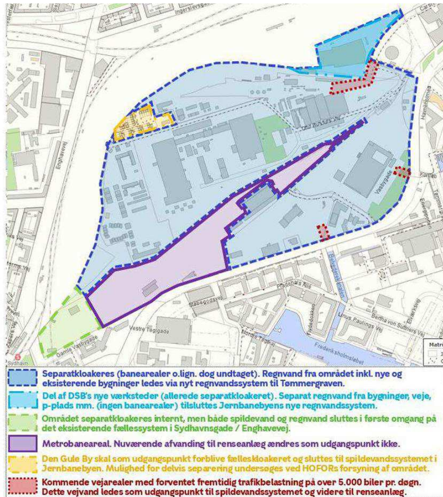
Figur 4-21 Plan for fremtidig håndtering af regn- og spildevand (Spildevandsplanen). Kilde Københavns Kommunes Spildevandsplan 2018, tillæg 2024 Bilag 2, projekt B.118.
