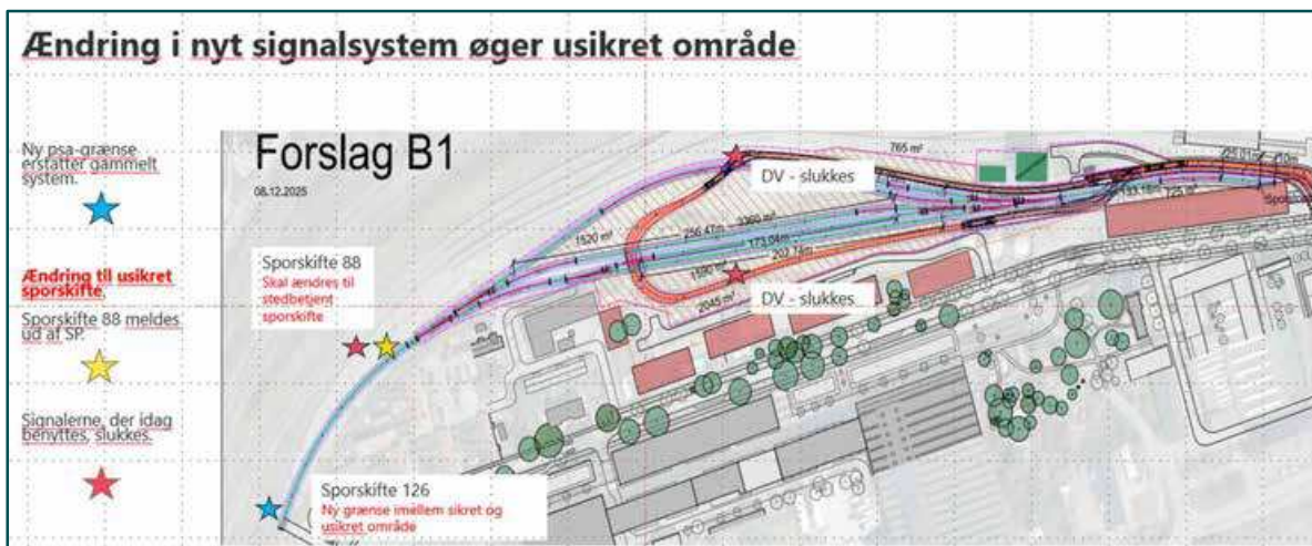
Figur 10: Udvidelse af det usikrede område til base formål og markering af ændringer fra hidtidige signaler til implementering af det nye signalsystem.
