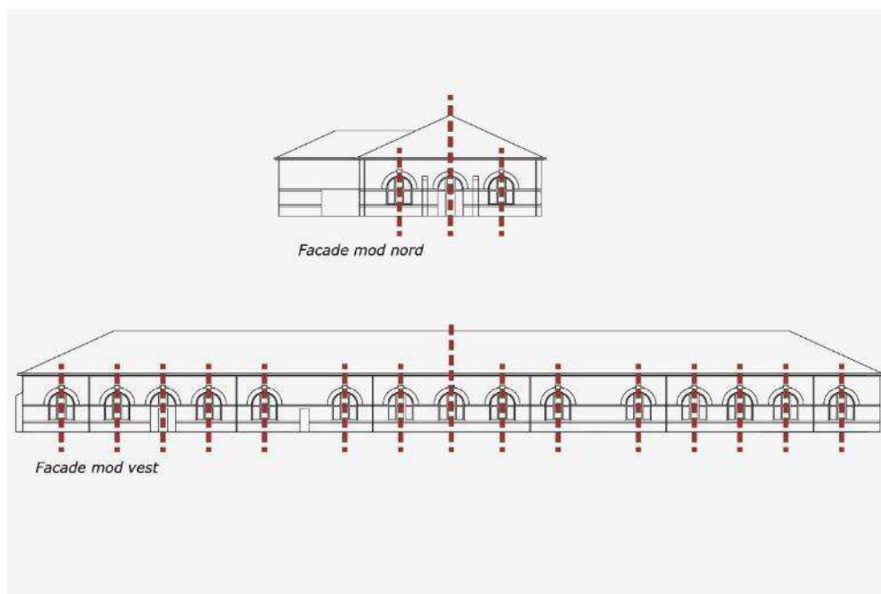
Figur 5-72 Blanketlageret vestfacade. De lodrette stiplede linjer viser facadens rytme. I centrum ses akse som spejler facaden. Tegning Cobe.
