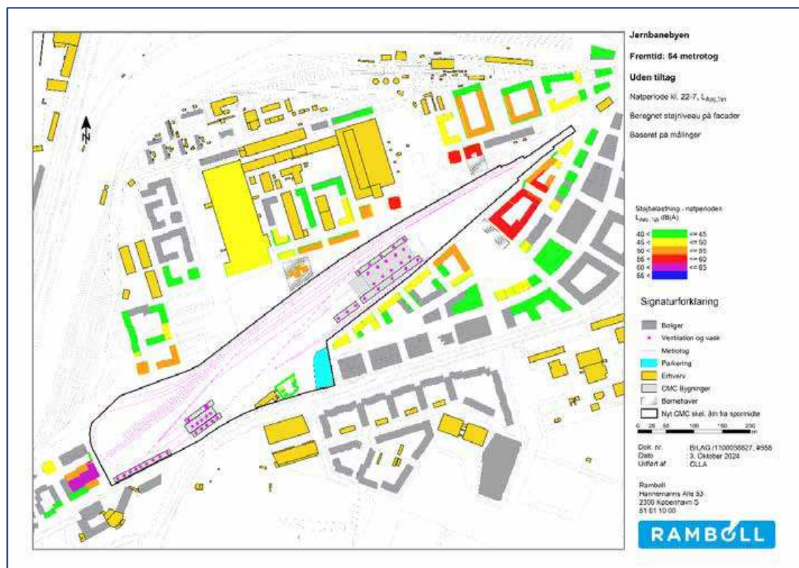
Figur 20-6. Scenarie: Uden støj dæmpende tiltag. Beregnet støjniveau på facaden i natperioden. Grå bygninger er udsat for støj med niveauer under 40 dB.
