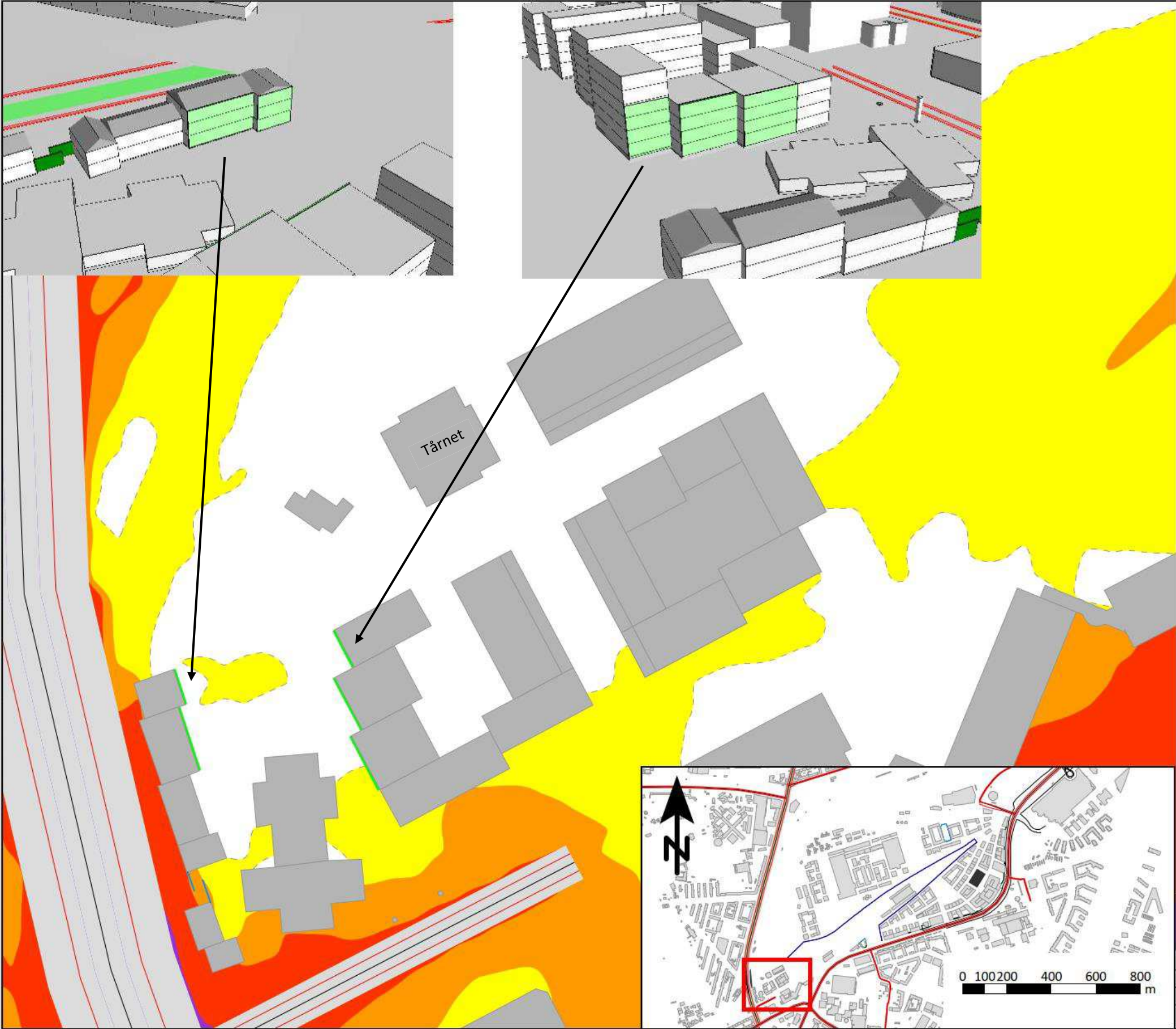
Beregningsresultater i Delområde 3 – Vejtrafik-støjudbredelseskort i 1,5 m over terræn
