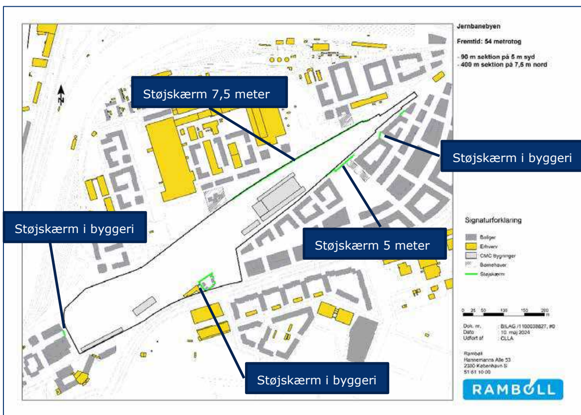
Figur 13-2. Placering af 5 og 7,5 meter høje støjskærme (grøn line). Der er forudsat, at skærmene placeres ved skel til naboejendomme. Skærmens topkote skal være 5 og 7,5 meter over nærmeste skinneoverkant. "Skærm i byggeri" indgår den mulige byudvikling og vedrører ikke mulige løsninger på CMC.
