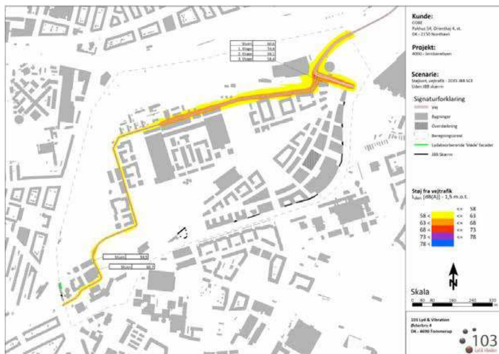
Figur 10-15 Støjudbredelseskort for vejtrafikstøj fra interne veje – drift i scenarie 2035. (Kort: 103 Rådgivende Ingeniører).
