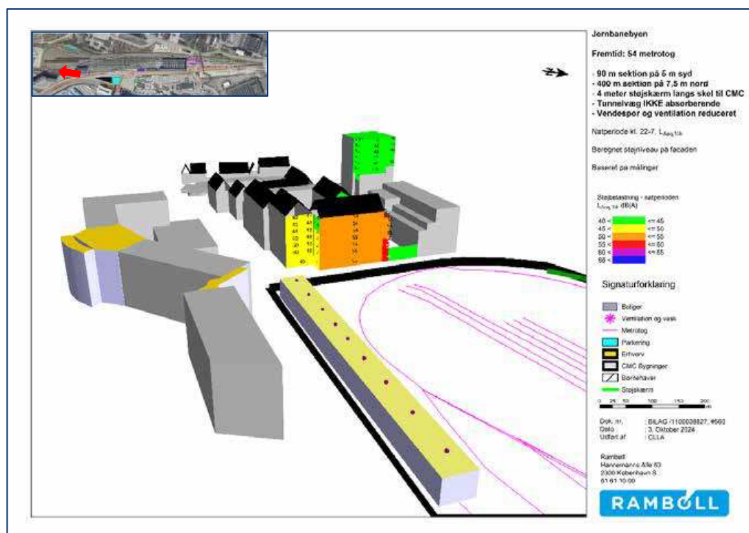
Figur 20-26. Scenarie: Reduceret støj uden overdækning. 3D opstalt af beregnet støjniveau på facaden i natperioden. Grå facader er udsat for støj med niveauer under 40 dB. Bygninger sydvest for loop.
