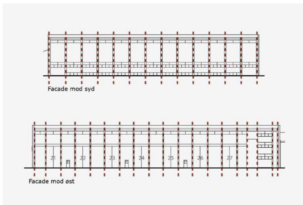
Figur 5-122 Ny eftersynshal. Illustrationen viser rytmen i syd og østfacaden. Tegning Cobe.
