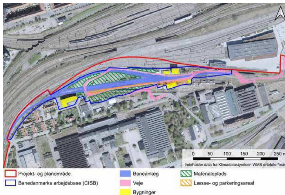
Figur 4-19 Skitseløsning for disponering af areal til Banedanmarks arbejdsbase (CISB). (Kort: COWI)
