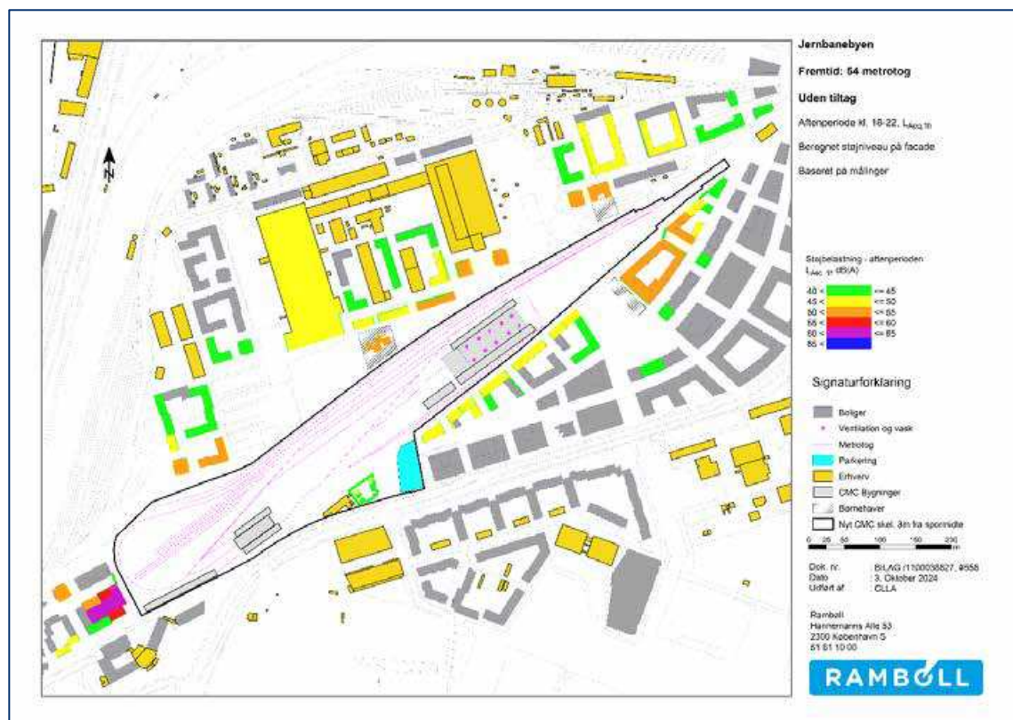
Figur 20-4. Scenario: Uden støj dæmpende tiltag. Beregnet støjniveau på facaden i aftenperioden. Grå bygninger er udsat for støj med niveauer under 40 dB.
