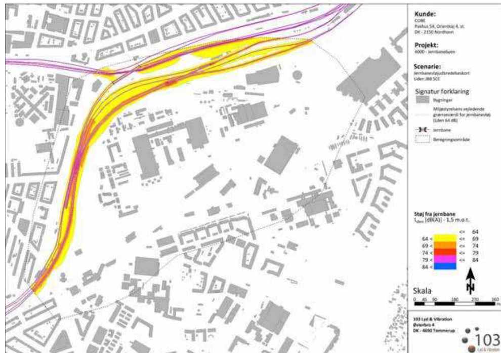
Figur 10-4 Støjudbredelseskort jernbanestøj – eksisterende forhold. (Kort: 103 Rådgivende Ingeniører).
