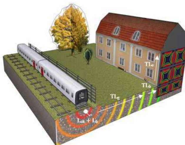
Figur 9 Principet bag Banedanmarks Vibrationsmodel.
