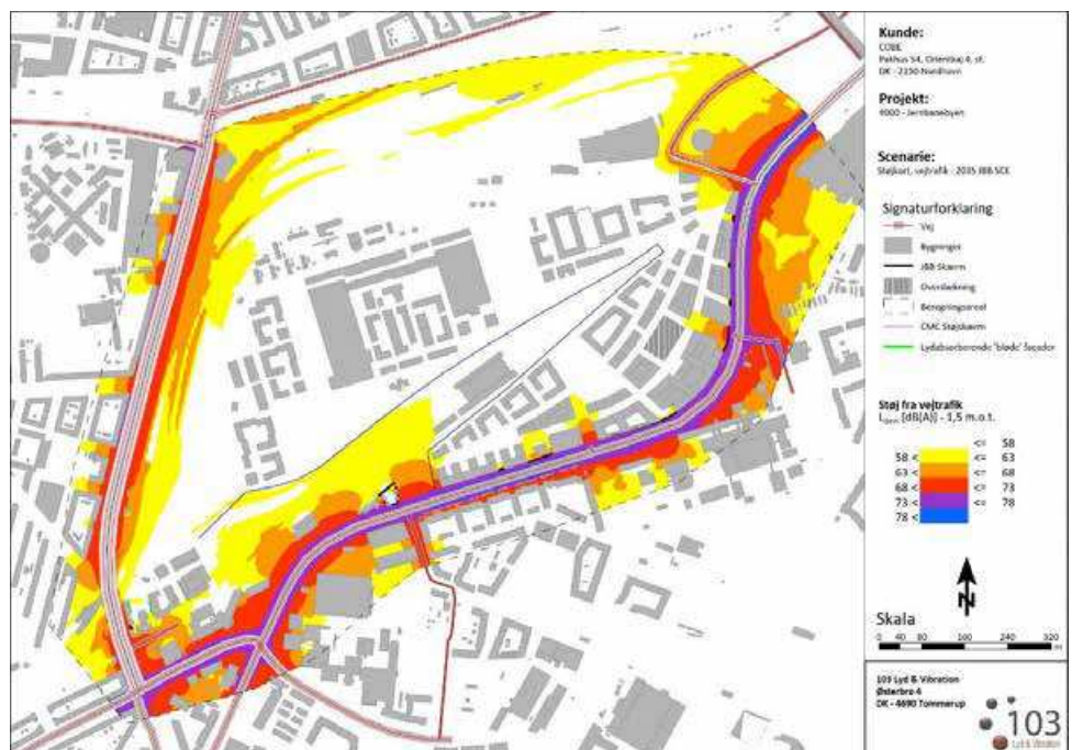
Figur 6-1 Støjudbredelseskort vejtrafikstøj 1,5 meter over terræn for fremtidigt scenario med udbygning af Jernbanebyen 2035 (103) med støjskærme etableret langs Vasbygade og Enghavevej.
