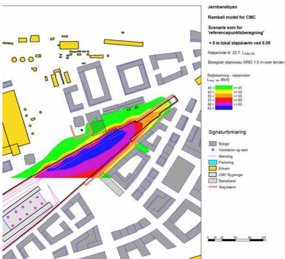
Figur 3. Delområder 6. Lokal afskærmning ved byggefelt 6.09. Skærmhøjde 5 m
