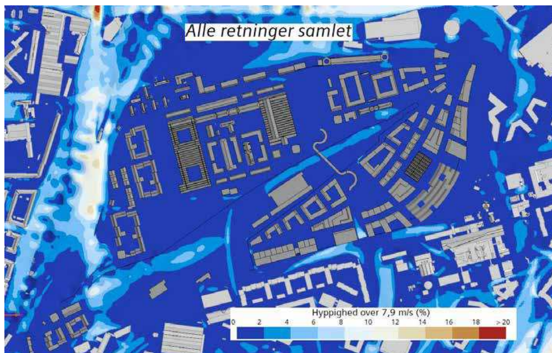
Figur 4.7 Hyppighed for overskridelse af 7,9 m/s beregnet 1,5 m over gadeniveau i Jernbanebyen. Alle vindretninger, årsklima. Beregnet ud fra Weibull-parametrene og hyppighederne i Tabel 3.1. Aktivitet: gang/slentren (4%).
