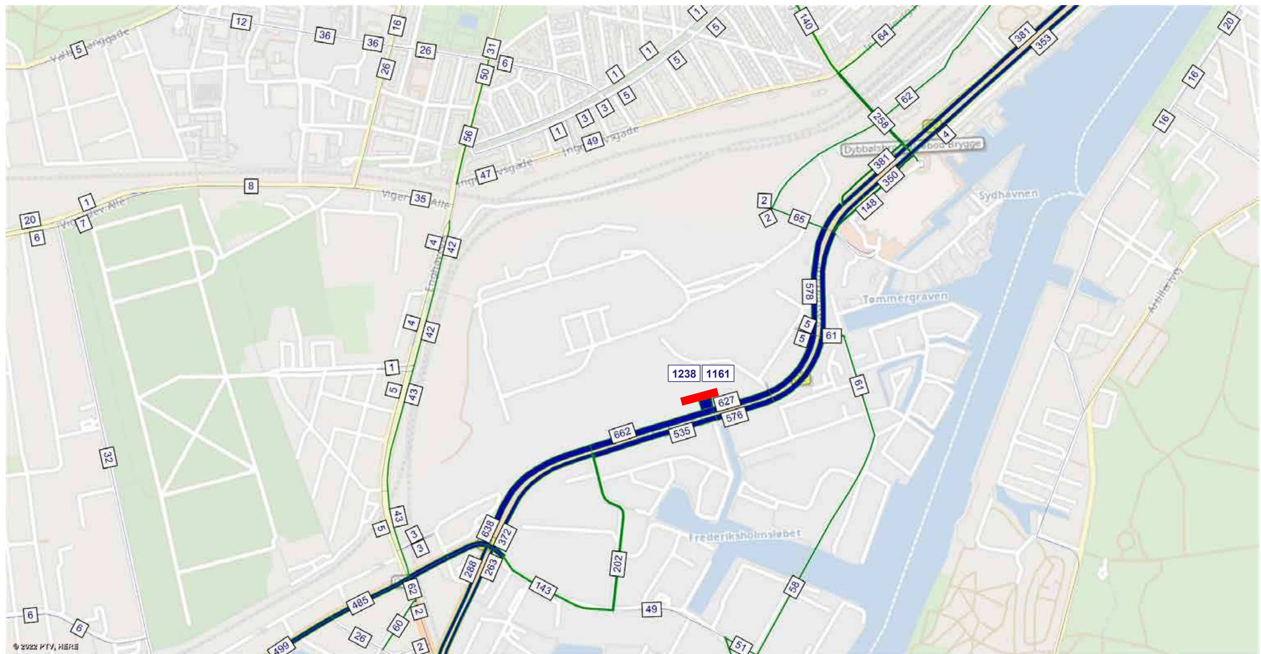
Figur 4-19 Rutebunt for biltrafik ved Jernbanebyens udkørsel ved Belvederekanalen. Det bemærkes, at der ikke er korrigeret for fordeling af trafik mellem Kortløb og Belvederekanalen, jf. afsnit 3.3.1. Rutebundet her indikerer, at trafikken fordeler sig nogenlunde ligeligt mod øst og vest på Vasbygade.
