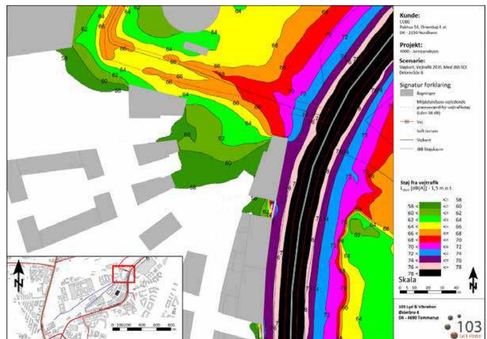
Figur 7-8 Jernbanebyen. Zoom nær Delområde 6. Støjudbredelseskort for vejtrafik vist med flere intervaller. Der ses støj ved facader på op mod 63 dB ( L_{den} ).
