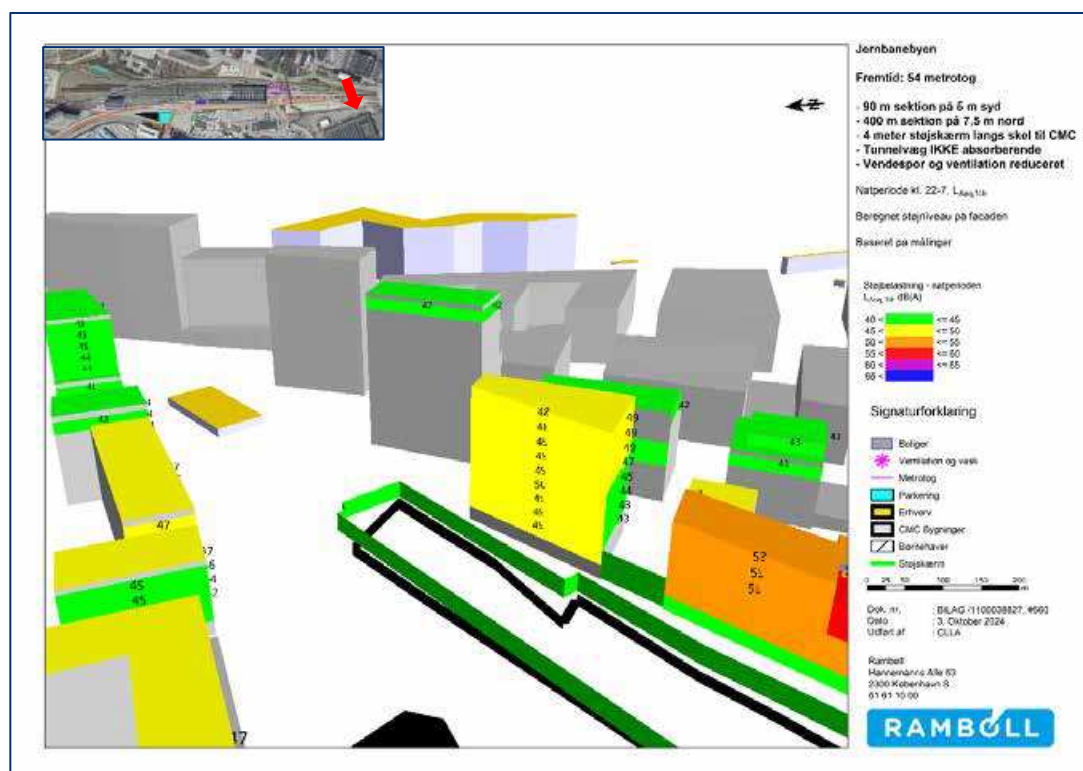
Figur 20-19. Scenarie: Reduceret støj uden overdækning. 3D opstalt af beregnet støjniveau på facaden i natperioden. Grå facader er udsat for støj med niveauer under 40 dB. Opstalten viser bygninger på sydøst siden af CMC set fra CMC området med tunnelrampen til venstre (sammenlign evt. med Figur 20-18).
