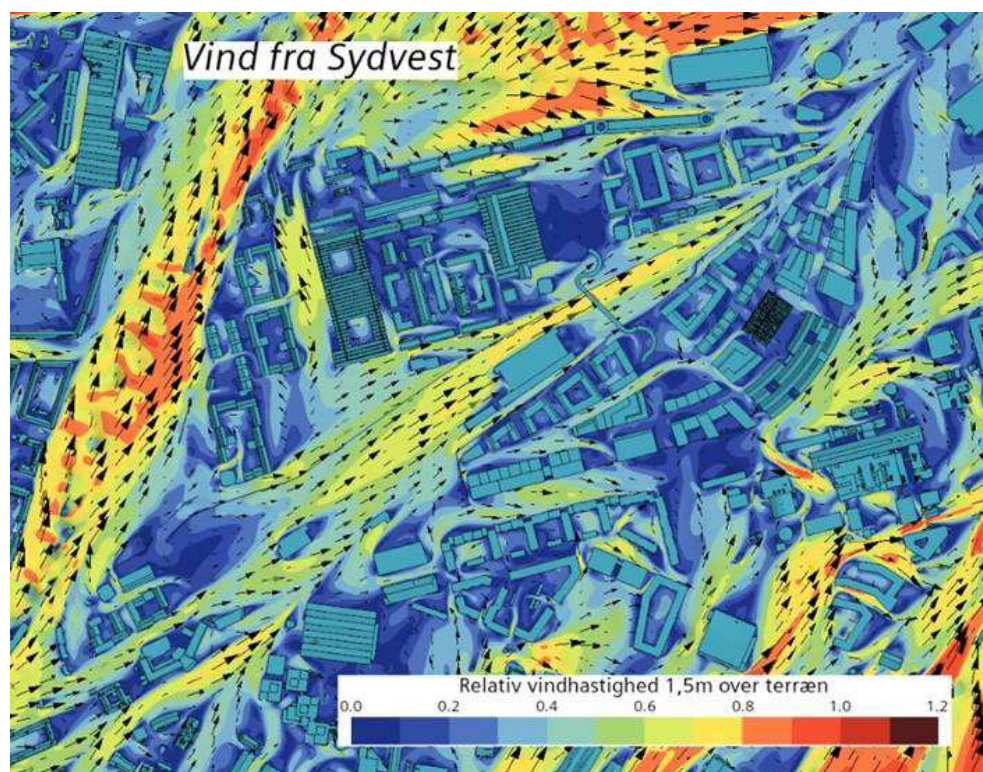
Figur 12-16 Relativ vindhastighed (ift. vinden i 10 meters højde uforstyrret) beregnet 1,5 meter over gadeniveau i Jernbanebyen. Vind fra sydvest. (Figur: COWI).
