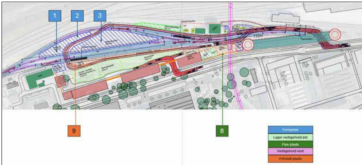
Figur 5: Skitseløsning fra figur 2, hvor dedikerede arealer til fornyelse er markeret.
