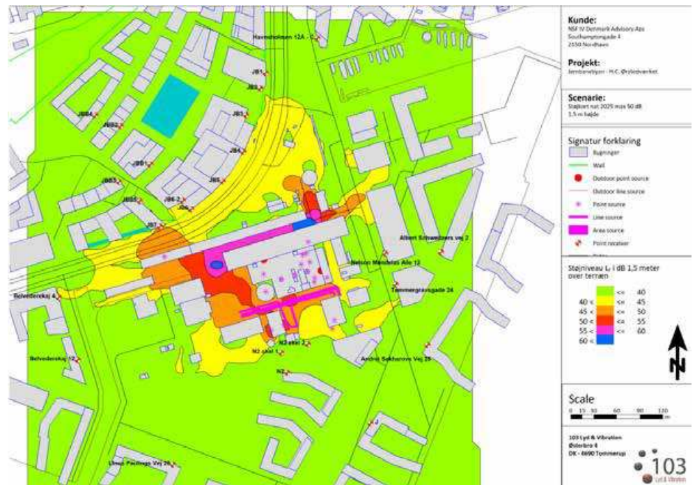
Figur 5-19 H.C. Ørstedværket fremtidigt scenario inkl. støj dæmpning for overholdelse af 50 dB(A) på facader i Jernbanebyen langs Vasbygade. Støjudbredelseskort for natperioden 1,5 meter over terrænet (103).
