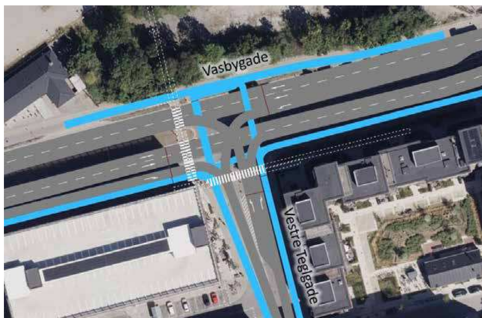
Figur 6-8 Krydset Vasbygade/Vestre Teglade i Basis 2019 og Basis 2035 (Udklip fra VISSIM-modellen). Samtlige resultater for krydset kan ses i Bilag C.8.
