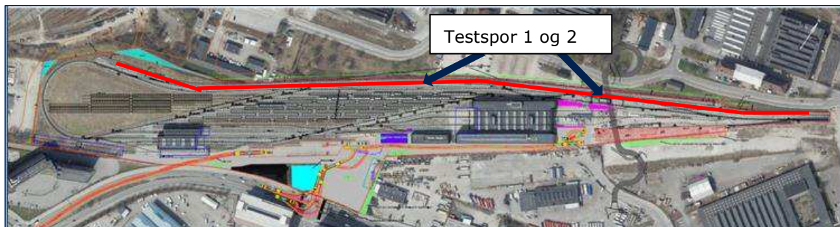
Figur 9-8. Testspor 1 er fuldt funktionsdygtig i dag. Testspor 2 etableres som en del af kapacitetsudvidelse til 54 metrotog. Der køres i gennemsnit 60 km/t på testspor 1 og 2.
