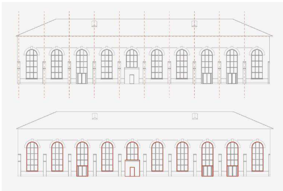
Figur 5-51 Eksisterende sydfacade analyse af rytme (øverst) og åbninger af facade (nederst). Tegning Cobe.
