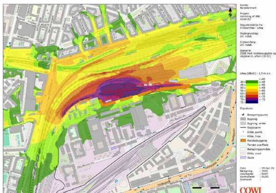
Figur 5-14 CISB. Støjudbredelse aftenperioden.
