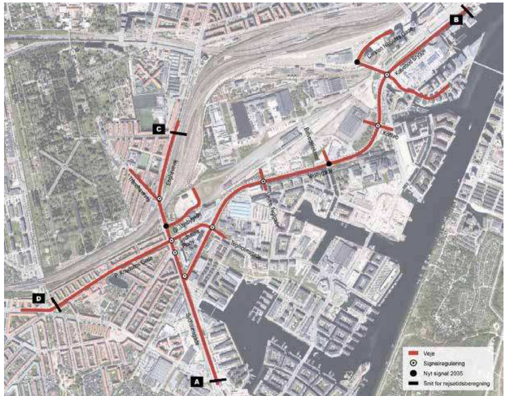
Figur 9-10 Snit i vejnettet, der er anvendt til at beregne rejsetider for motorkøretøjer.
