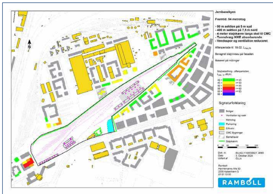
Figur 20-16. Scenarie: reduceret støj uden overdækning. Beregnet støjniveau på facaden i afterperioden.
