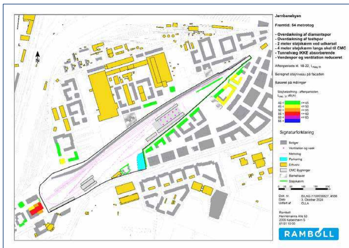
Figur 20-10. Scenarie: Reduceret støj med overdækning. Beregnet støjniveau på facaden i aftenperioden.
