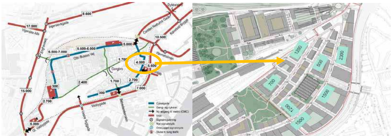
Figur 3-10 Fordeling af cykeltrafik fra det forenklede stinet trafikberegningerne til helhedsplanens vej- og stinet
