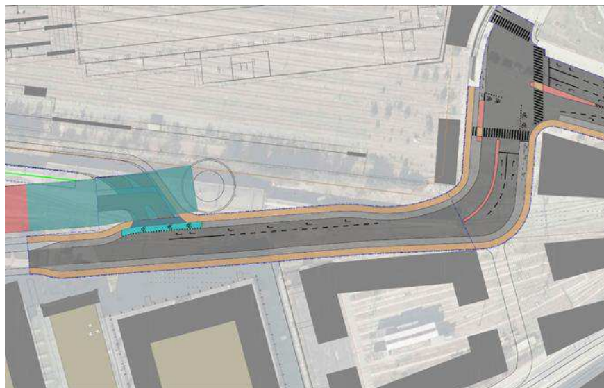
Figur 4-20: Skitse af adgangsforhold til delområde XII (randbebyggelse og p-hus) og delområde IXa (CISB).
