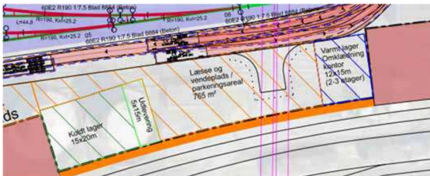
Figur 11: Flex pladsens disponering med koldt lager og udendørs udleveringsplads, læsseplads og midlertidig parkering samt varmt lager, kontorer, velfærdsfaciliteter m.v. i 3 etagers højde.
