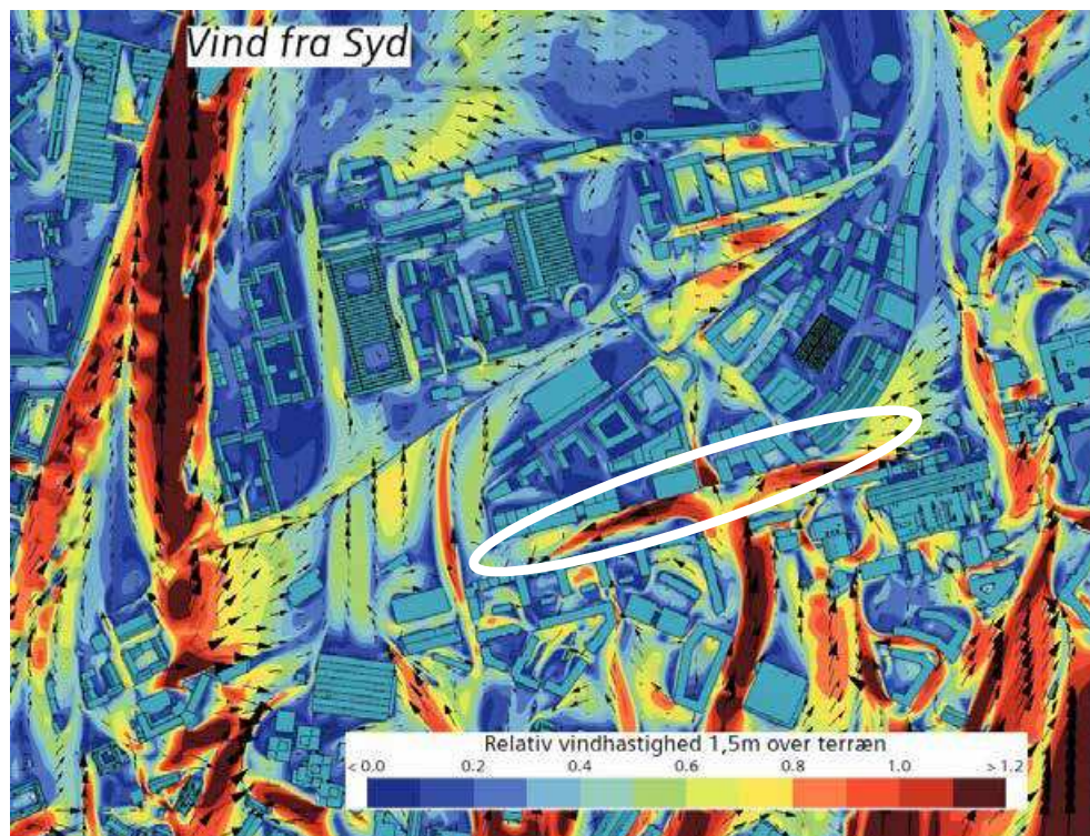
Figur 12-10 Relativ vindhastighed (ift. vinden i 10 meters højde uforstyrret) beregnet 1,5 meter over gadeniveau i Jernbanebyen. Vind fra syd. Vasbygade vist med hvid markering. Se Bilag D – Vindmiljøanalyse – Jernbanebyen. (Figur: COWI).
