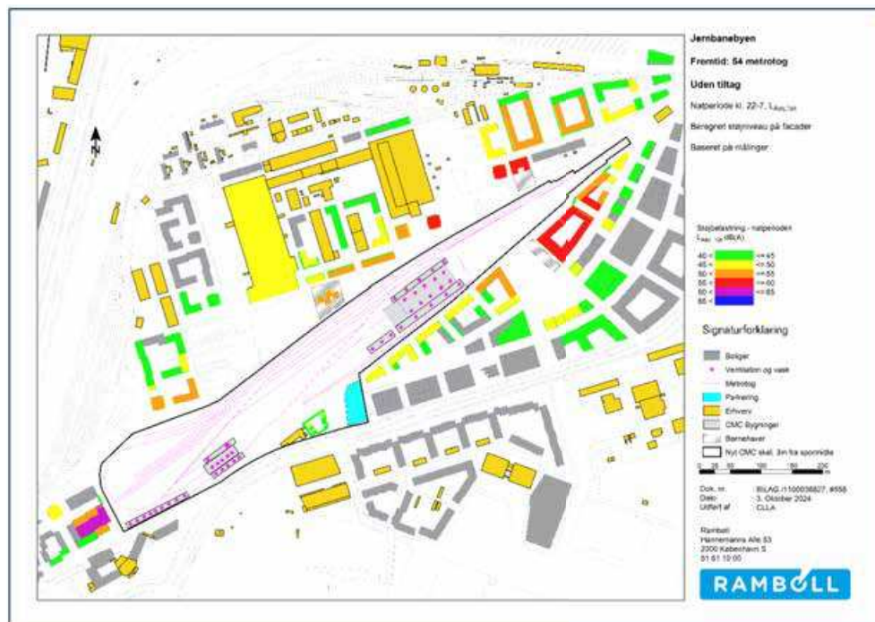
Figur 5-8 CMC. Facadestøjskort natperioden uden støjdæmpende foranstaltninger ved maksimal kapacitetsudbygning (Rambøll).
