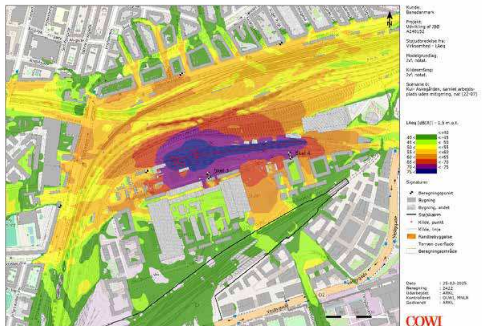
Figur 5 Støjbreddelseskort for fremtidig samlet arbejdsbase i Askegården, uden støjmitigerende tiltag.
