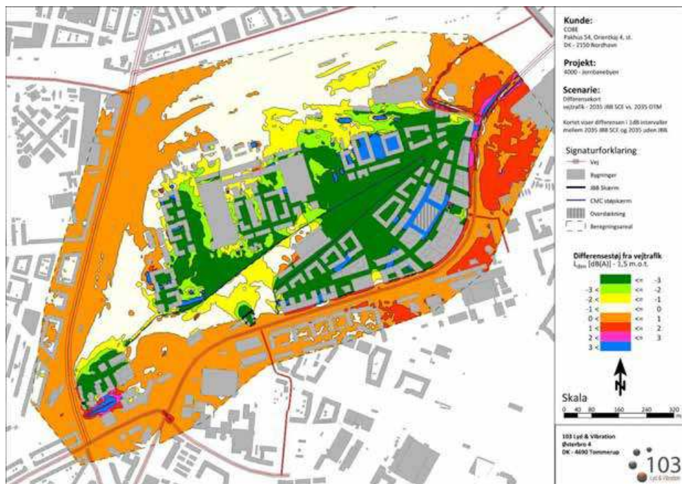
Figur 10-14 Støjudbredelseskort for vejtrafikstøj – differenskort for 2035. (Kort: 103 Rådgivende Ingeniører).
