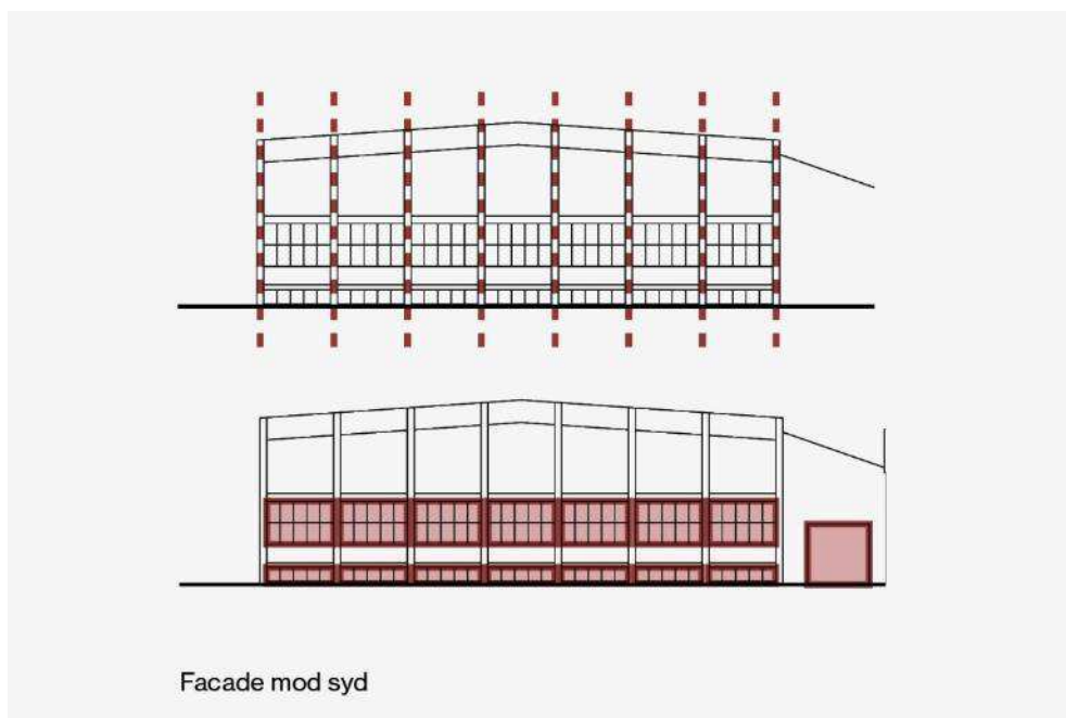
Figur 5-109 Eftersynshallen sydfacade. Her vises rytmen i facadens søjler øverst og nederst ses de vertikale vinduesbånd. Tegning Cobe.
