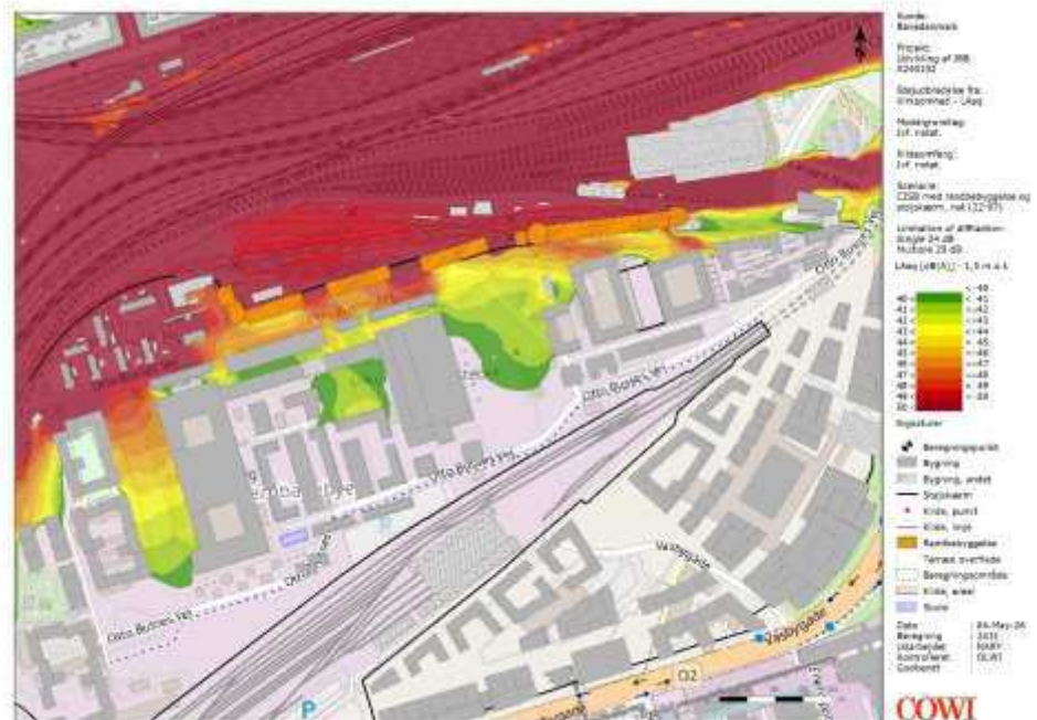
Figur 10 Støjkonturkort for fremtidige aktiviteter på CISB i natperioden med 1 dB intervaller. Grænse for maksimal dæmpning hævet til henholdsvis 24 dB og 29 dB.
