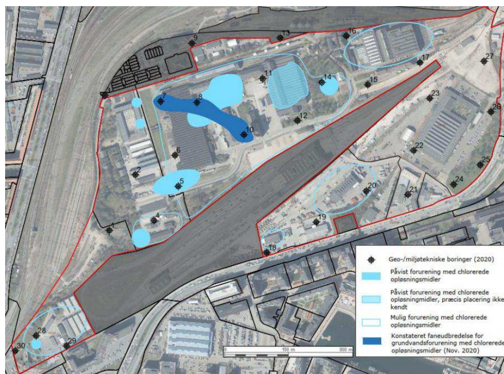
Figur 17-4 Områder med påvist og potentiel forurening med klorerede opløsningsmidler i de kvartære lag (fra DMR resumerapport af 23.02.2021).
