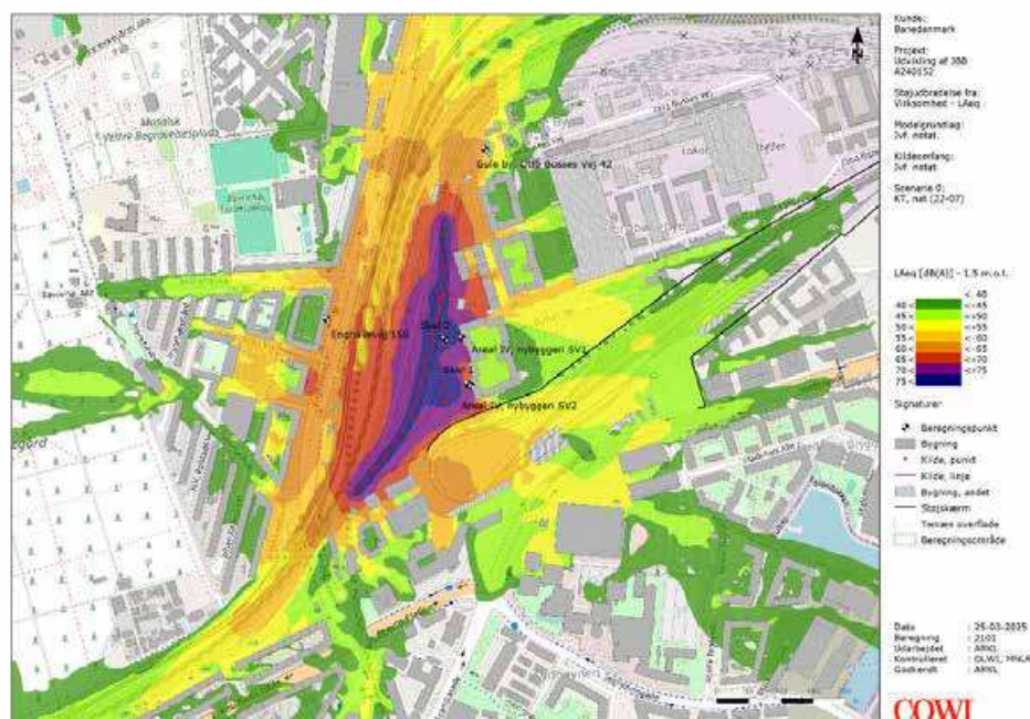
Figur 2 Støjuddredelseskort for KT nuværende forhold.
