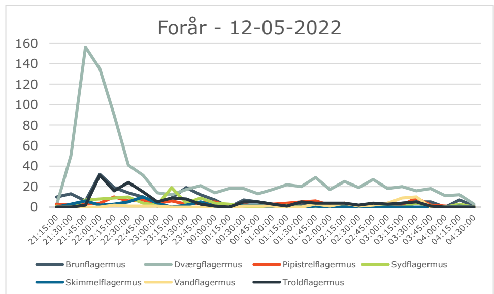
Figur 6-3 Den tidslige fordeling af de enkelte arters aktivitet for boks Vk1.1 og Vk1.3.
