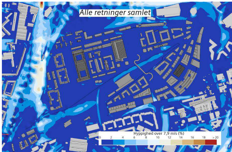
Figur 12-9 Hyppighed for overskridelse af 7,9 m/s , som skal være mindre end 4 % for aktivitet gang/slentren. Alle vindretninger, årsklima. Bilag D – Vindmiljøanalyse – Jernbanebyen. (Figur: COWI).
