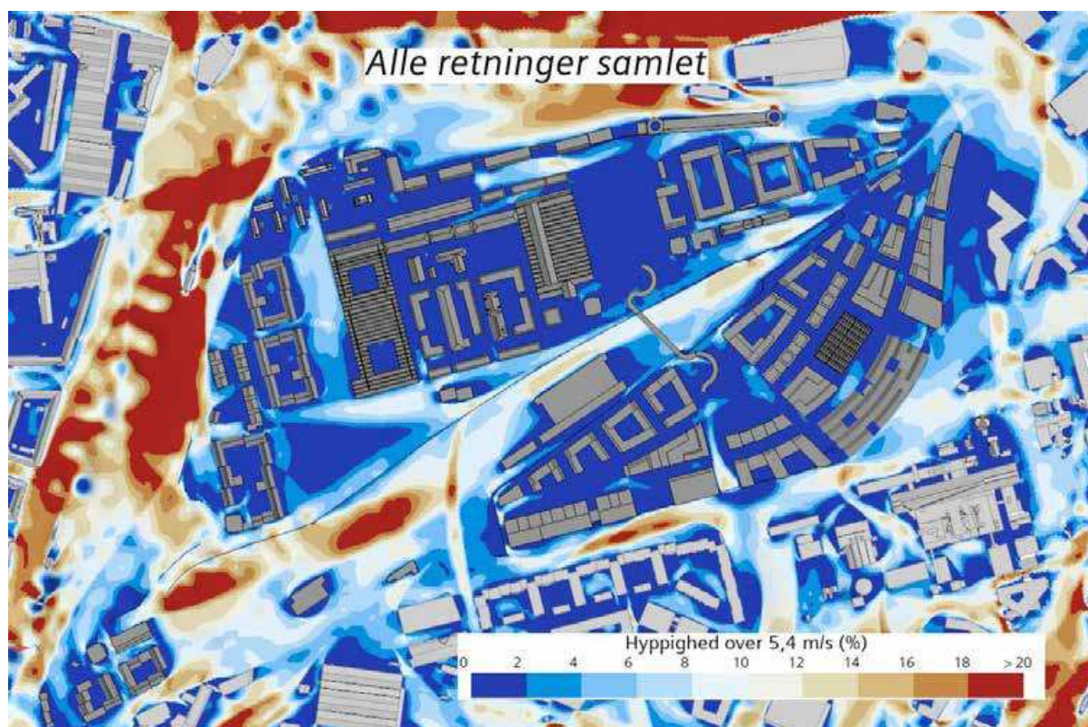
Figur 4.5 Hyppighed for overskridelse af 5,4 m/s beregnet 1,5 m over gadeniveau i Jernbanebyen. Alle vindretninger, årsklima. Beregnet ud fra Weibull-parametrene og hyppighederne i Tabel 3.1. Aktivitet: siddende og stående.
