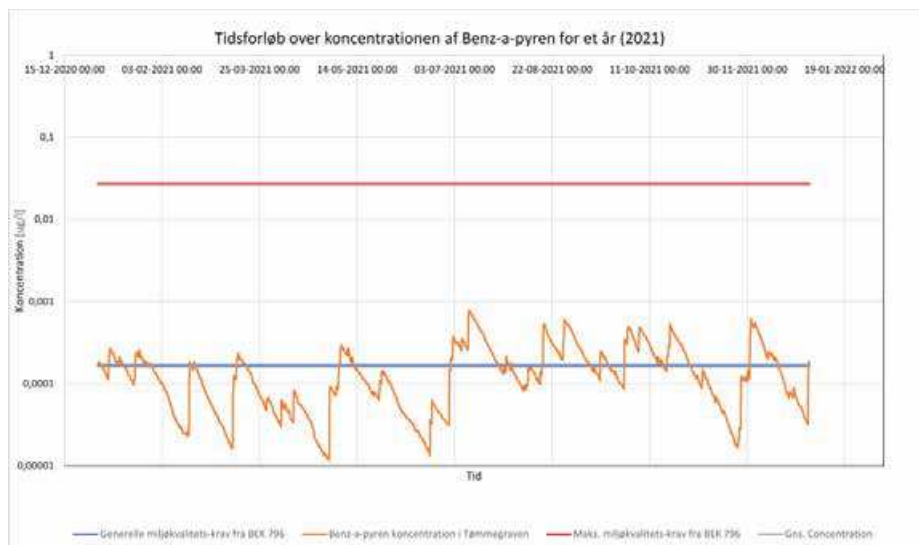
Figur 4-5: Benz(a)pyren koncentration i hele Tømmergraven over tid for år 2021
