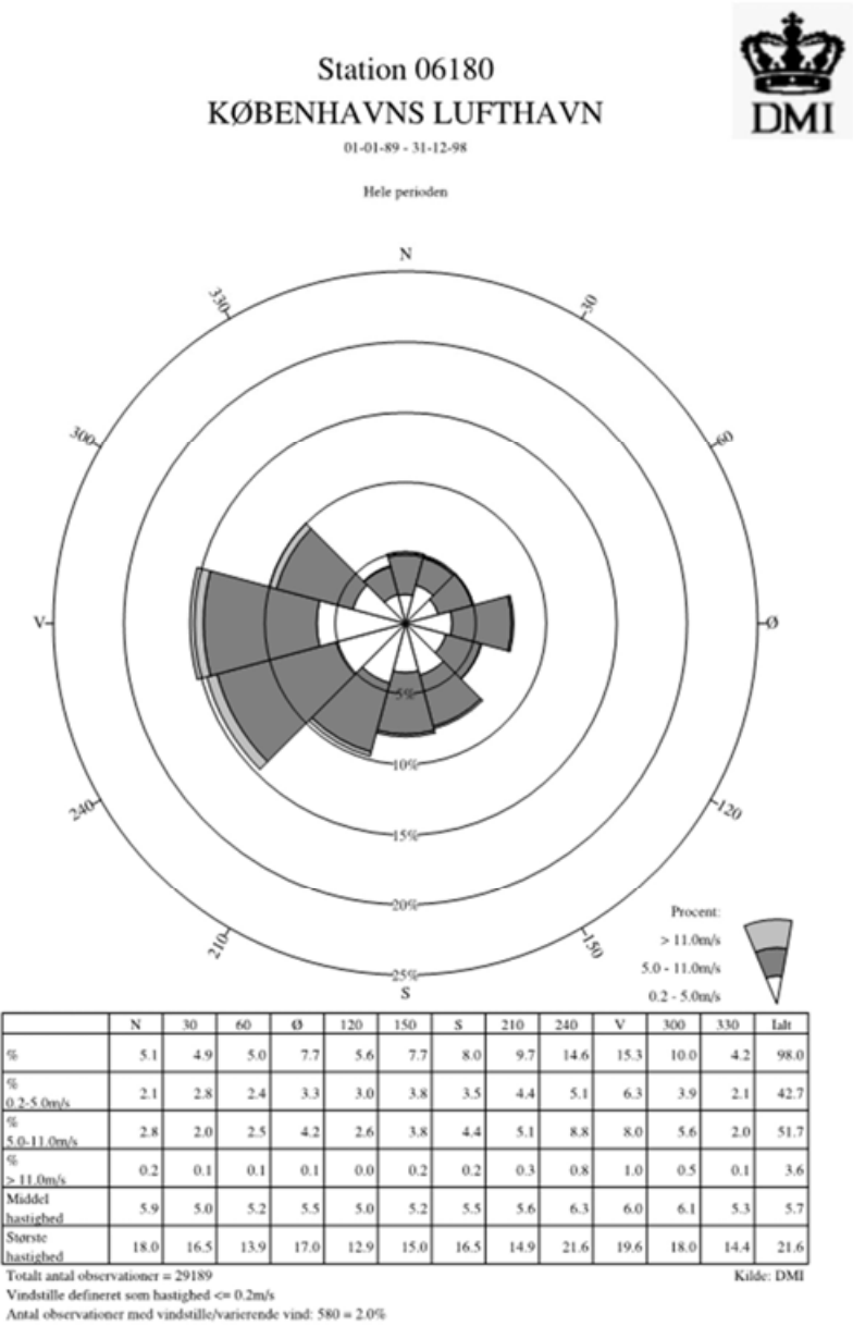
Figur 3.6 Vindrose, hele året. Fra DMI.
