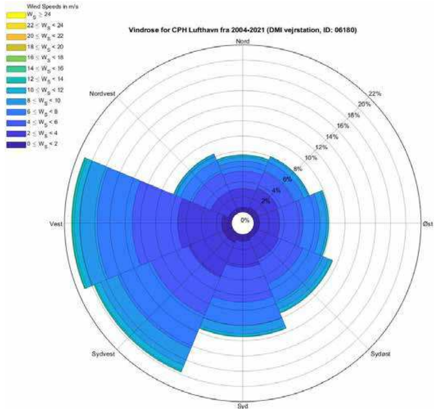
Figur 3.5 Vindrose, hele året. DMI Frie Data 2004-2021. Retningsopløsning for komfortanalysen. Højde over terræn 5 m.
