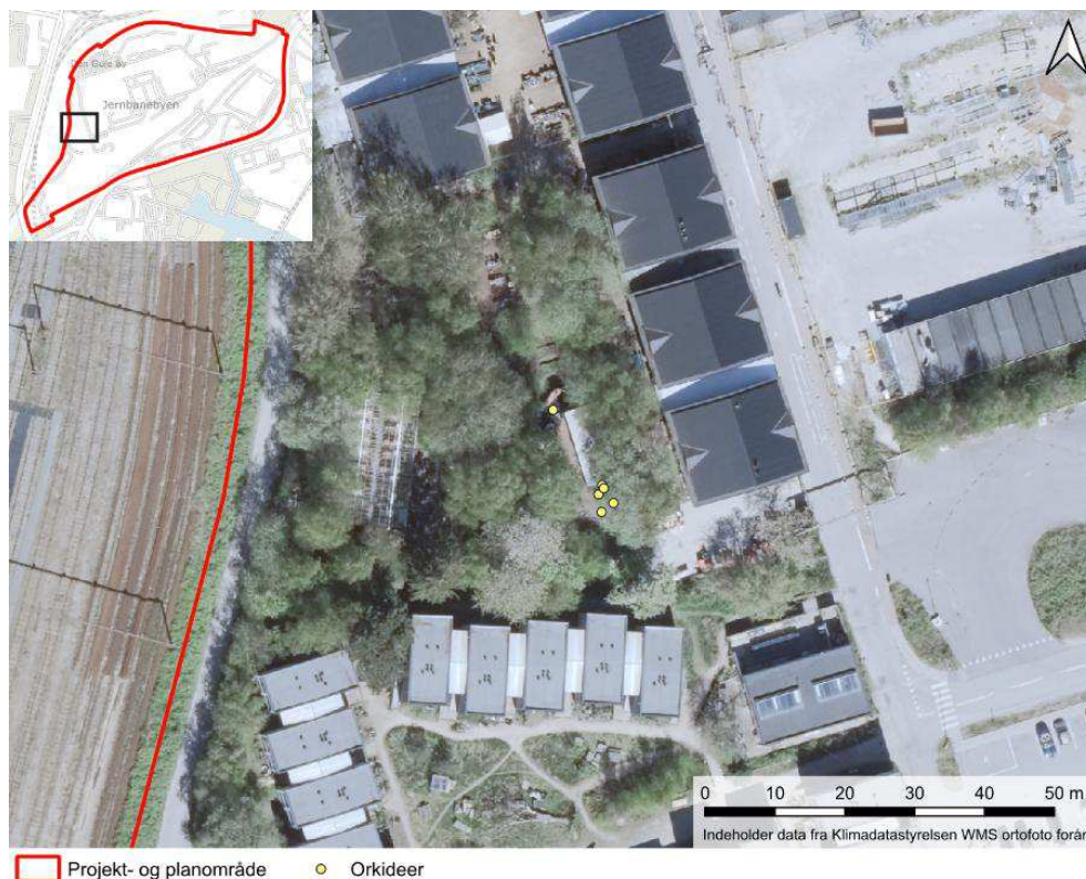
Figur 14-4 Lokationerne for de syv registreringer (gule prikker) af skovhullæbe. (Figur: COWI).
