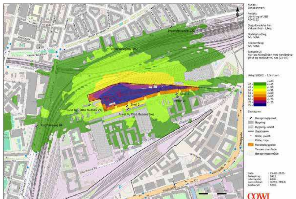
Figur 6 Støjdbredelseskort for fremtidig samlet arbejdsbase i Kulgården/Askegården, med randbebyggelse langs JBB og støjskærme mod nord og vest.
