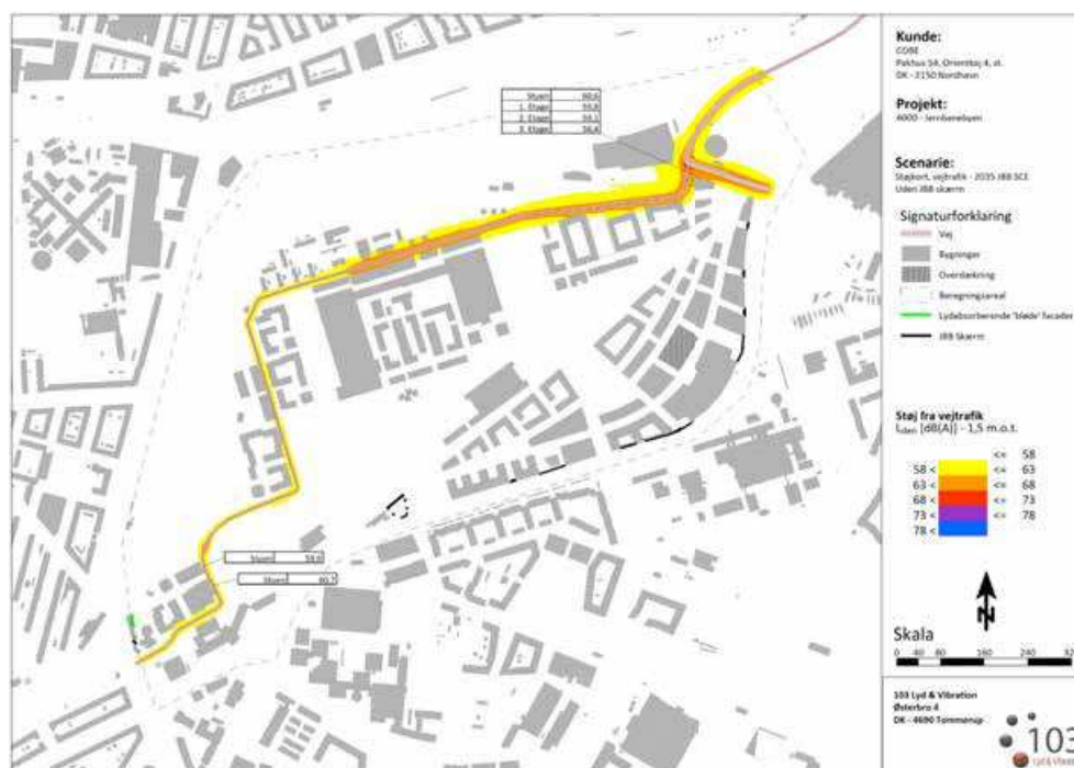
Figur 5-2 Støjudbredelseskort vejtrafikstøj 1,5 meter over terræn for trafikstøj fra Otto Busses Vej og Carsten Niebuhrs Gade i fremtidigt scenario med udbygning af Jernbanebyen år 2035 (103).
