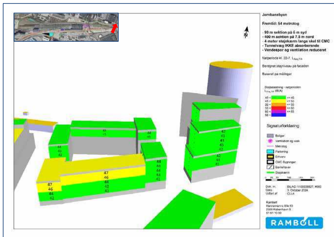
Figur 20-21. Scenarie: Reduceret støj uden overdækning. 3D opstalt af beregnet støjniveau på facaden i natperioden. Grå facader er udsat for støj med niveauer under 40 dB. Bygninger nord for tunnelrampen.
