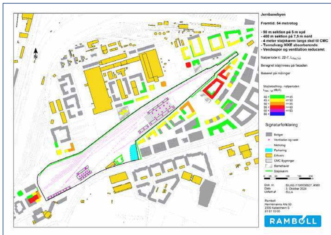
Figur 20-18. Scenarie: Reduceret støj uden overdækning. Beregnet støjniveau på facaden i natperioden.
