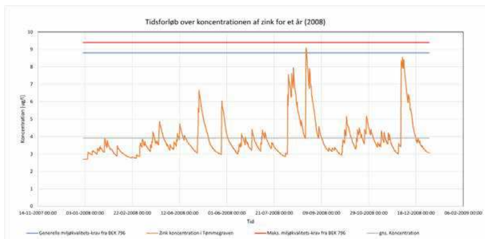
Figur 4-6: Zink koncentration i hele Tømmergraven over tid for år 2008
