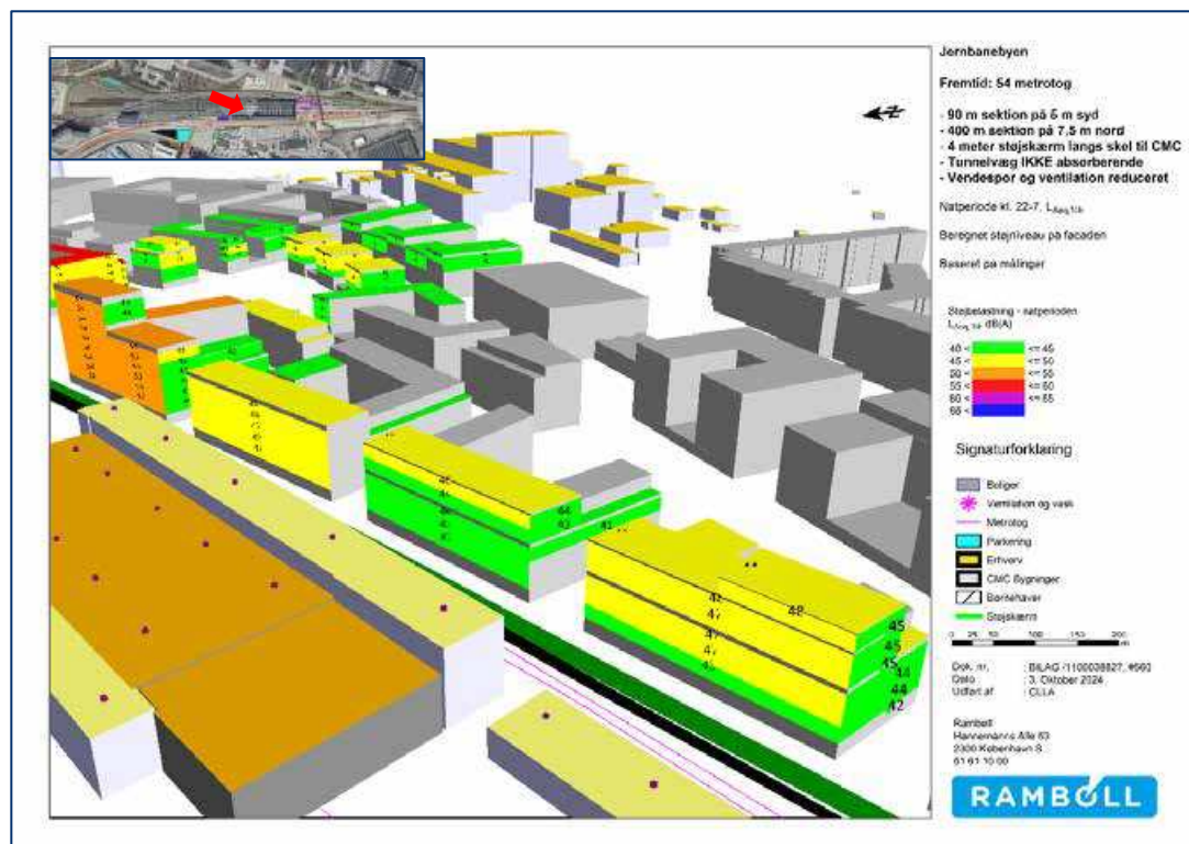
Figur 20-28. Scenarie: Reduceret støj uden overdækning. 3D opstalt af beregnet støjniveau på facaden i natperioden. Bygninger på sydøst siden ud for CMC værkstedsbygning.
