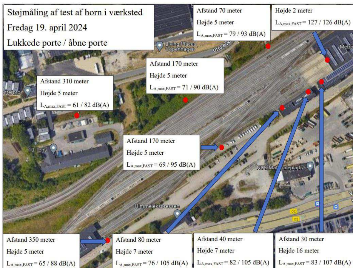
Figur 23-1. Resultat af støjmåling af test af horn i værksted med lukkede og åbne porte. Som eksempel " L_{Amax,FAST} = 69 / 95 dB(A)" betyder L_{Amax,FAST} = 69 dB(A) med lukkede porte og L_{Amax,FAST} = 95 dB(A) med åbne porte. Selv med lukkede porte så er der målt L_{Amax,FAST} \geq 55 dB(A) for samtlige målepunkter.
