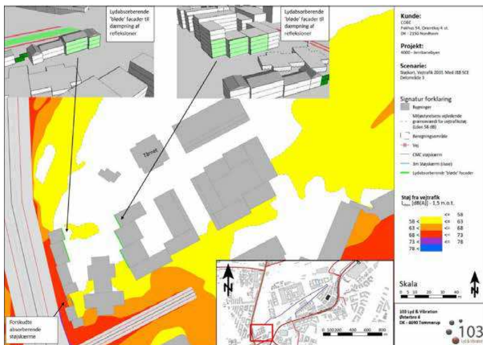
Figur 6-4 Delområde 3. Støjudbredelseskort vejtrafikstøj 1,5 meter over terræn for fremtidigt scenario med støjreducerende tiltag (103)
