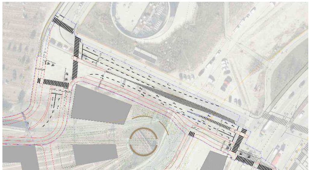
Figur 3-3 Foreslået udformning for det signalregulerede kryds ved Otto Busse vej/ Carsten Niebuhrs Gade. Krydsudformningen anvendes i Scenario 2035.
