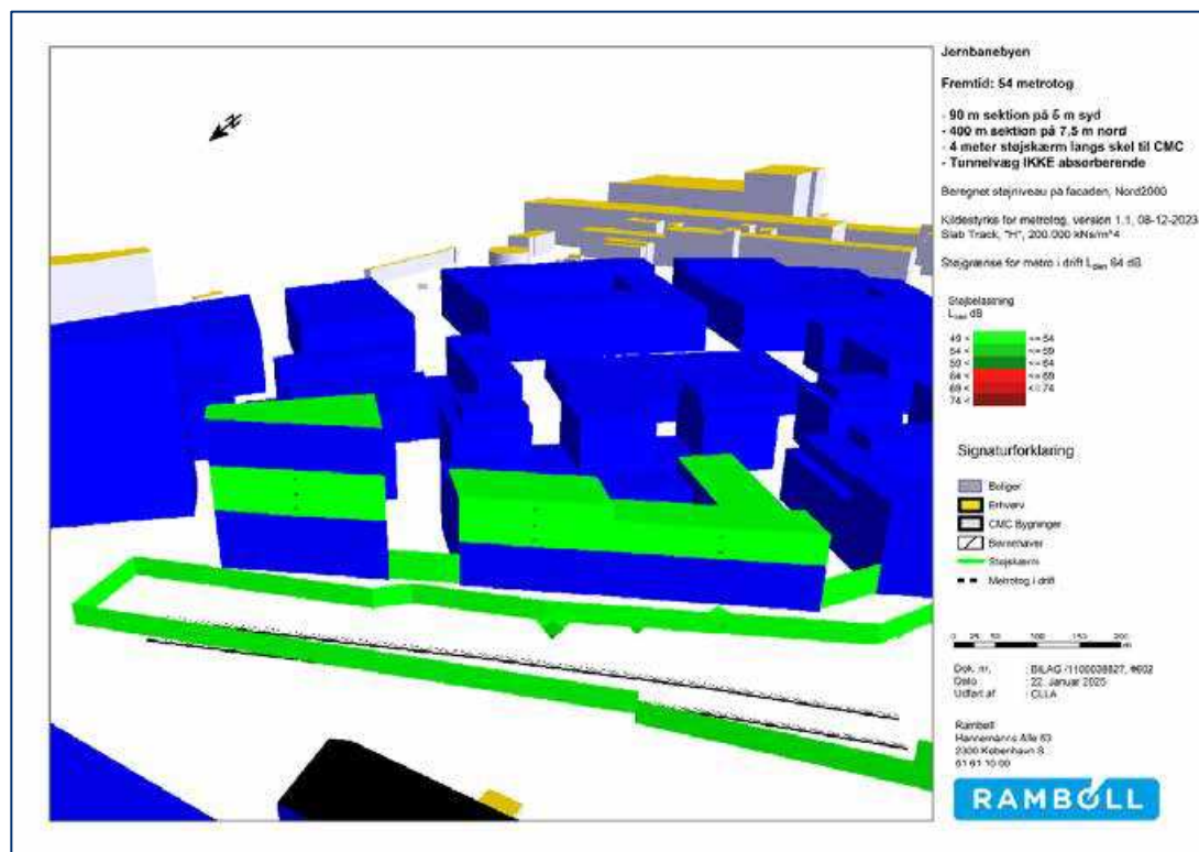
Figur 21-2. Støj i driftsfasen for metrotog som kører med 40 km/t ned mod tunnelåbning og 40 km/t op fra tunnelåbning. Støjgrænse for metro i drift er L_{den} 64 dB for boliger.
