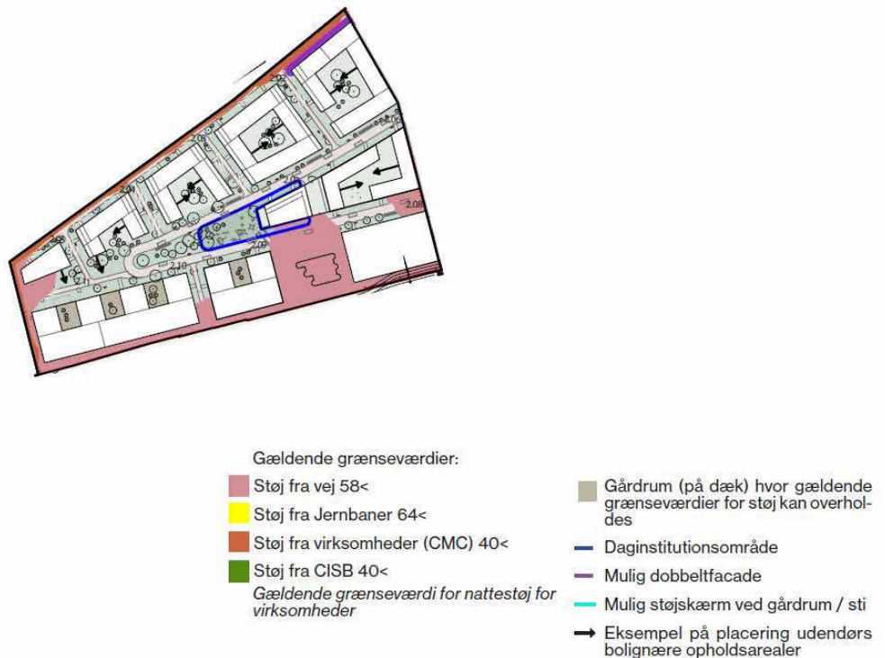
Figur 7-3 Jernbanebyen Delområde 2. Oversigtskort over udbredelse af støj fra veje, jernbaner, CMC og andre virksomheder. Der er kun vist støjudbredelse for områder, hvor støjniveauet er beregnet over Miljøstyrelsens vejledende grænseværdier for støj på udendørs opholdsarealer. Pile angiver adgang til udendørs opholdsarealer.
