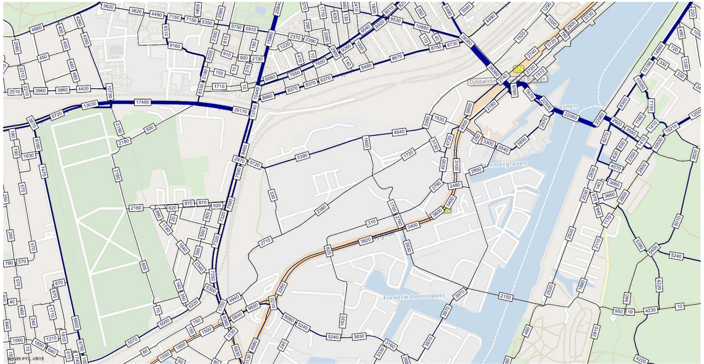
Figur 4-1 Beregnet cykeltrafik (hverdagsdøgn) igennem Jernbanebyen og på vejnettet omkring, beregnet for et scenarieår 2035 efter Jernbanebyens udbygning.
