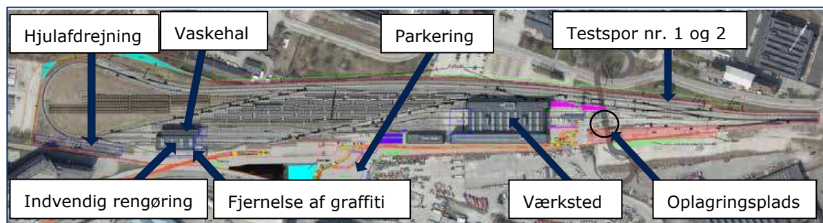
Figur 9-1. Placering af bygninger, spor og områder på CMC Vasbygade ved fremtidig indretning til fuld kapacitet.
