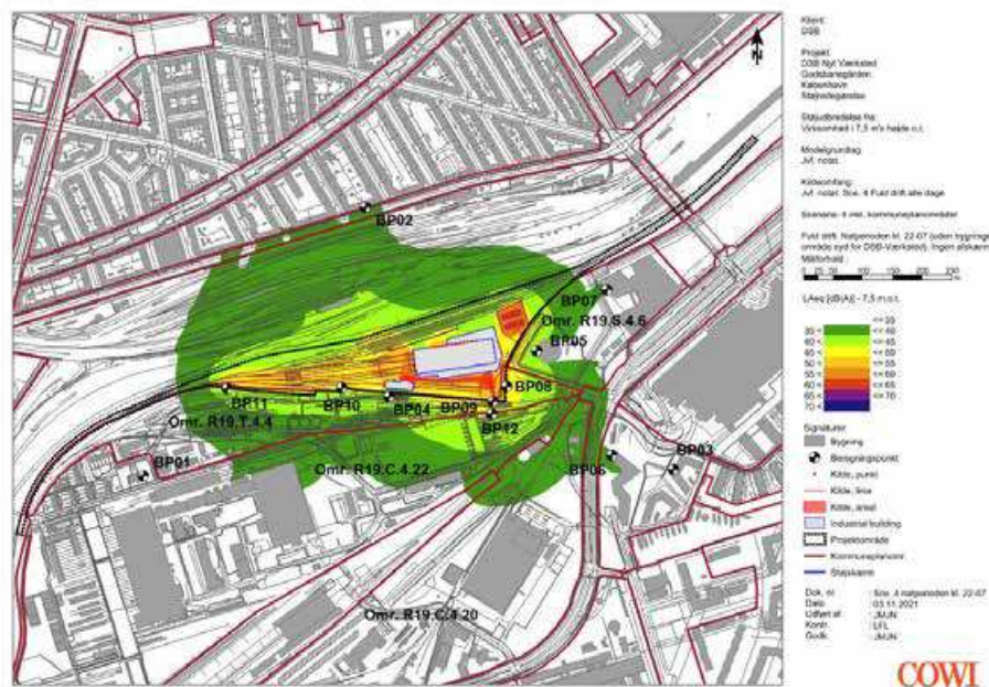
Figur 5-17 DSB Nyt værksted. Støjudbredelseskort for projektforslaget (år 2024) af nyt værksted i natperioden, 1,5 meter over terræn svarende til friarealer og stueetage (COWI).
