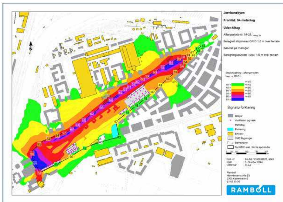
Figur 5-5 CMC. Støjdbredelseskort aftenperioden uden støj dæmpende foranstaltninger ved maksimal kapacitets udbygning (Rambøll).
