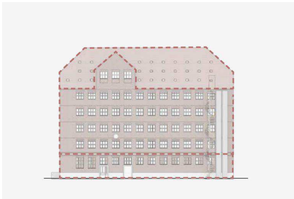
Figur 5-83 Facaden tredeling mellem base, krop og tag. Tegning Cobe.
