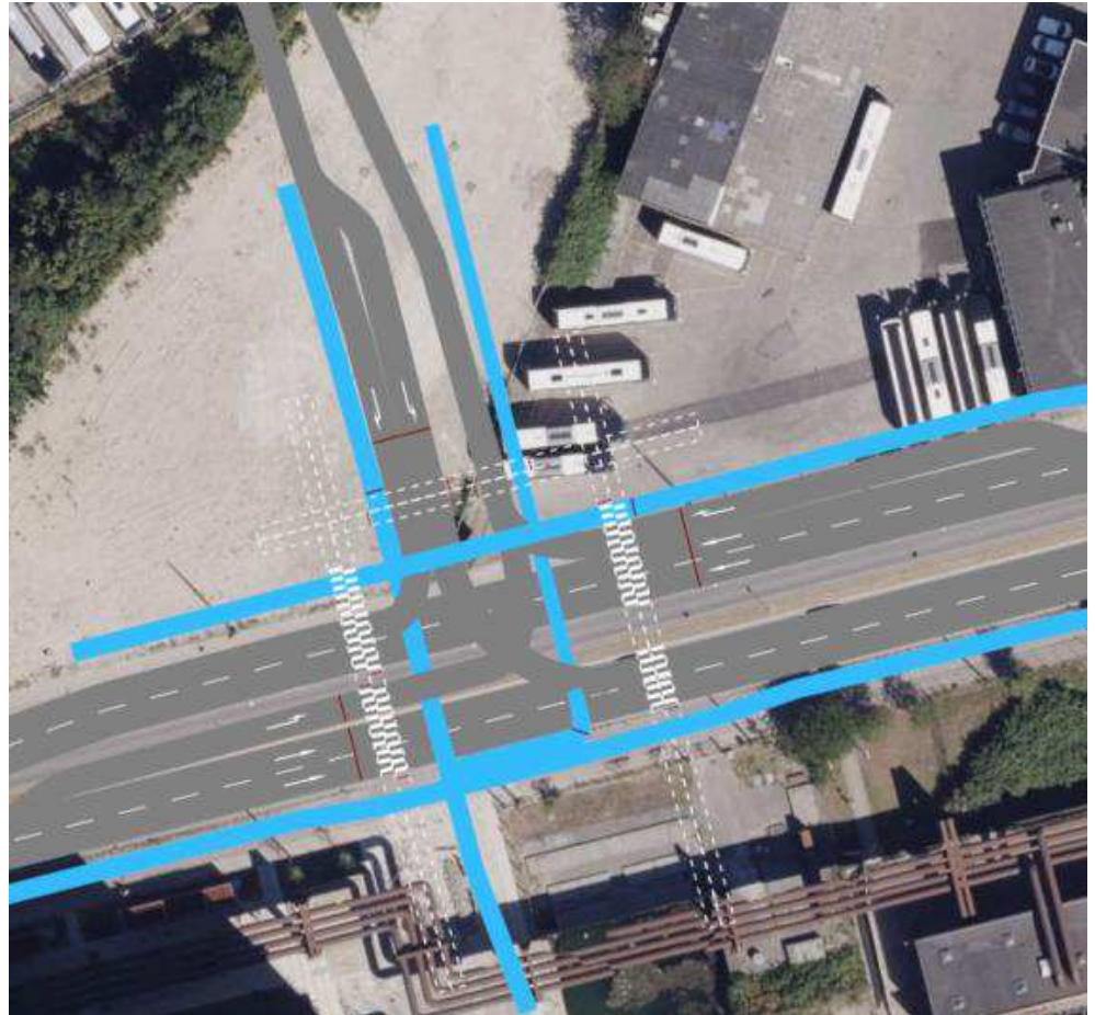
Figur 6-11 Krydset Belvederekanalen /Vasbygade (Udklip fra VISSIM-modellen Scenario 2035). Samtlige resultater for krydset kan ses i Bilag C.9
