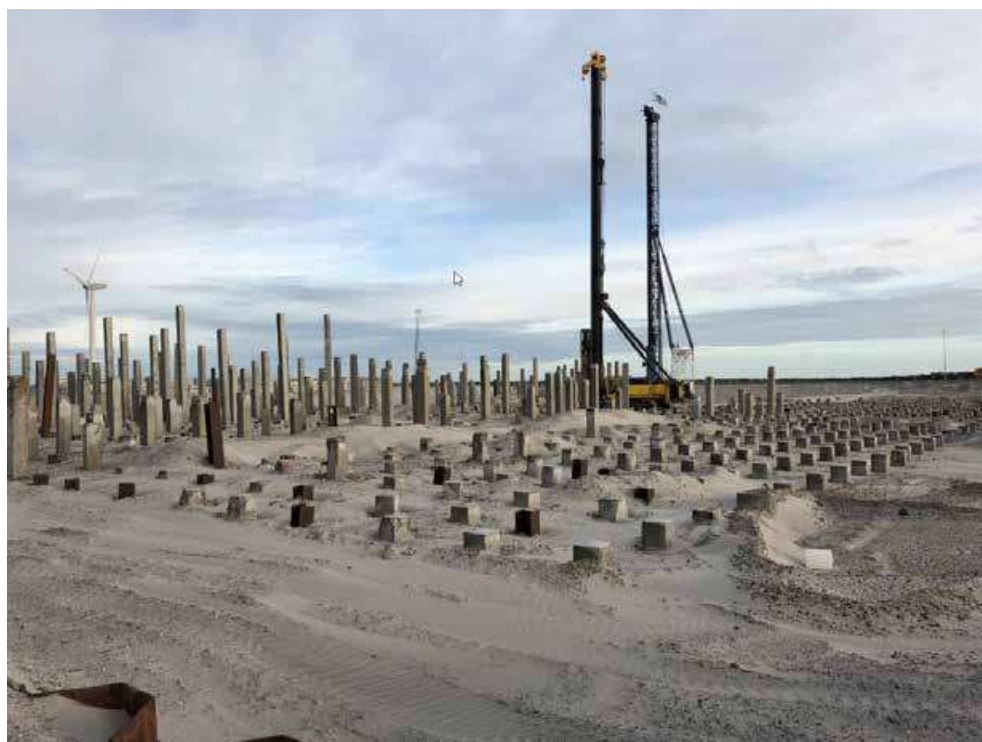
Figur 4-28 Eksempel på anlæg af pælefundering. (Foto: COWI).
