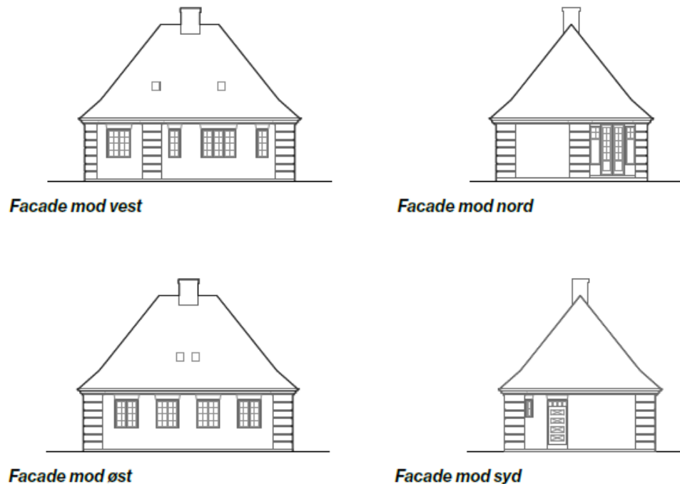
Figur 5-7 Portbygningens eksisterende facader. Illustration Cobe.
