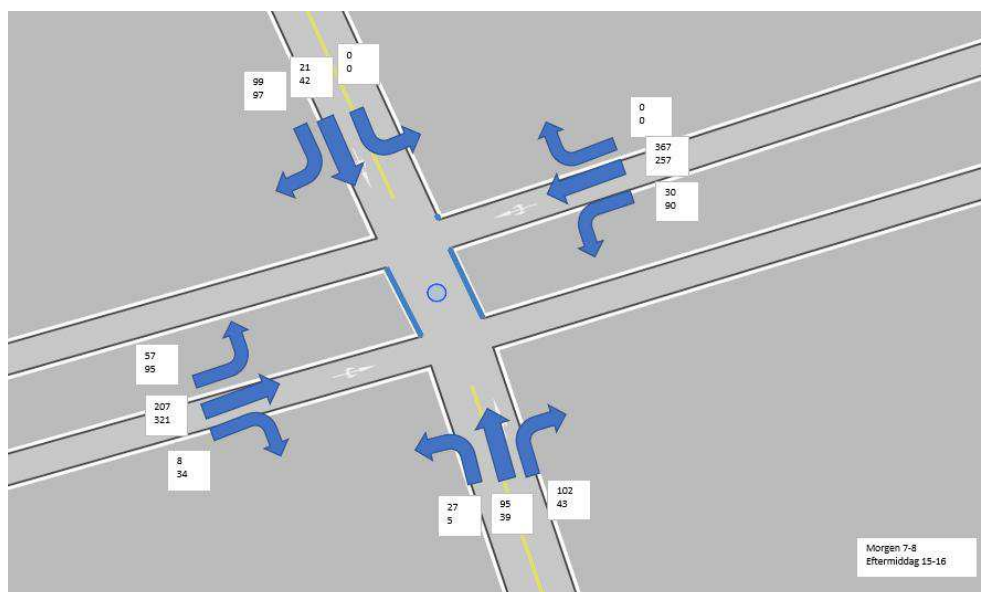
Figur 5-17 Beregnet cykeltrafik i OTM for spidstimerne i krydset Vasbygade/ Belvederekanalen. (Det bemærkes, at retningsfordeling for cykeltrafik i trafikmodeller er behæftet med en stor usikkerhed, da der er mange parametre, som trafikmodellerne har vanskeligt ved at tage højde for, der påvirker cyklisterne rutevalg).
