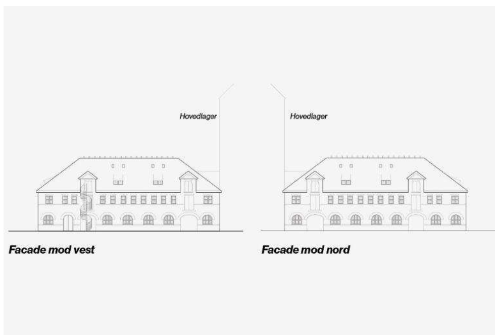
Figur 5-79 Facadetegninger – eksisterende forhold. Tegning Cobe.
