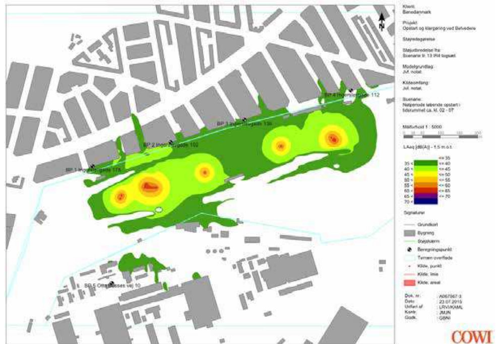
Figur 5-16 Opstart af ellokomotiver ved Belvedere. Støjudbredelseskort (COWI).
