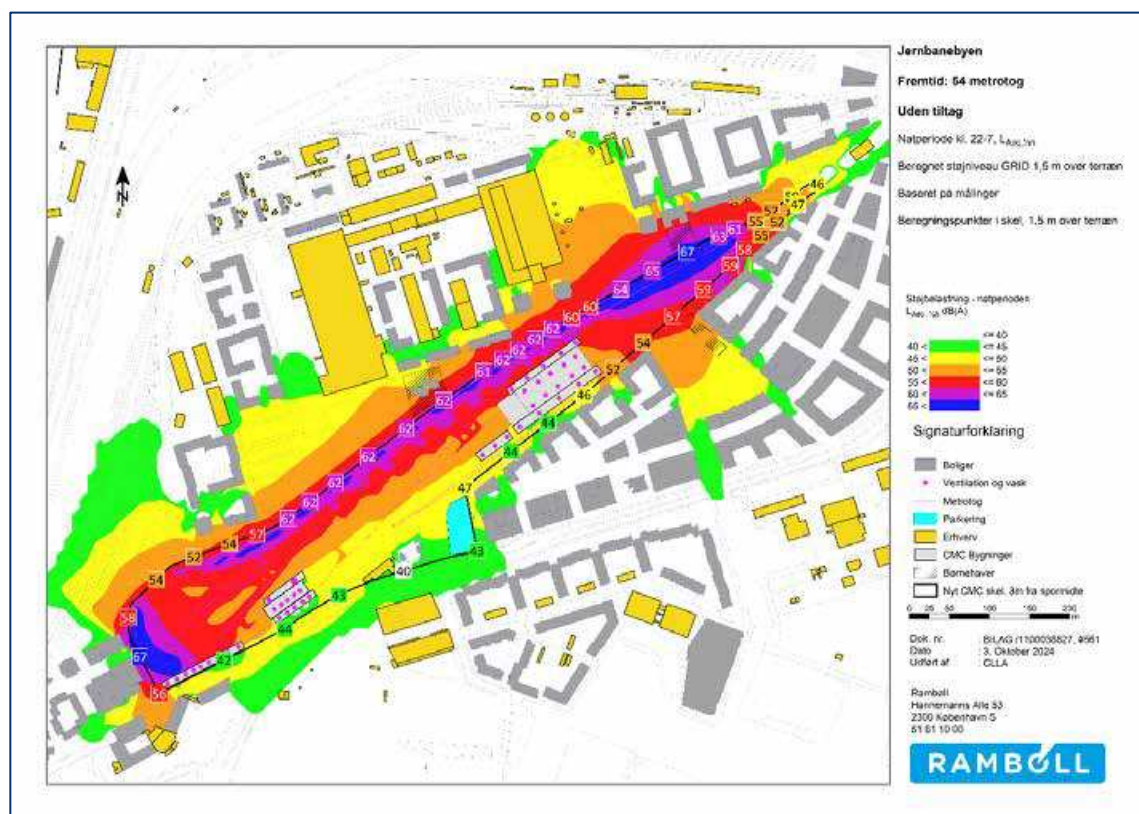
Figur 20-5. Scenarie: Uden støj dæmpende tiltag. Beregnet støjniveau i skel og støjkontour 1,5 meter over terræn i natperioden.
