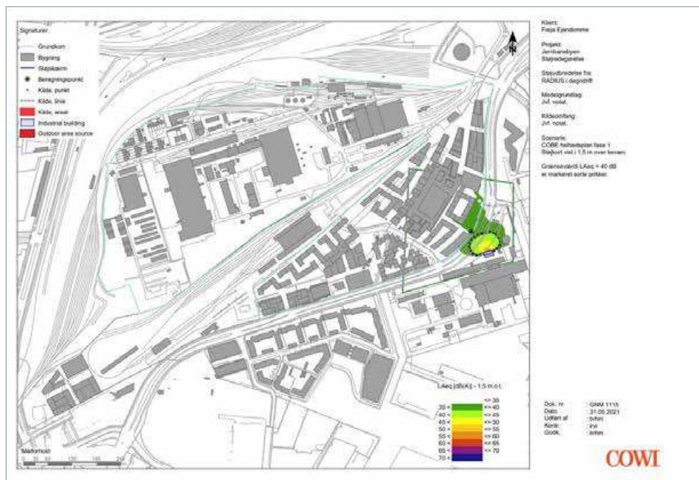
Figur 5-20 Radius. Støjdbredelseskort 1,5 meter over terræn (COWI).
