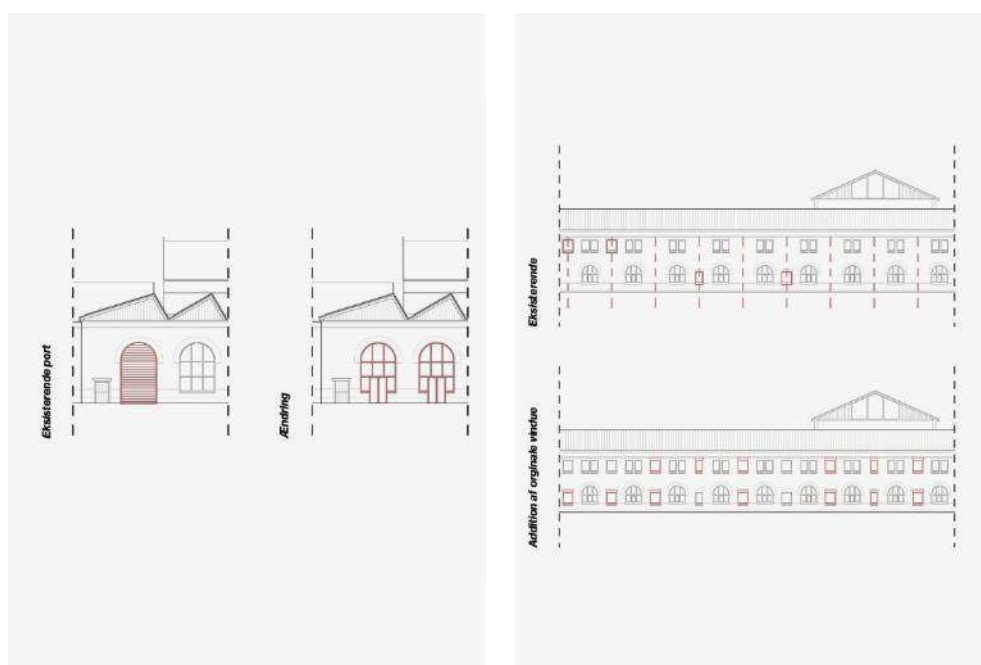
Figur 5-91 Forslag til ændringer i facader på Lokomotivværkstedet. Tegning Cobe.
