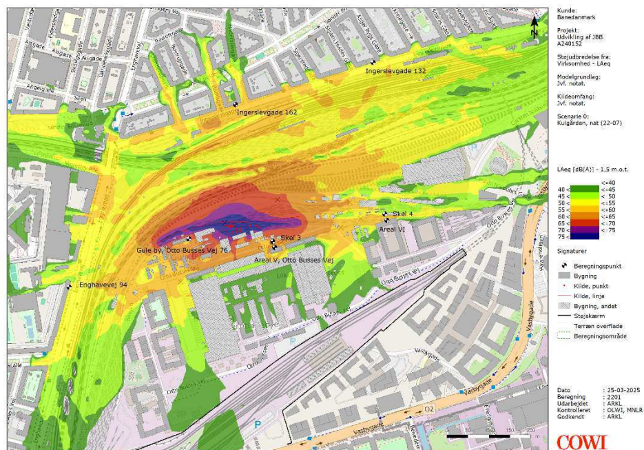
Figur 7 Støjudbredelseskort for Kulgården - nuværende forhold.
