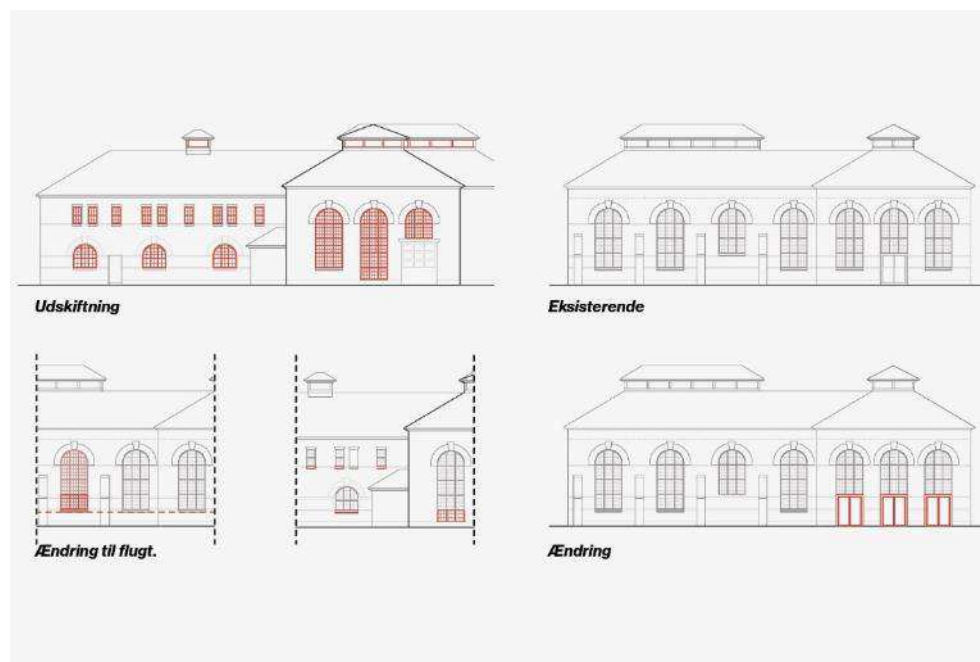
Figur 5-68 Forslag til ændringer i Kraftcentralen/baderums facader i form af udskiftning af vinduer og døre. Tegning Cobe.
