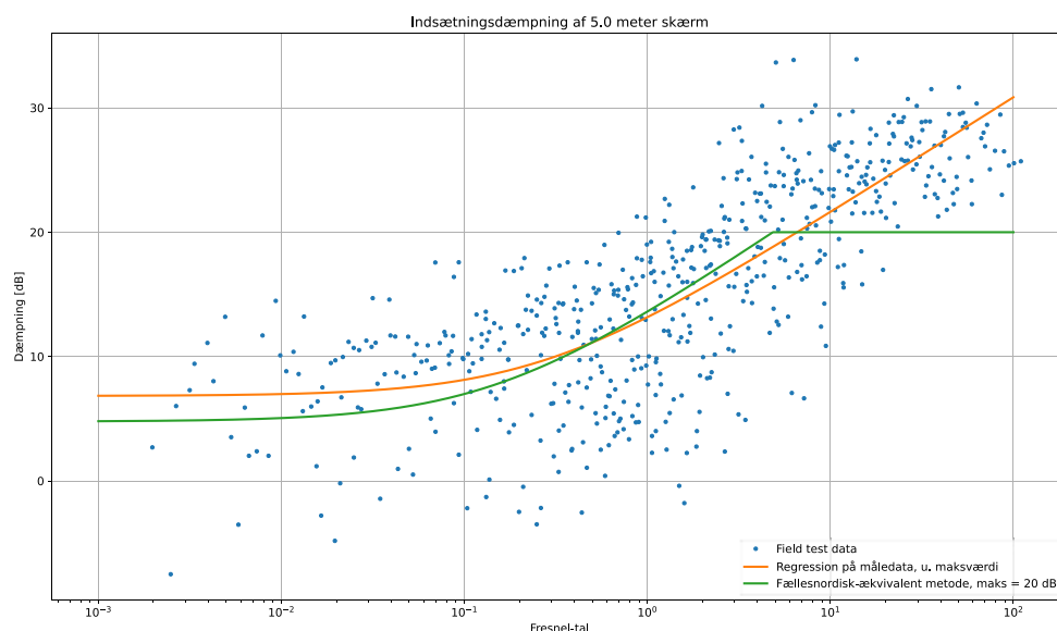
Figur 9 Indsætningsdæmpning for støjskærm som funktion af Fresneltal. Måledata er markeret med blå prikker. Kurvetilpasning af måledata er markeret med orange kurve, og den officielle danske beregningsmodel med grøn farve.
