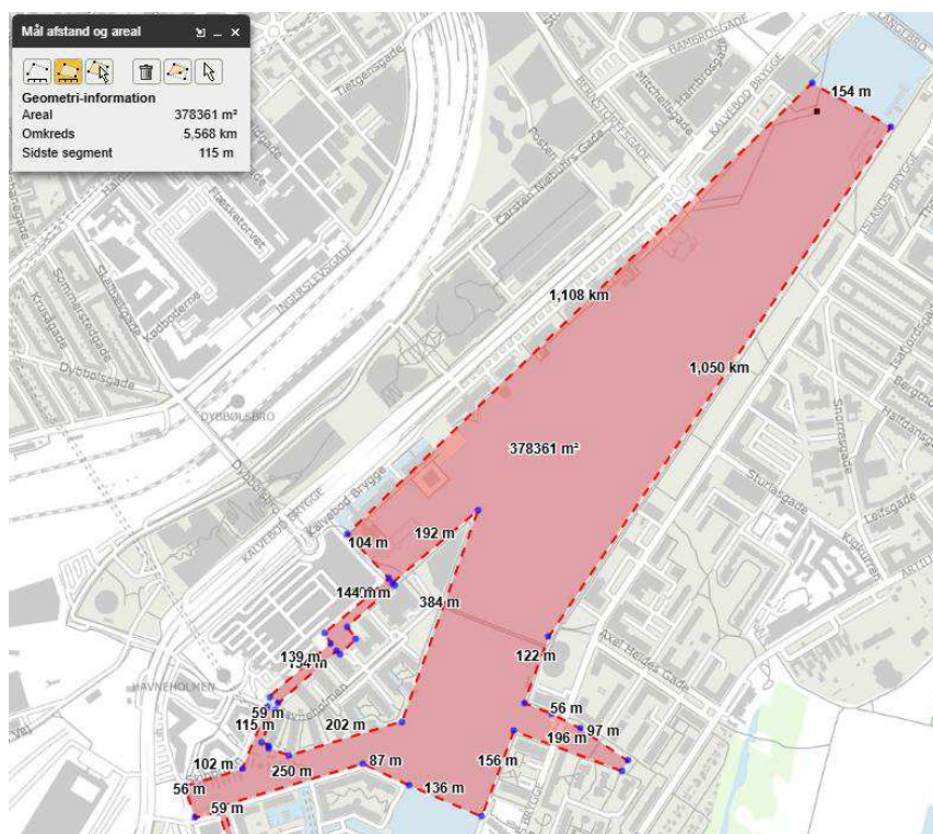
Figur 4-2 Areal fra udledningspunkt i Tømmergraven frem til repræsentativt målepunkt, Overvågningsstationen 97120111.
