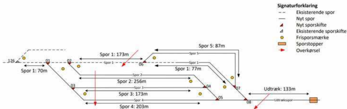
Figur 3: Skematisk gengivelse af sporanlægget på basen.
