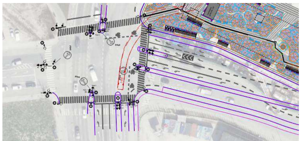
Figur 3-2 Ny geometri Havneholmen/Carsten Niebuhrs Gade/Vasbygade/Kalvebod Brygge. Ændring i krydset er Havneholmen, hvor der er to højresvingsspor og et venstre-, ligeudspor, hvor der før var to venstresvingsspor.
