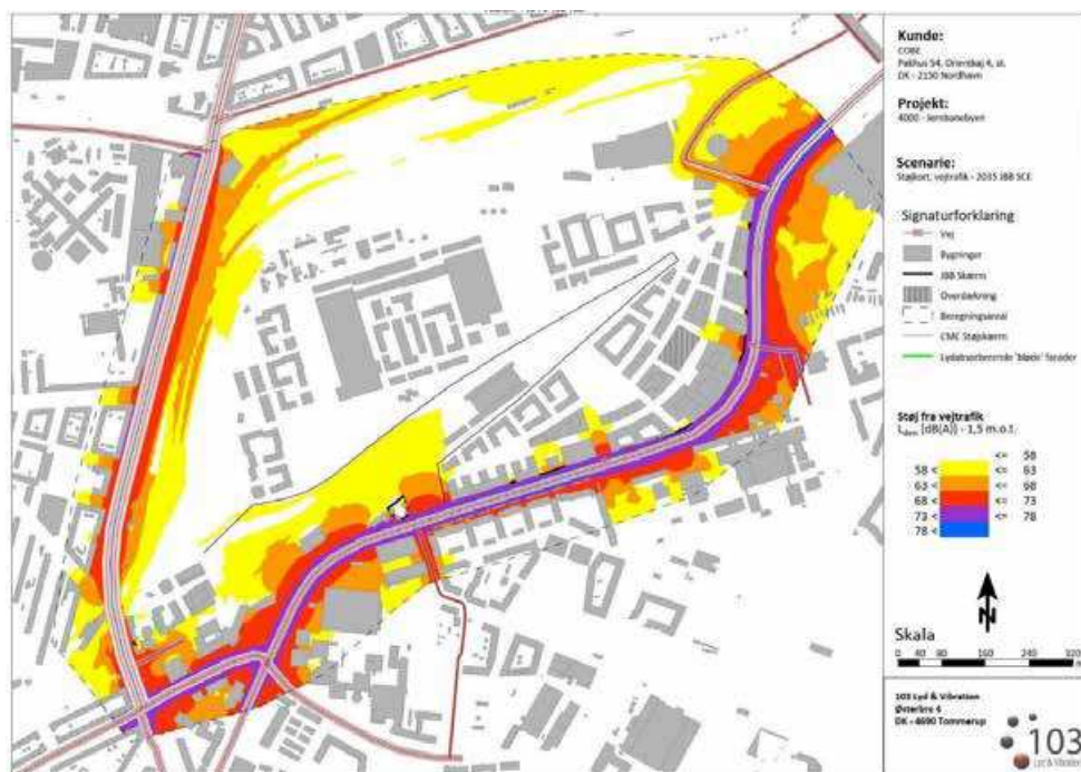
Figur 10-13 Støjbreddelseskort for vejtrafikstøj – drift i scenarie 2035. (Kort: 103 Rådgivende Ingeniører).
