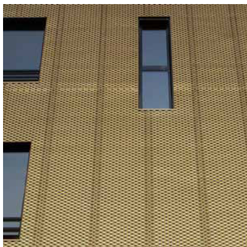
Figur 7-6 Eksempel på perforeret stålfacade med absorbent bagved.
