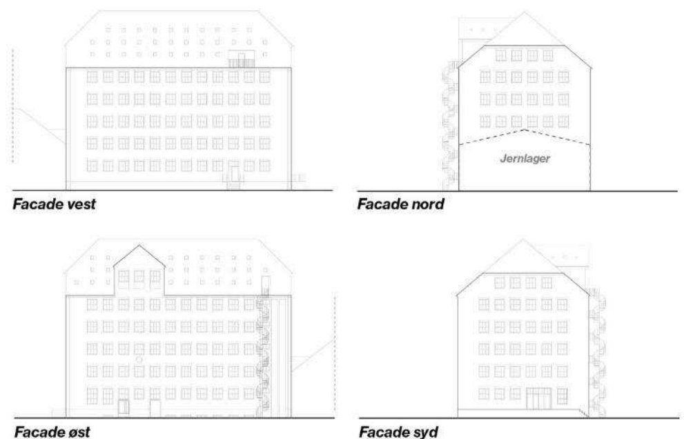
Figur 5-82 Hovedlagerets eksisterende facader. Tegning Cobe.
