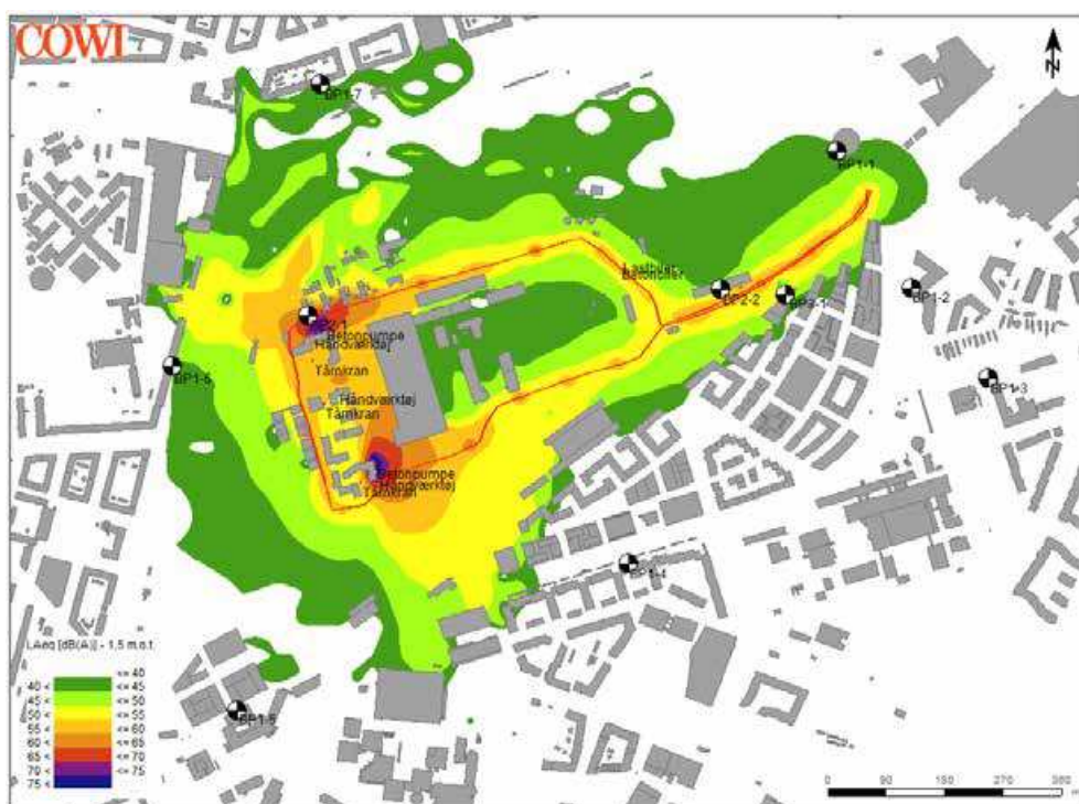
Figur 10-11 Støjudbredelseskort, Scenarie 4-2 – Byggeri i delområde 4. (Kort: COWI).
