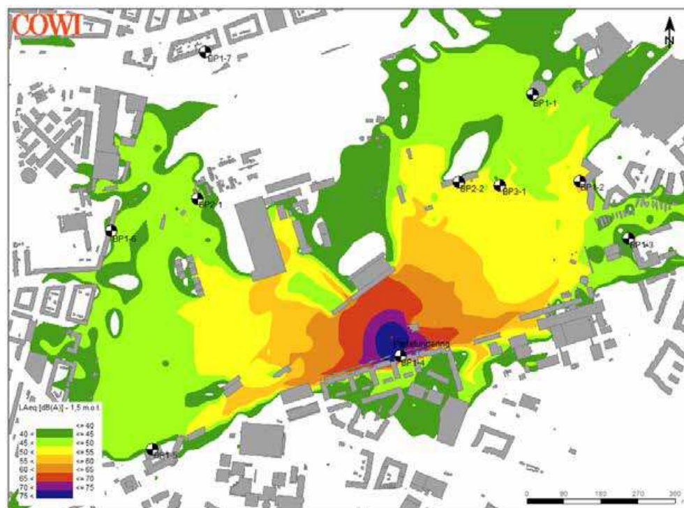
Figur 10-9 Støjudbredelseskort, Scenarie 3 – Pælefundering i delområde 2, støjniveauer uden impulstillæg. (Kort: COWI).
