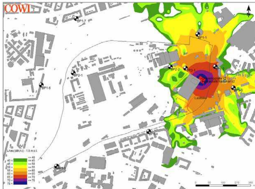
Figur 10-7 Støjdbredelseskort, Scenarie 1 – Nedrivning og opbrydning af belægninger, støjni- veauer uden impulstillæg. (Kort: COWI).
