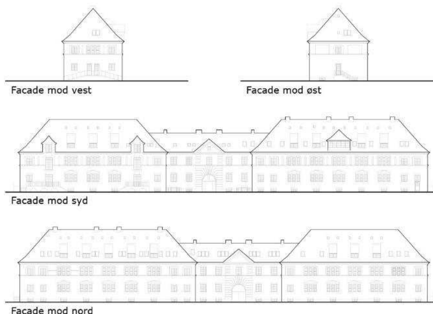
Figur 5-129 Kontor- og administrationsbygning facader. Tegning Cobe.
