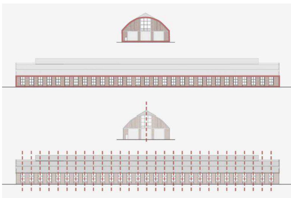
Figur 5-32 Lyntogsløftehallen facaderytme. Tegning Cobe.
