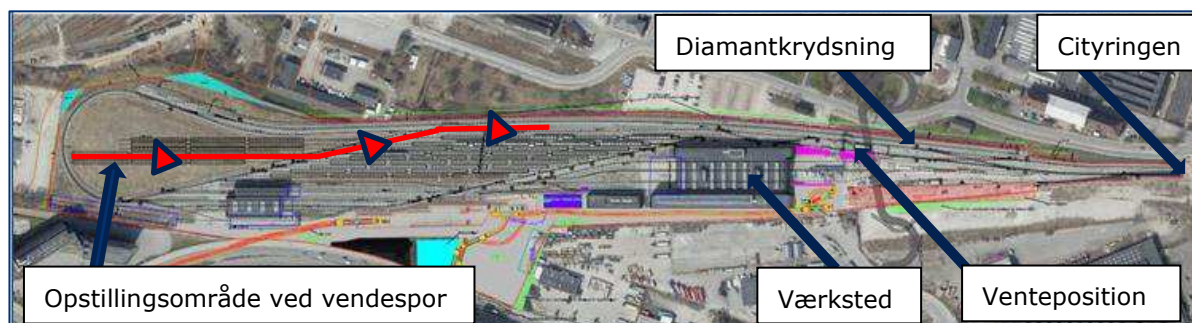
Figur 9-3. Udkørsel til Cityringen foregår fra opstillingsområde ved vendespor med 15 km/t til venteposition nordøst for værksted. Derefter køres der gennem diamantkrydsningen og videre ind på Cityringen med 40 km/t.
