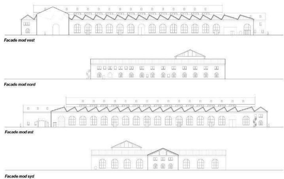
Figur 5-90 Lokomotivværkstedets eksisterende facader. Tegning Cobe.
