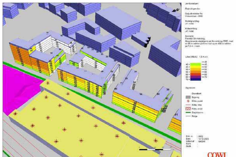
Figur 5-9 CMC. Støj udbredelseskort uden støjdæmpende foranstaltninger ved fuld udnyttelse af støjvilkår (COWI). (Beregningerne er ikke foretaget på det mest opdaterede bygningslayout).
