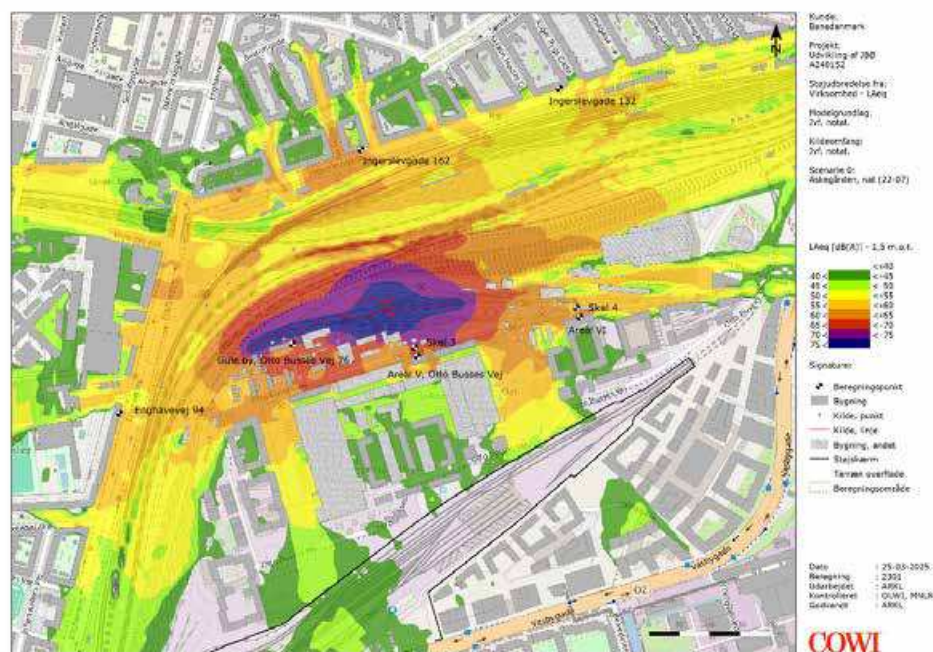
Figur 4 Støjdbredelseskort for Askegården fremtidige forhold uden mitigering.
