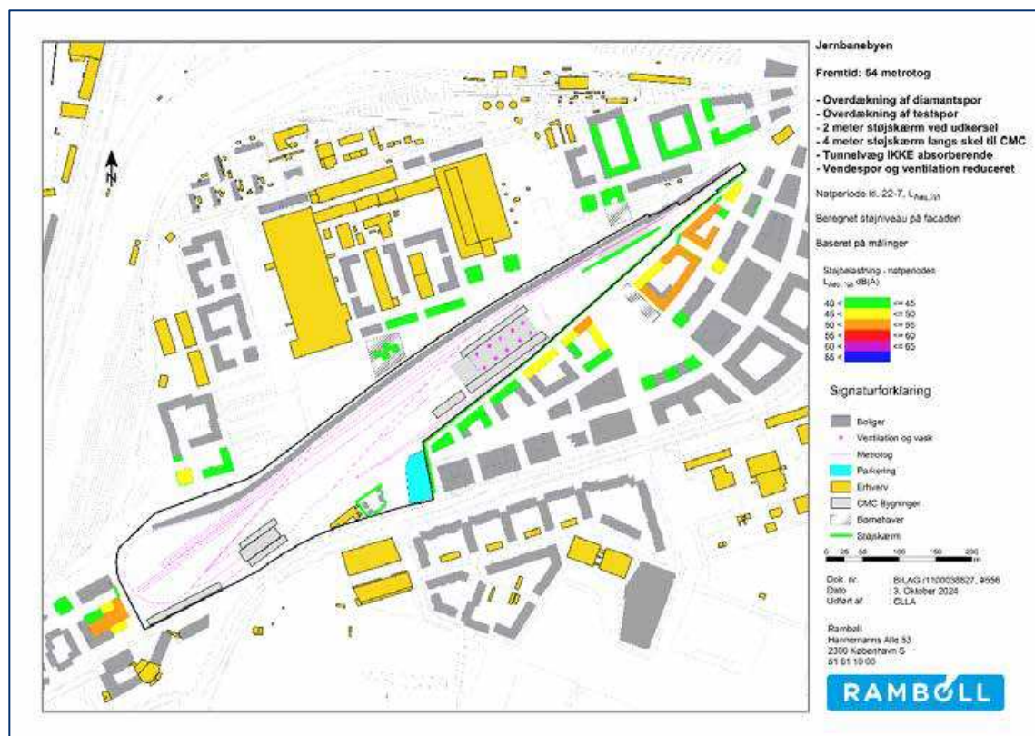
Figur 20-12. Scenarie: Reduceret støj med overdækning Beregnet støjniveau på facaden i natperioden.
