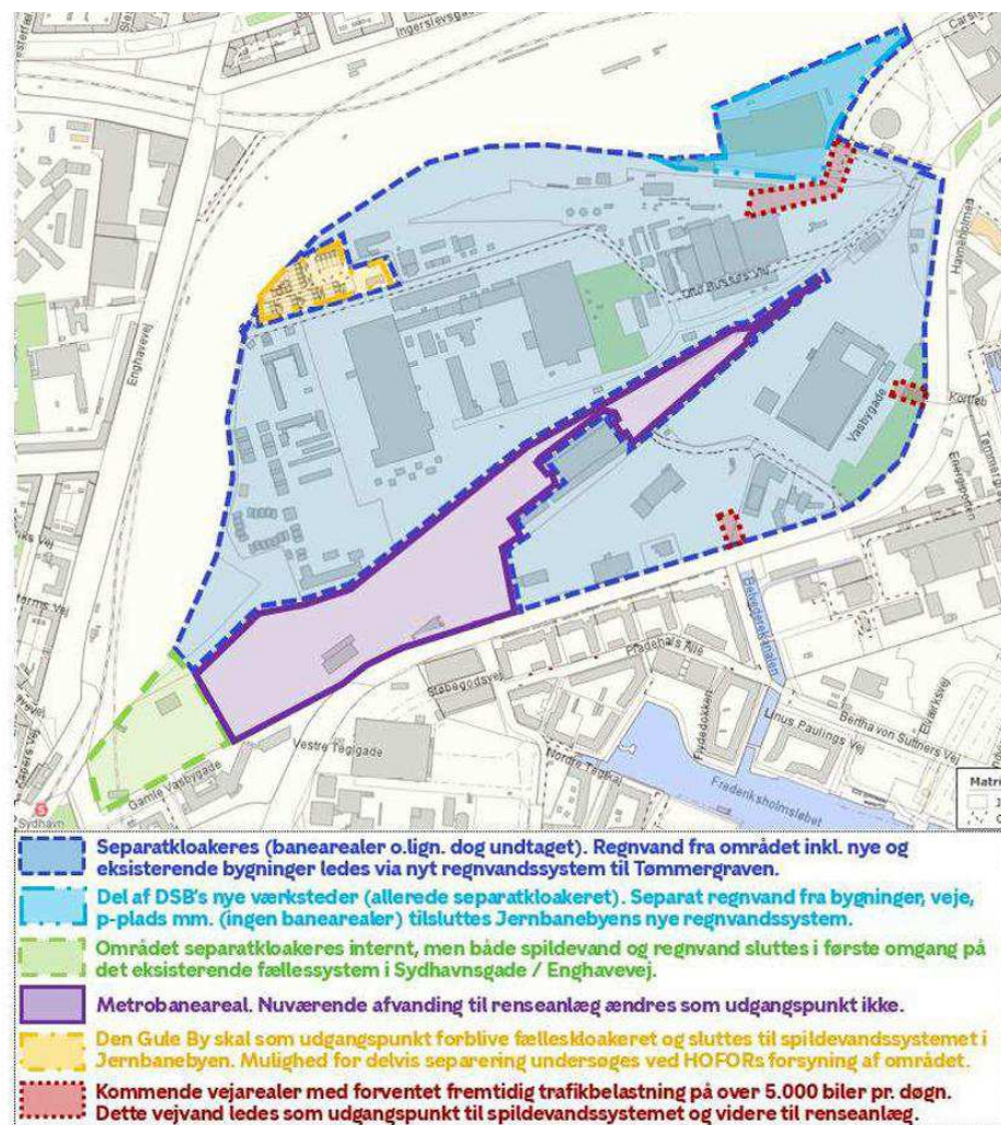
Figur 18-3 Oversigt over området i Jernbanebyen iht. Københavns Kommunes Spildevandsplan 2018, som efter byudviklingen leder til hhv. fælleskloakledning og regnvandsledning.
