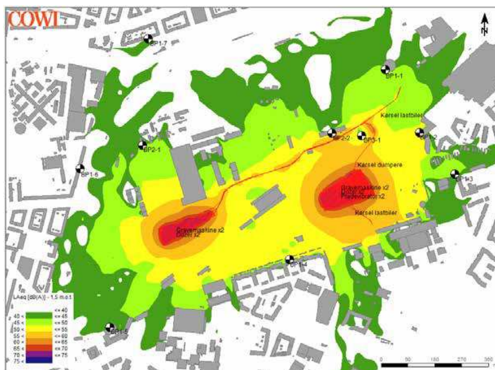
Figur 10-8 Støjudbredelseskort, Scenarie 2 – Terrænregulering. (Kort: COWI).
