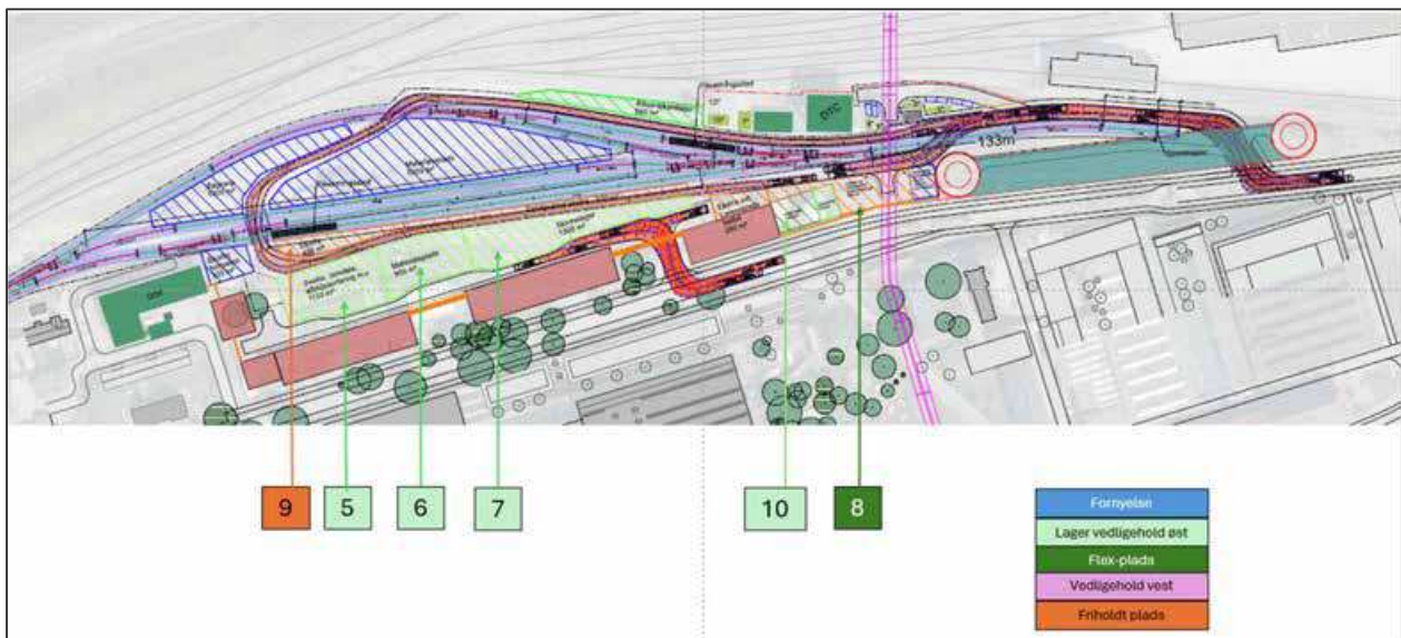
Figur 6: Skitseløsning fra figur 2, hvor dedikerede arealer til lagrene til manuelt Vedligehold øst, administreret af Lager & Logistik er markeret.
