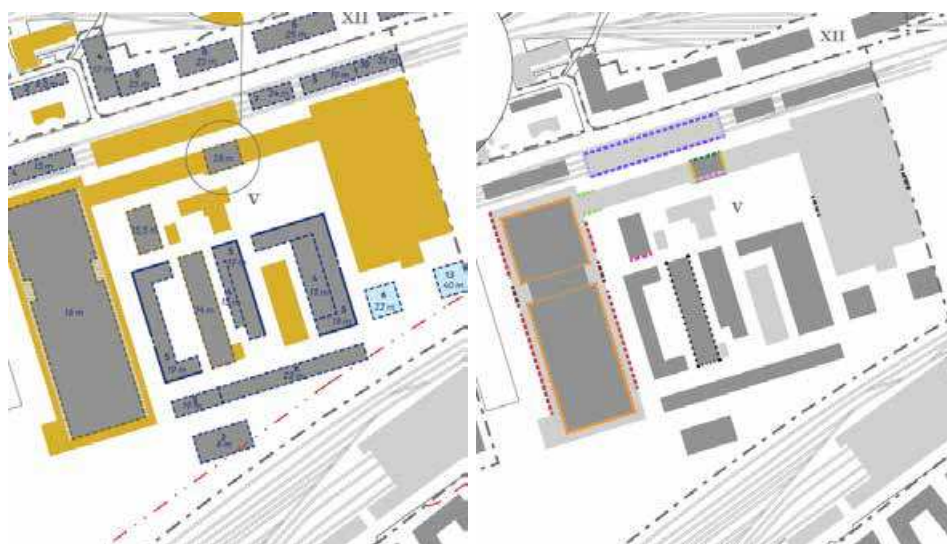
Figur 5-58 Tv. udsnit af tegning 5b3 · Bebyggelsens omfang og placering · IV, V, VII, XII, som viser hvilke muligheder der er for påbygning på Trykløftværkstedet. Th. udsnit af tegning 6d2 · Bevaring - ydre fremtræden · IV, V. Københavns Kommune, 2026.
