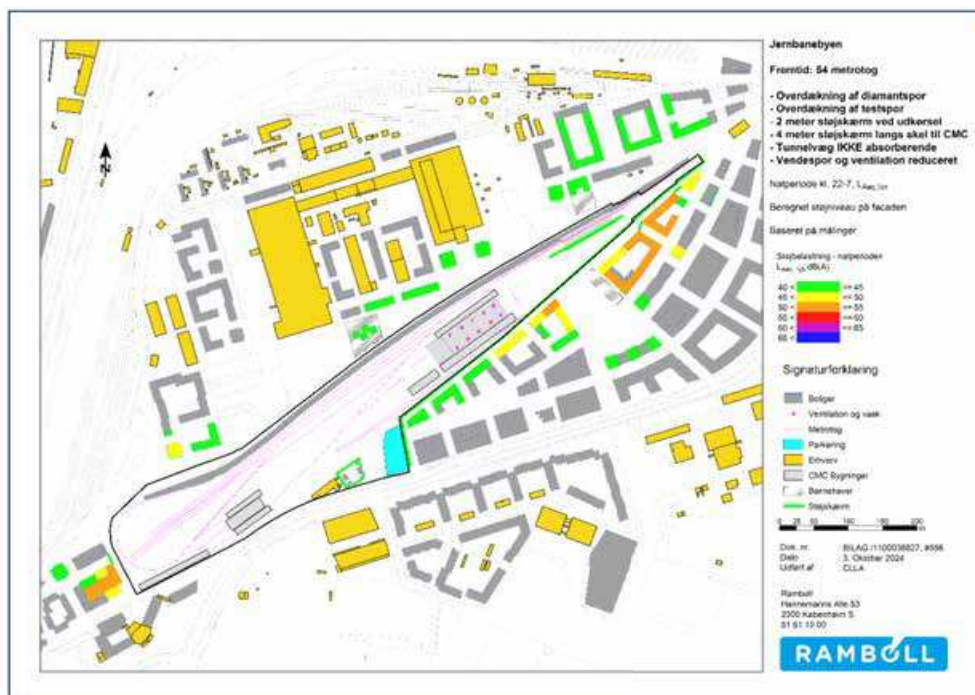
Figur 6-14 CMC. Støjdæmpende tiltag i form af overdækning når planlovens § 15, stk. 2, nr. 29, jf. § 15a, stk. 1 finder anvendelse. Facadestøjskort natperioden (Rambøll).
