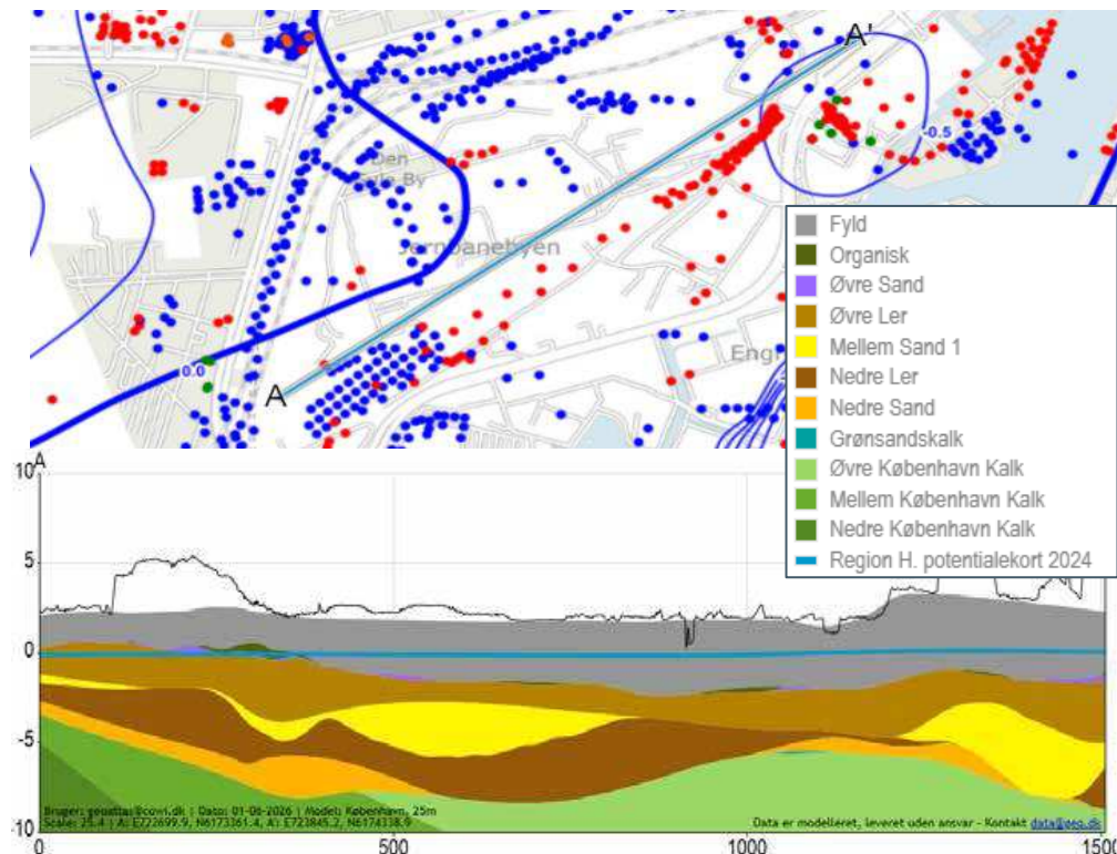
Figur 17-2 Geologisk lagfølge i projekt- og planområdet samt kote for grundvandsspejlet i det primære magasin (kalkmagasinet), modelleret data ud fra boreprofiler. (Figur: COWI, 2026).
