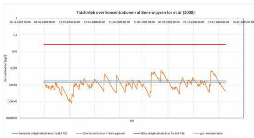
Figur 4-3: Benz(a)pyren koncentration i hele Tømmergraven over tid for år 2008
