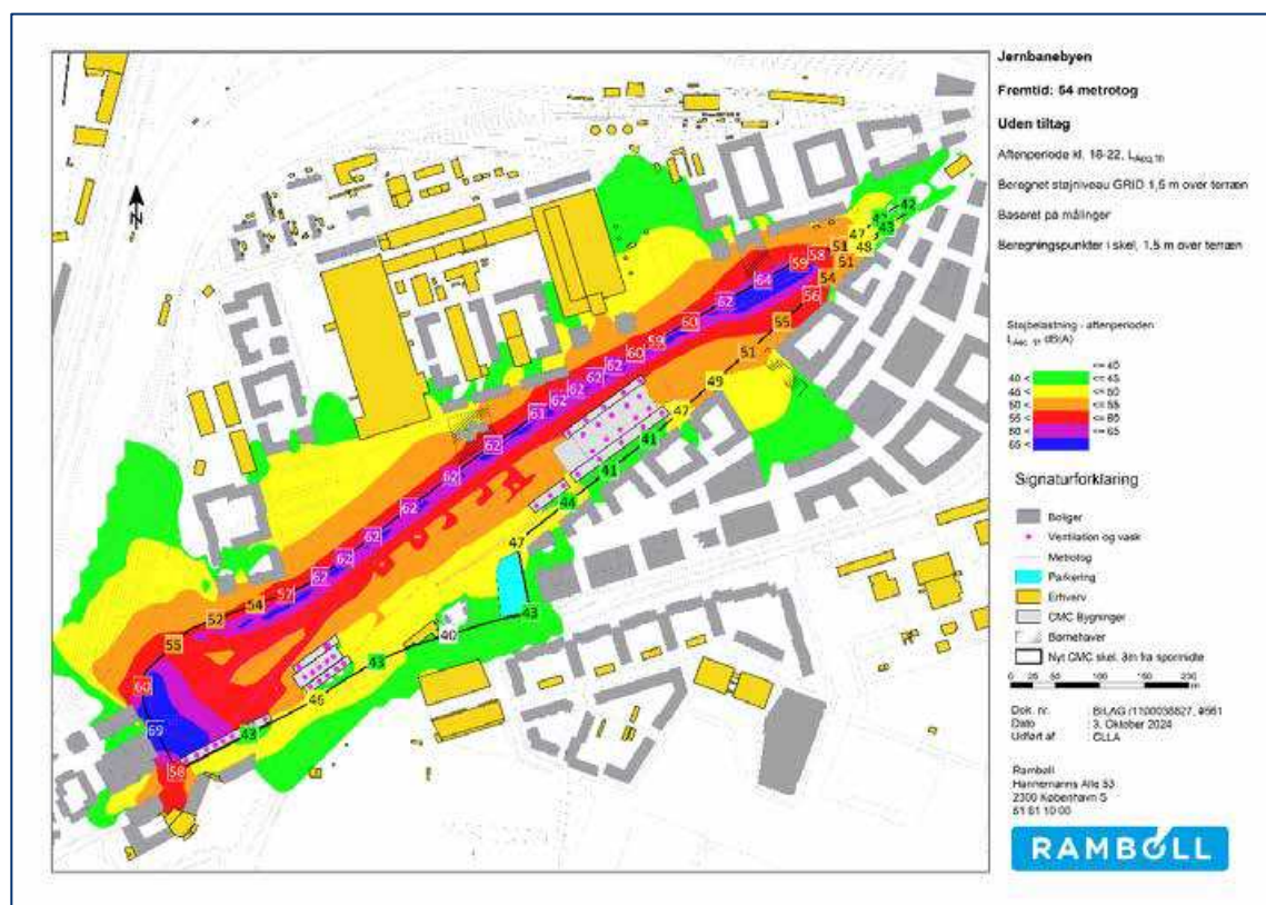
Figur 20-3. Scenario: Uden støj dæmpende tiltag. Beregnet støjniveau i skel og støjkontour 1,5 meter over terræn i aftenperioden.
