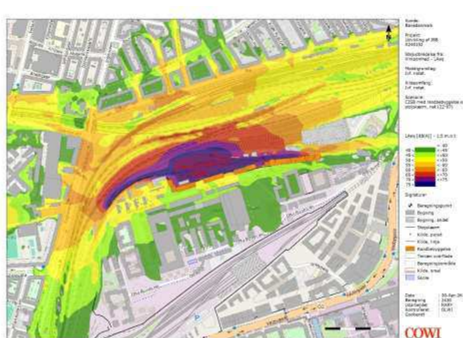
Figur 5 Støjubredeleskort for CISB fremtidige forhold – natperioden.
