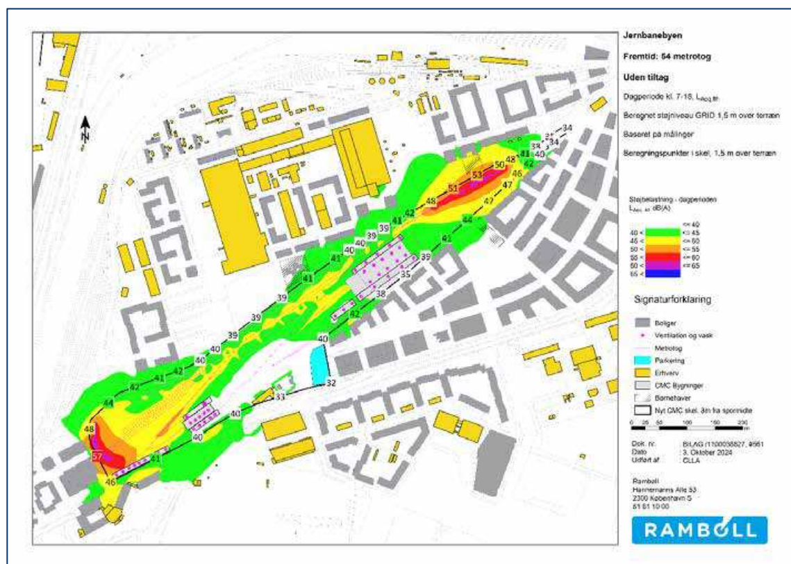
Figur 20-1. Scenario: Uden støj dæmpende tiltag. Beregnet støjniveau i skel og støjkontour 1,5 meter over terræn i dagperioden.
