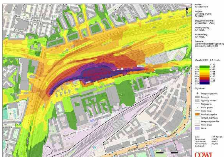
Figur 5-15 CISB. Støjudbredelse natperioden.
