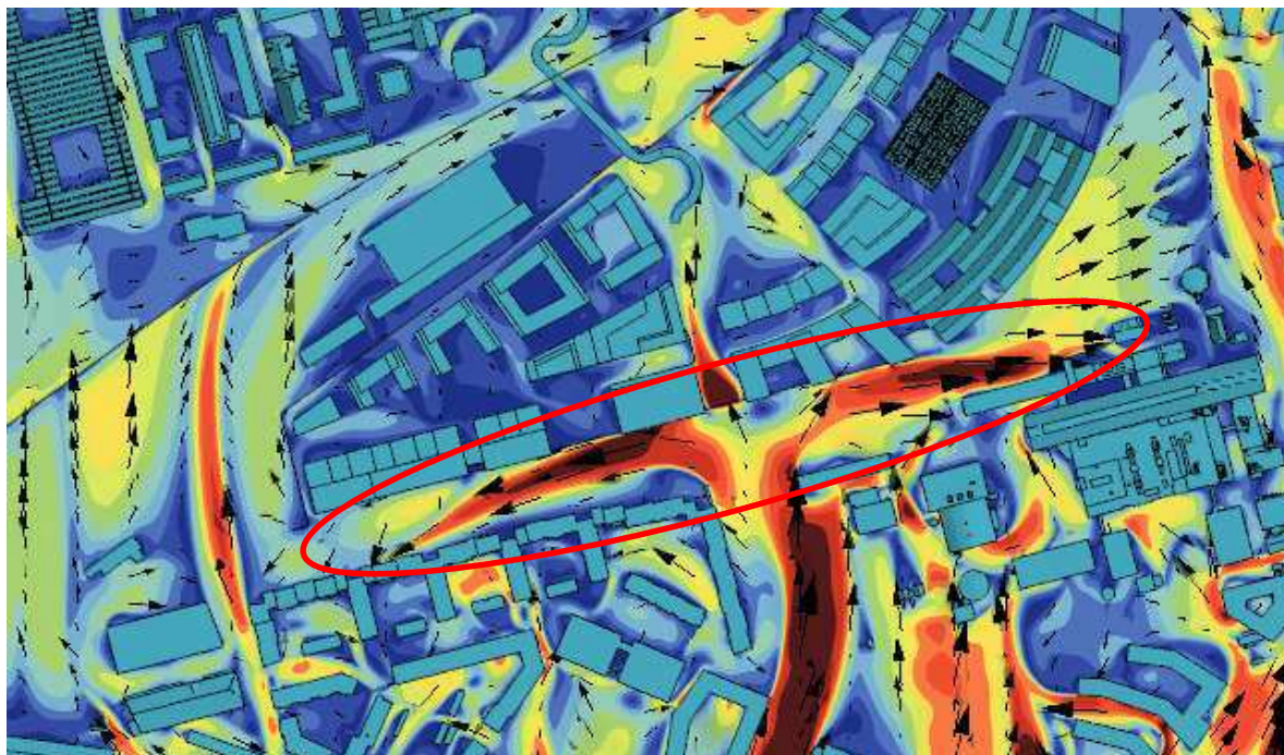
Figur 4.8 Vasbygade: Relativ vindhastighed (i forhold til vinden i 10 m højde uforstyrret) beregnet 1,5 m over gadeniveau i Jernbanebyen. Vind fra syd.
