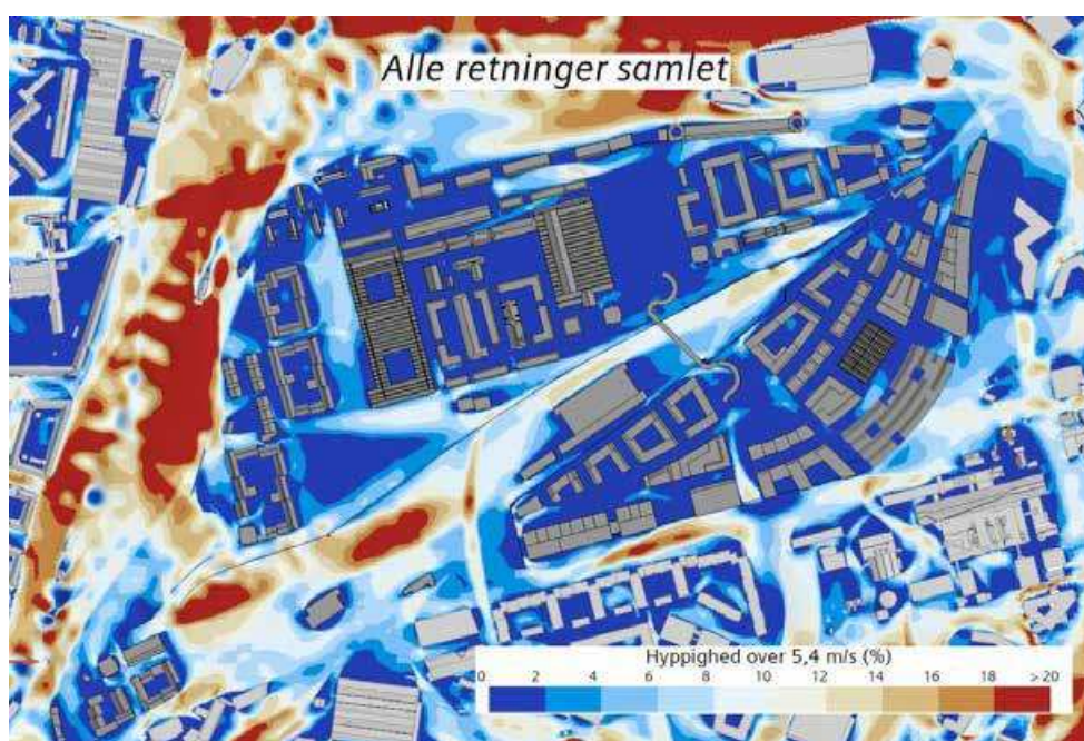
Figur 12-8 Vindkomfort beregnet 1,5 m over gadeniveau i Jernbanebyen. Nærbillede: hyppighed for overskridelse af 5,4 m/s, der helst skal være under 1 % hhv. 6 % for de to aktiviteter stillesiddende og stående. Alle vindretninger, årsklima. Bilag D – Vindmiljøanalyse – Jernbanebyen. (Figur: COWI).
