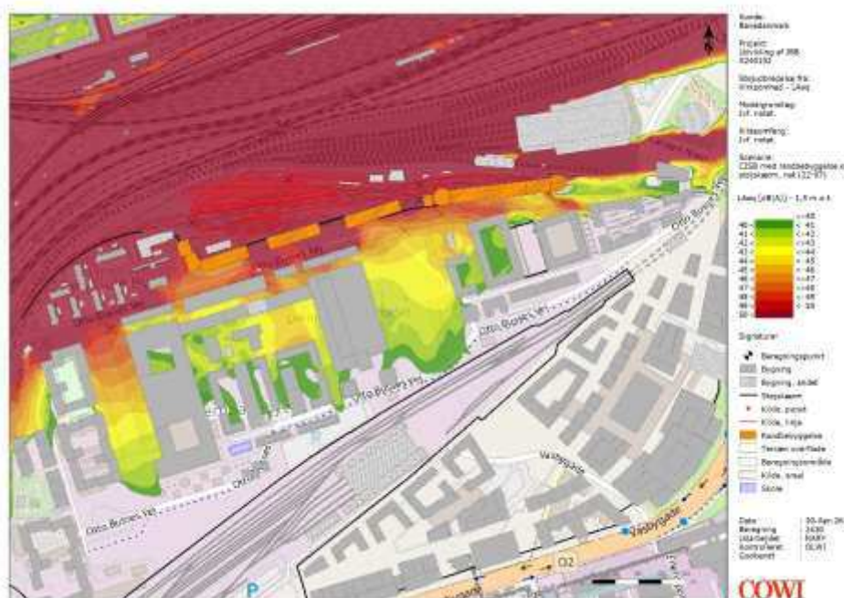
Figur 8 Støjkonturkort for fremtidige aktiviteter på CISB i natperioden med 1 dB intervaller.
