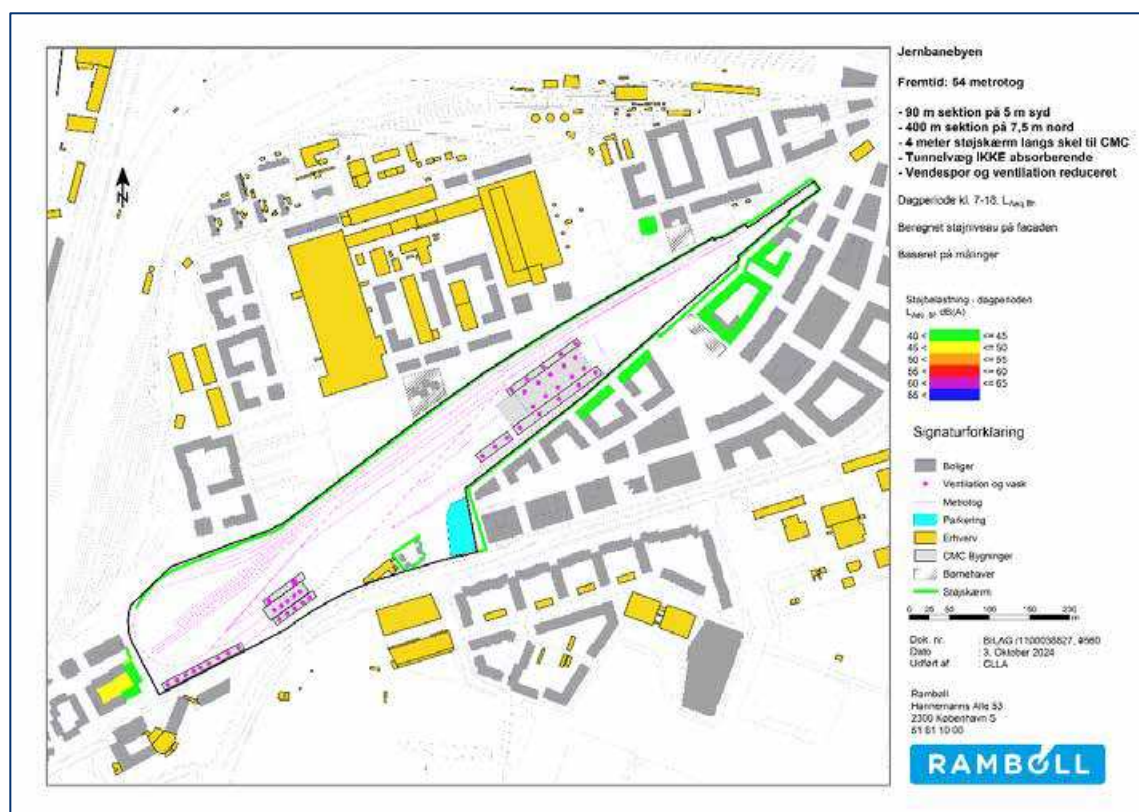
Figur 20-14. Scenarie: Reduceret støj uden overdækning. Beregnet støjniveau på facaden i dagperioden.
