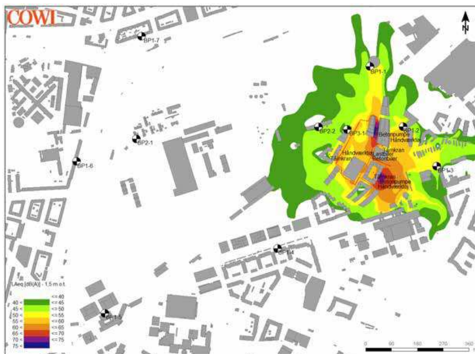
Figur 10-10 Støjudbredelseskort, Scenarie 4-1: Byggeri i delområde 1. (Kort: COWI).
