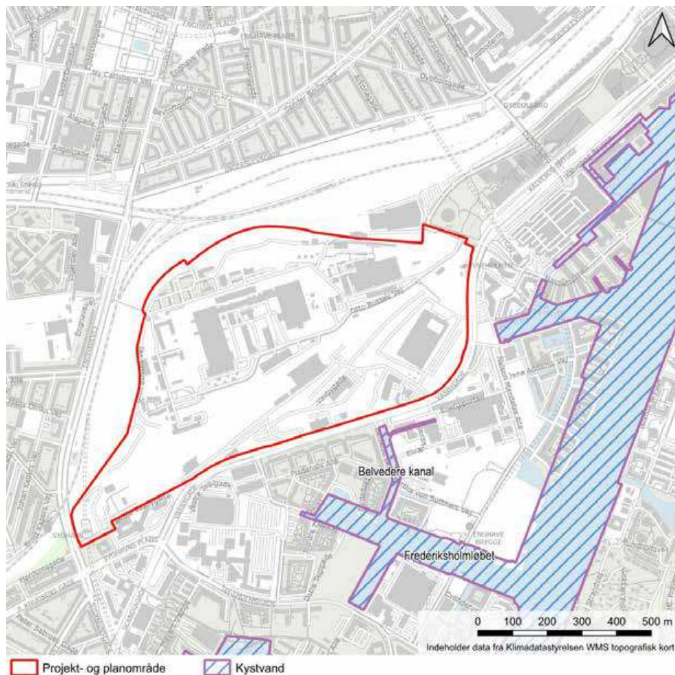
Figur 18-2 Oversigt over det målsatte kystvandområde nær projekt- og planområdet.
