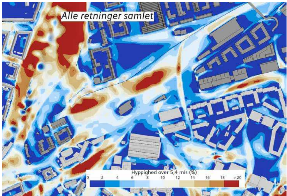
Figur 4.6 Nærbillede: hyppighed for overskridelse af 5,4 m/s beregnet 1,5 m over gadeniveau i Jernbanebyen. Alle vindretninger, årsklima. Beregnet ud fra Weibull-parametrene og hyppighederne i Tabel 3.1. Aktivitet: siddende og stående.
