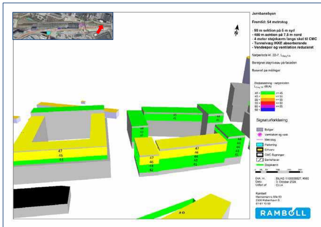
Figur 20-22. Scenarie: Reduceret støj uden overdækning. 3D opstalt af beregnet støjniveau på facaden i natperioden. Grå facader er udsat for støj med niveauer under 40 dB. Bygninger nord for tunnelrampen.
