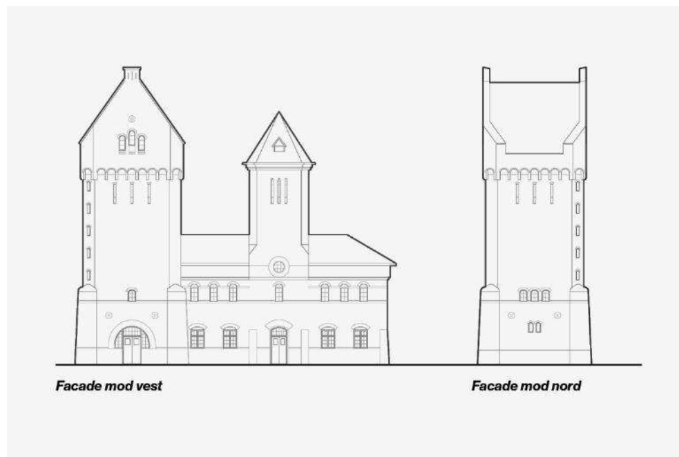
Figur 5-95 Vandtårnets facader mod vest og nord. Tegning Cobe.
