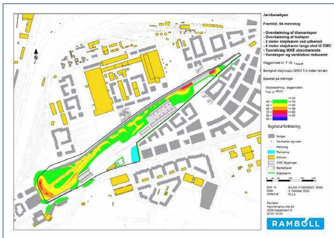
Figur 20-7. Scenarie: Reduceret støj med overdækning. Beregnet støjniveau 1,5 meter over terræn i dagperioden.
