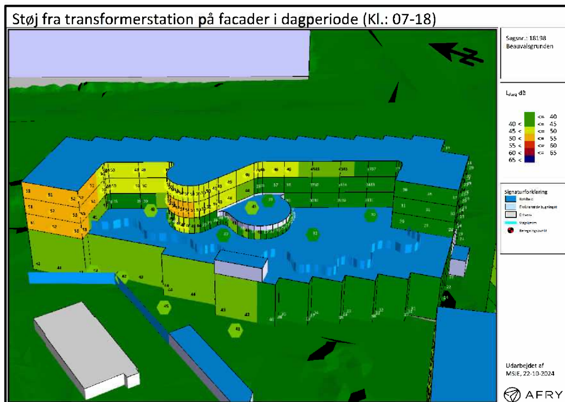
figur 4-8 Støj fra Transformerstation – Facadestøjskort
