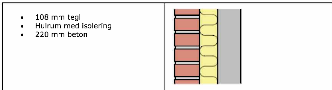
Figur 5-2 Eksempel på facadekonstruktion
