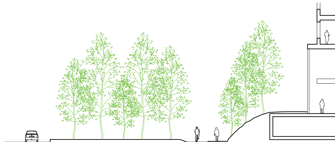
Principalsnit c-c, som viser blødt formet terræn og kantzone mod det rekreative areal
