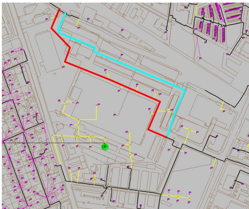
Figur 2 Udbygget ledningsnet for Grønttorvsområdet
