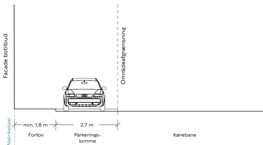
Snit A-A
