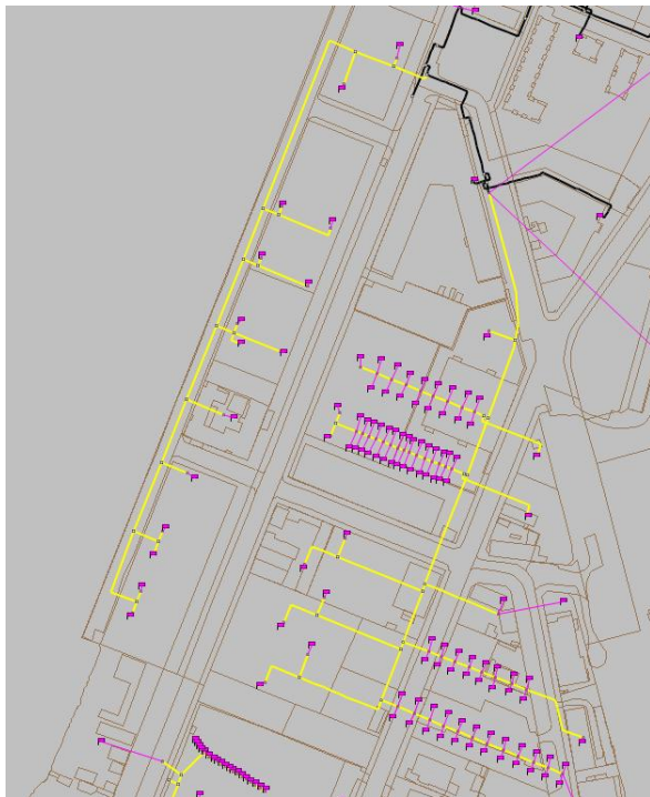
Figur 3 Udbygget ledningsnet for Artillerivej Syd
