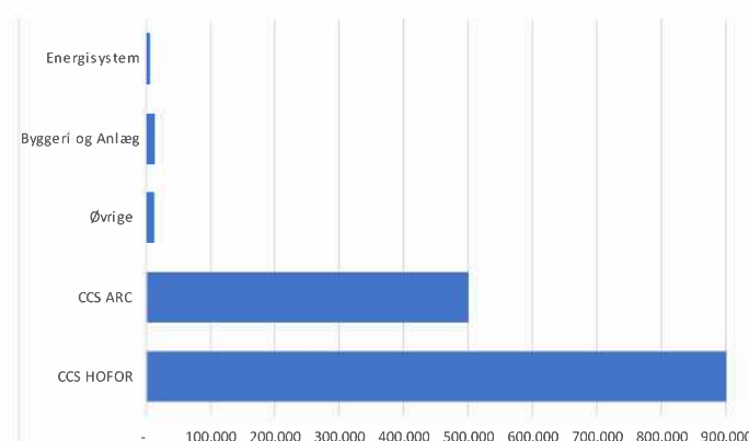
Figur 12: Effekt af initiativer i handleplanen, udledningsreduktion per indsatsområde for de geografiske udledninger
