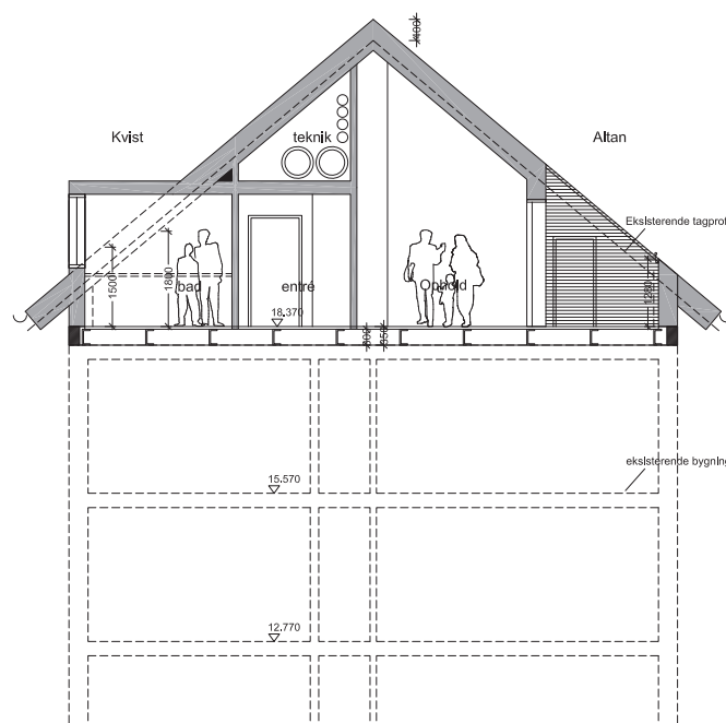
Tværsnit i tagbolig
