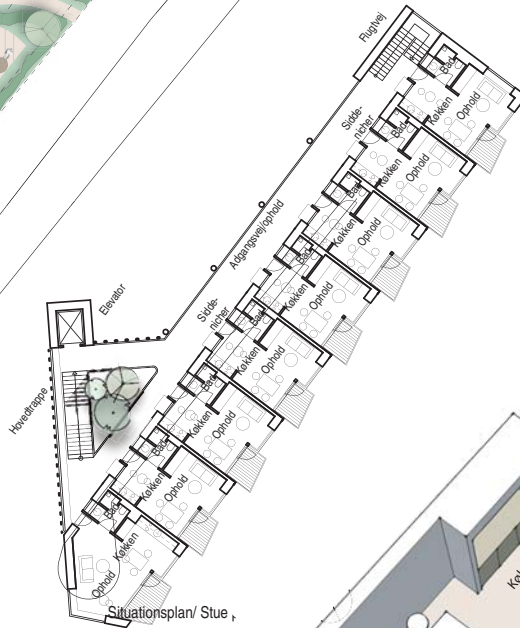
PLAN NORMALETAGE
