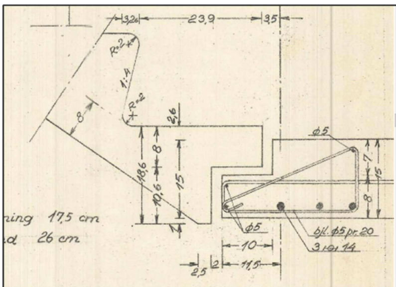
Figur 6.3. Samlingsdetalje mellem præfabrikeret trappeløb og insitustøbt repos.
