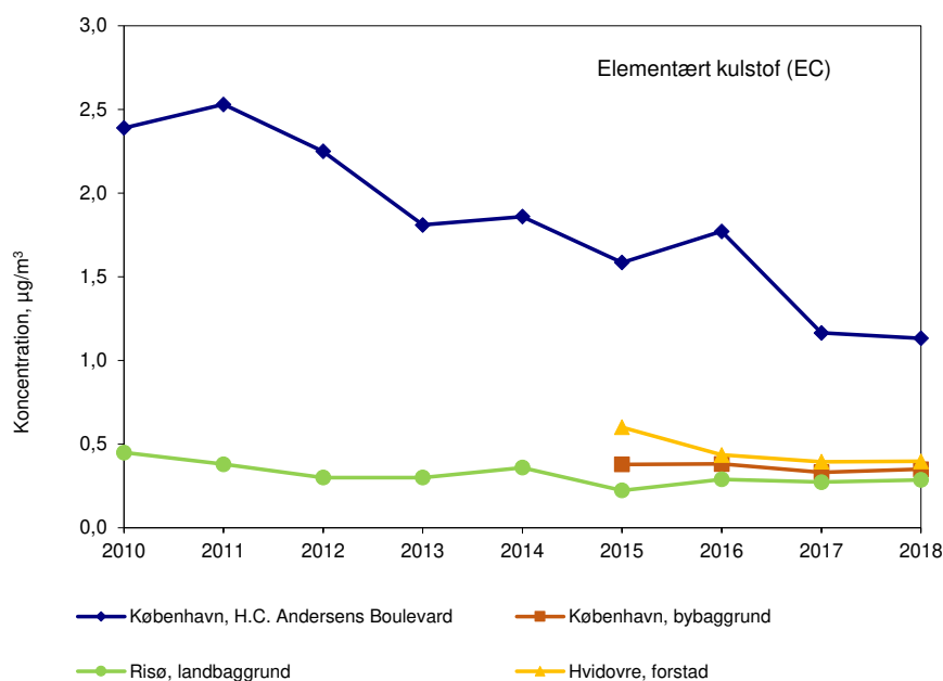
Figur 3.2. Udviklingstendens for årsmiddelkoncentrationen af elementært kulstof siden opstart af målingerne i 2010 (Ellermann et al., 2020).
