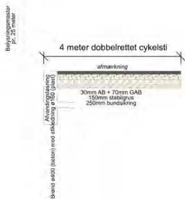
Figur 3: Principtværsnit for dobbeltrettet cykelsti på bar mark
