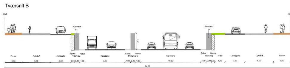
Figur 49 Tværsnit B på H. C. Andersens Boulevard mellem Jarmers Plads og Studiestræde, hvor man kigger ud af tunnellen.
