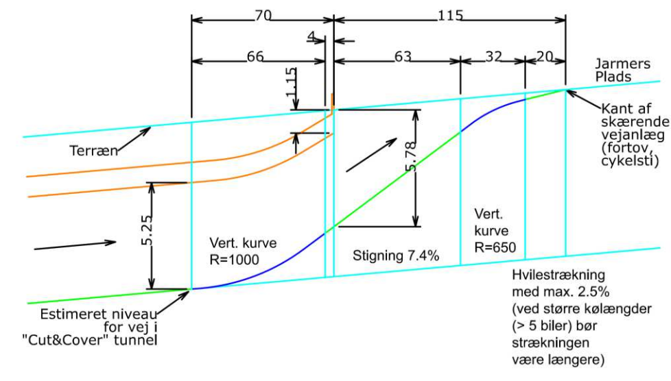
Figur 43 Princip for rampes længdeprofil fra hovedtunnel til terræn (opkørsel til tunnel) ved Jarmers Plads, hvor der er ca. 1 m's terrænforskel.
