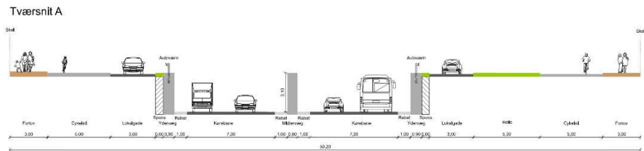
Figur 48 Tværsnit A på H. C. Andersens Boulevard mellem Rysensteensgade og Niels Brock Gade, hvor man kigger ud af tunnellen. Det bemærkes, at arealet med helle (grøn markering) på overfladen vil udgå i rampeudmundingen oppe omkring signalanlægget, hvor arealet er disponeret til højresvingbane og skillehelle som 3. tilfartsspor i tunnelens rampeåbning.
