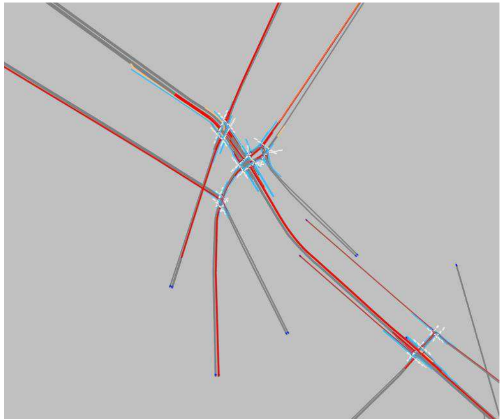
Figur 116 Figuren viser den maksimale kølængde (rød) i scenarie 2a ved krydset H. C. Andersens Boulevard / Jarmers Plads. Ses at køen går helt tilbage til rampekrydset H. C. Andersens Boulevard / Rysensteensgade i morgenspidsperioden (kl. 7:00-9:00) [95% fraktilen].
