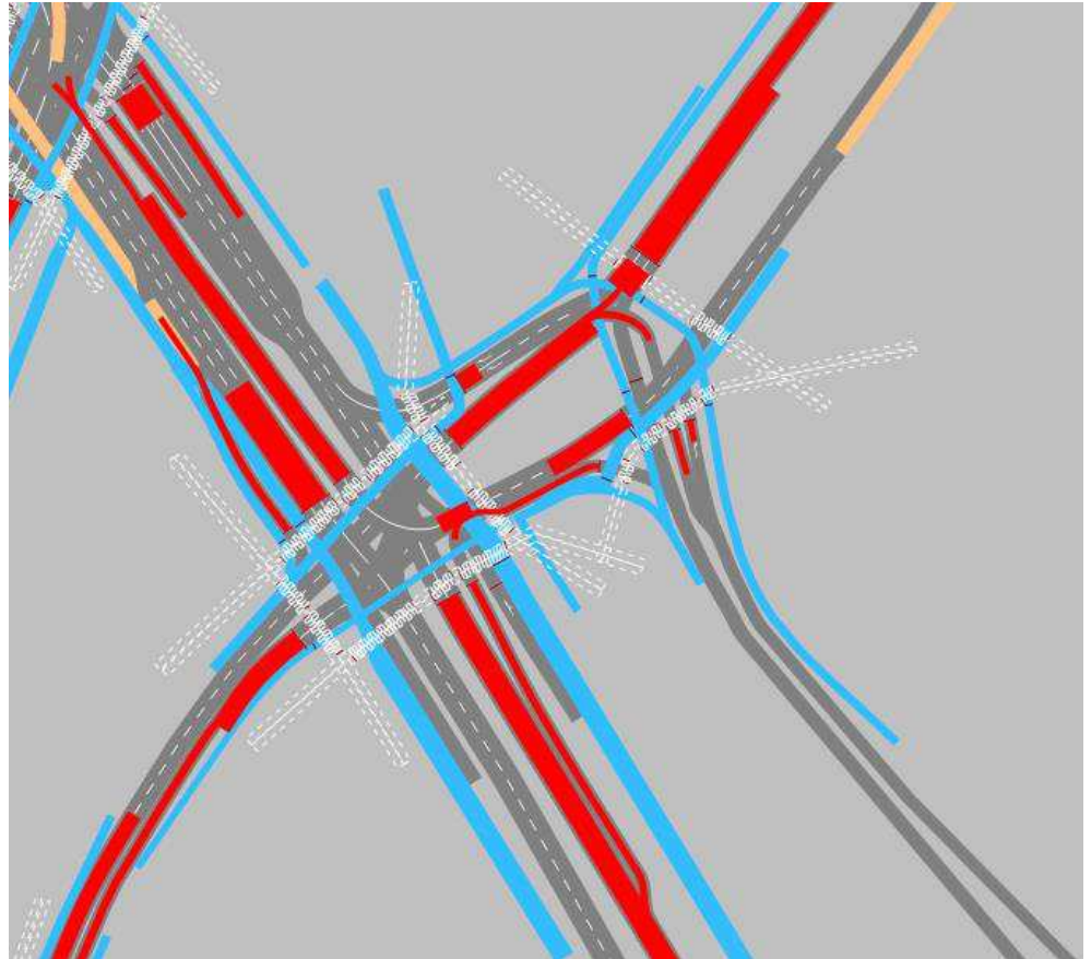
Figur 78 Figuren viser den maksimale kø længde (rød) i basisscenarie 2035 ved krydset H. C. Andersens Boulevard / Jarmers Plads i eftermiddagsskiftperioden (kl. 15:00-17:00) [95% fraktilen].
