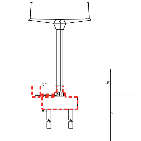
Principskitse for brofæste på land
