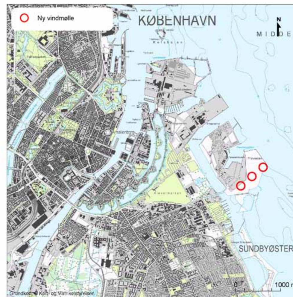
Figur 4.1 Oversigt over vindmøllernes placering på Prøvestenen.
