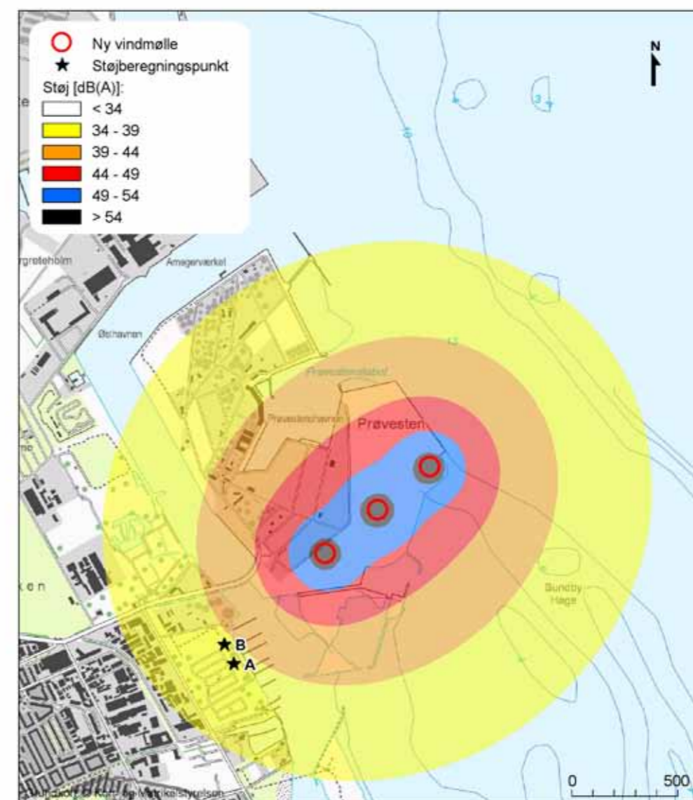
Figur 12.2 Beregnet støjdbredelse for møllerne ved vindhastighed på 8 m/s.
