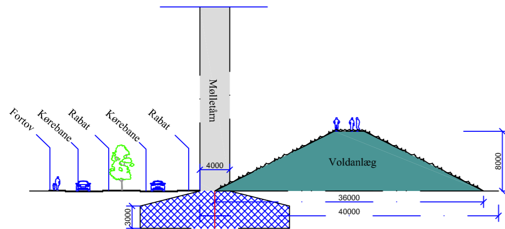
Figur 4.2 Skitse med placering af møllerne ved volden.
