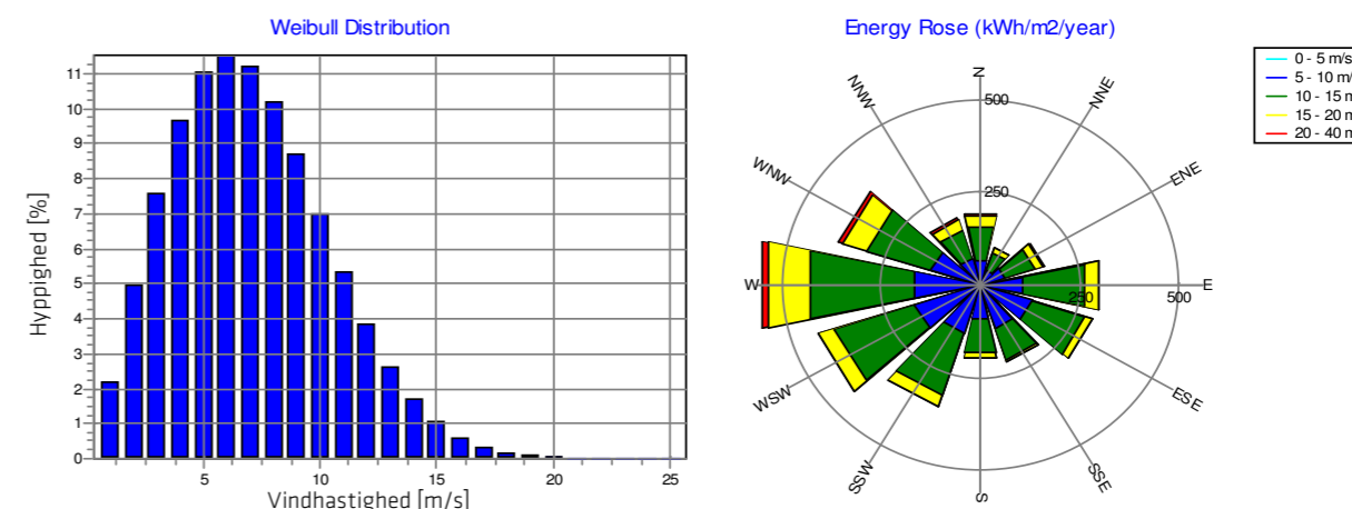
Figur 5.1 Vindhastighedsfordeling.
