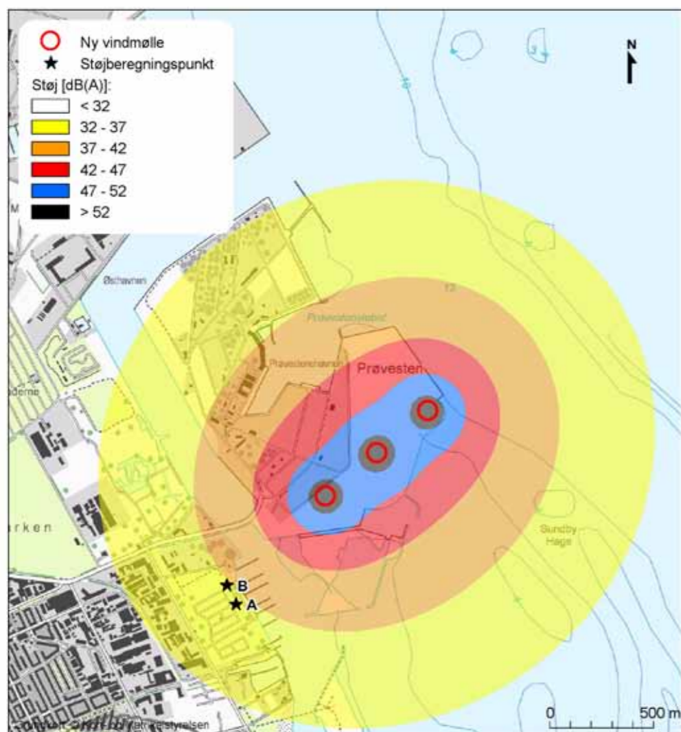
Figur 12.1 Beregnet støjdbredelse for møllerne ved vindhastighed på 6 m/s.
