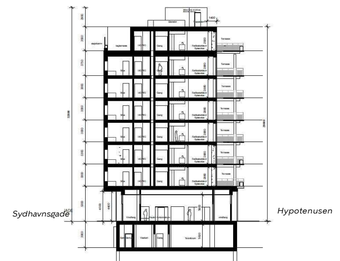
Principsnit
