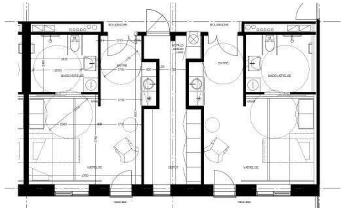
Plantegning der viser boligprincip 1 rums plejebolig nettoareal - 36 kvm
