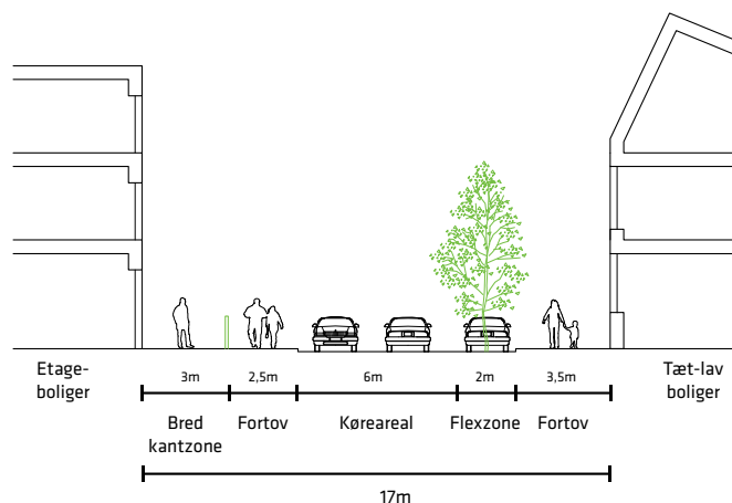
Figur 4.2. Principsnit af den interne vej i lokalplantillæggets område, jf. tegning 3.2
