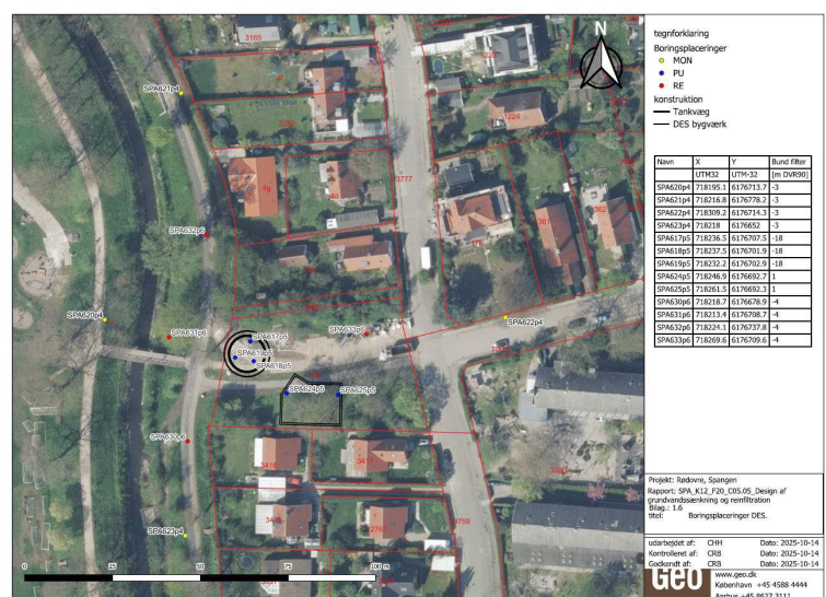
Figur 7: Placering af borer til grundvandssænkning samt monitorering ved DES. Der skal ikke placeres borer i umiddelbar nærhed af det §3 beskyttede område.
