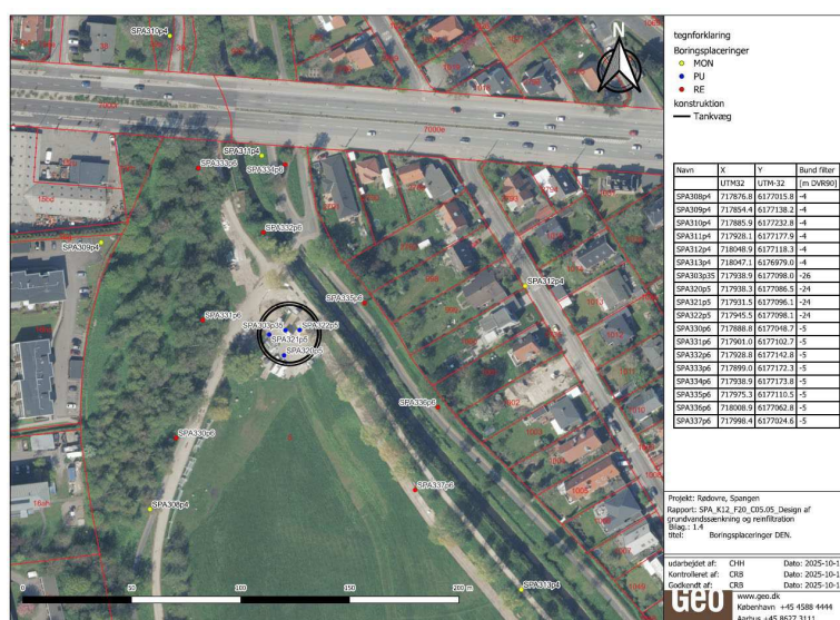
Figur 6: Placering af borer til grundvandssænkning samt monitorering ved DEN. Alle borer er uden for det §3 beskyttede område.
