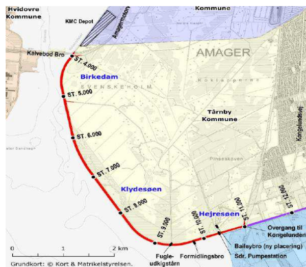
Figur 21: Plantegning af hævnning af Vestamager Kystdige, 2012.
