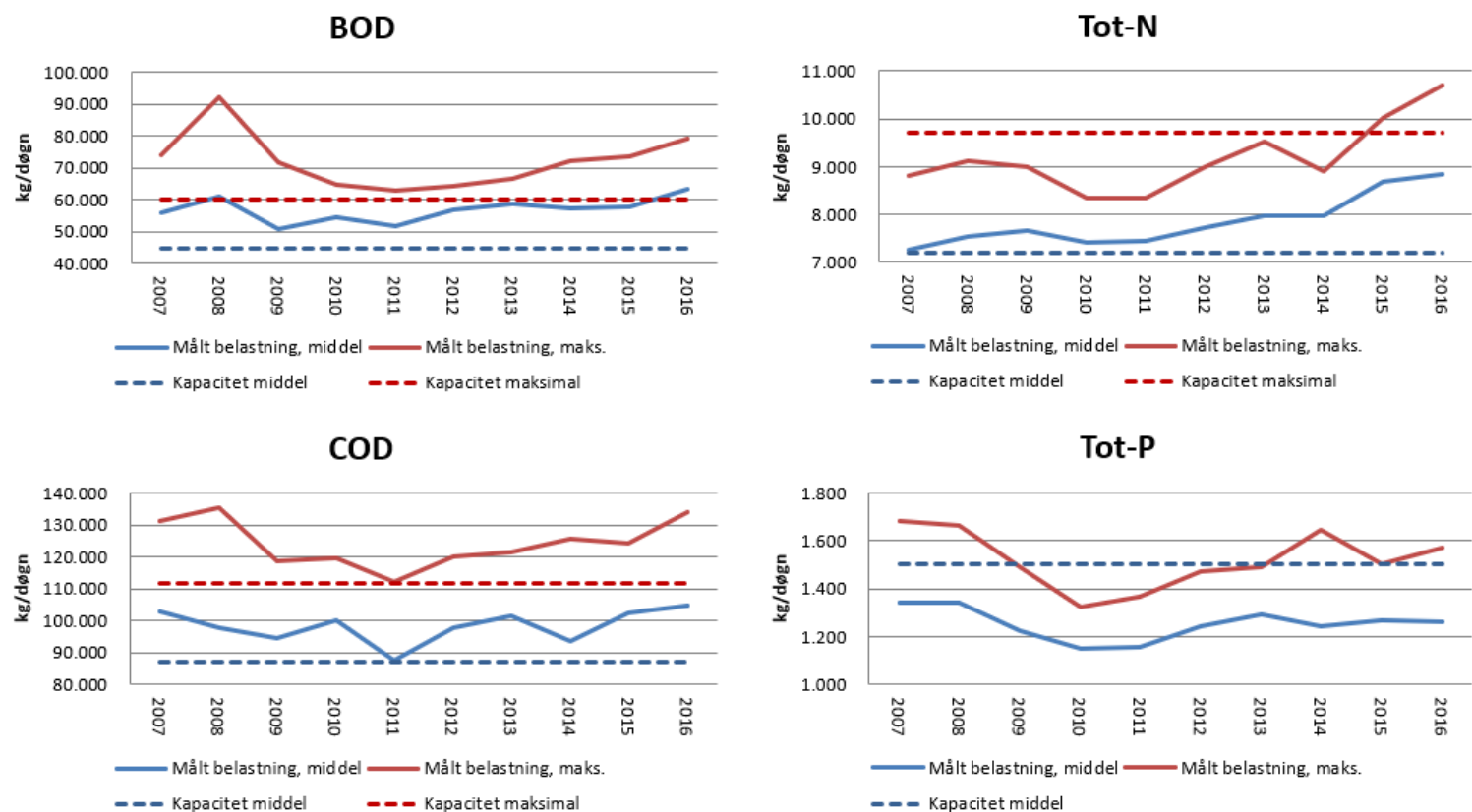
Figur 4.1: (Bearbejdn af Data 60 og 85 % belastning, Københavns Kommune, 2018) på baggrund af data fra BIOFOS (Data 60 og 85% belastning, BIOFOS, marts 2017). Middelbelastning svarer til 60 %-fraktil og maksimal belastning svarer til 85 %-fraktil.
