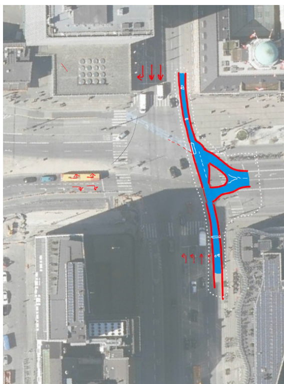
Figur 9. Kryds 13. Lukke Vesterbrogade og tilpasse krydset – Den viste udformning tager afsæt i scenarie 3, men udformningen svarende til scenarie 4 er ikke så meget anderledes, at det påvirker estimeret pris
