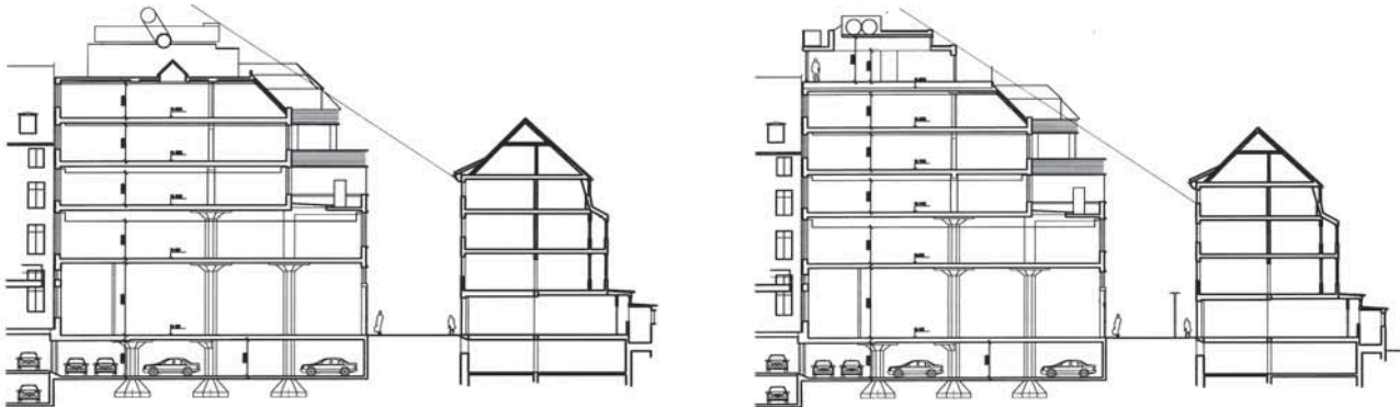
Snittegning visende lysforhold i gaden ved det eksisterende ventilationsanlæg på taget af Sværtegadebebyggelse og ved realisering af ny penthouseetage som erstatning herfor. Som det ses bliver lysforholdene på modstående gadefacader forbedret ved realisering af den ny penthouseetage.
