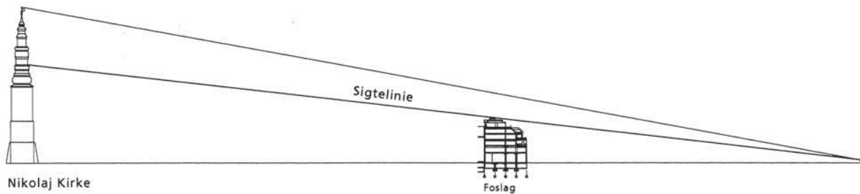
Snittegning visende vue fra Kongens Have til Nikolaj Kirke med det eksisterende ventilationsanlæg på taget af Sværtegadebebyggelse og ved realisering af ny penthouseetage som erstatning herfor.
