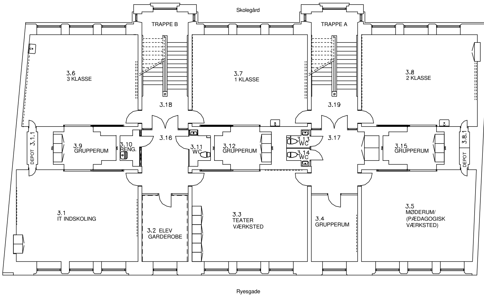
2 SALSPLAN
