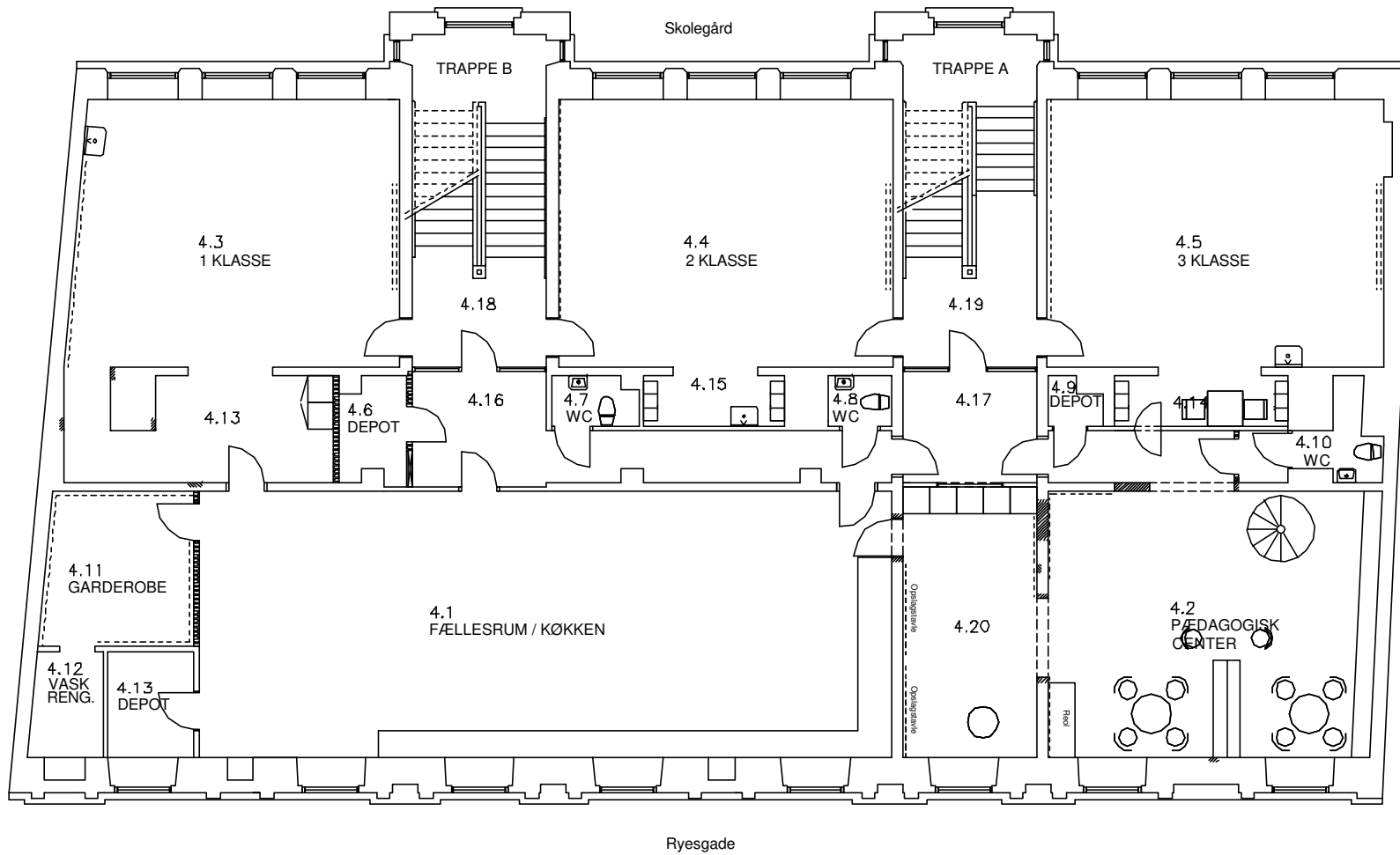
3 SALSPLAN
