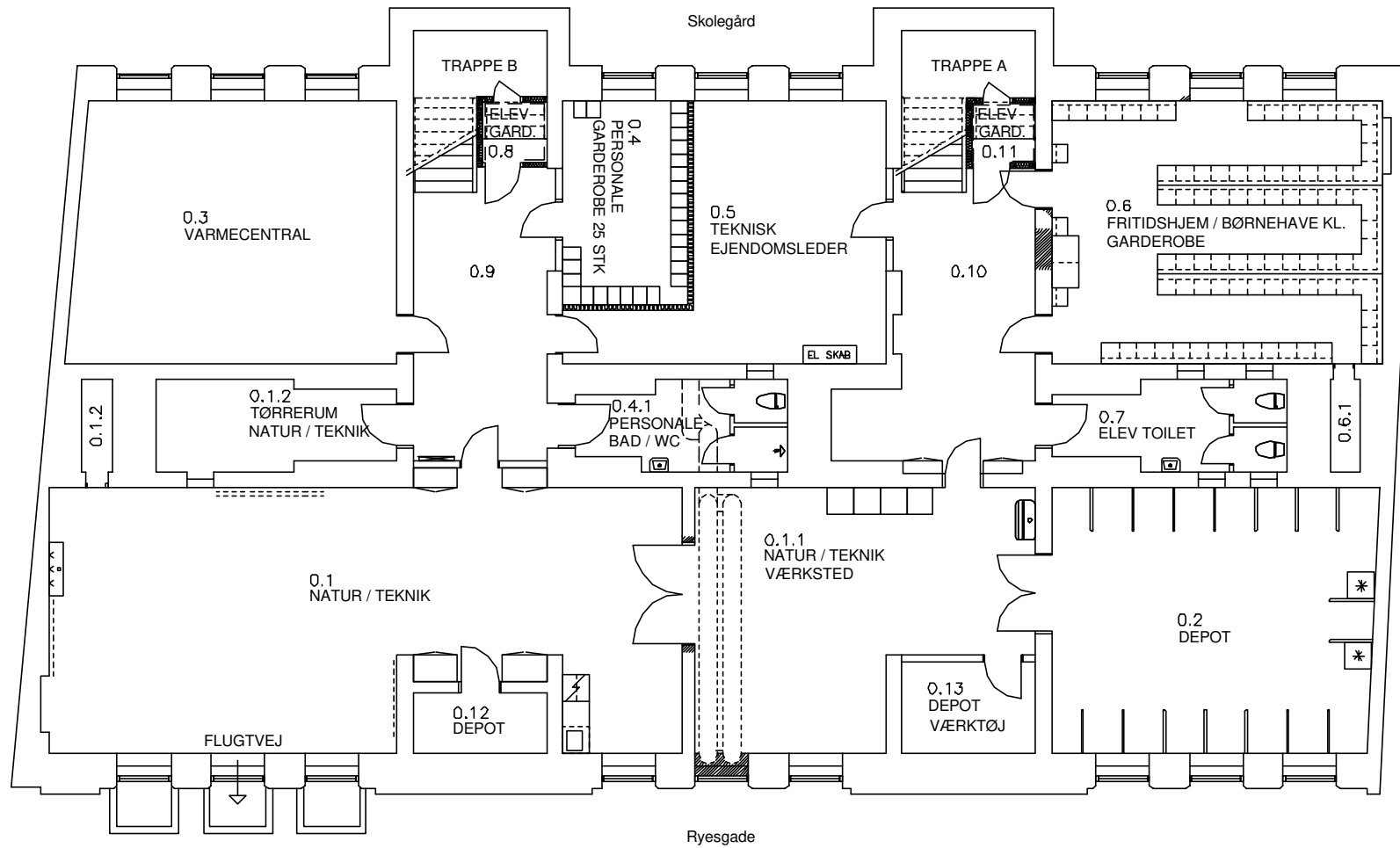
KÆLDERPLAN
