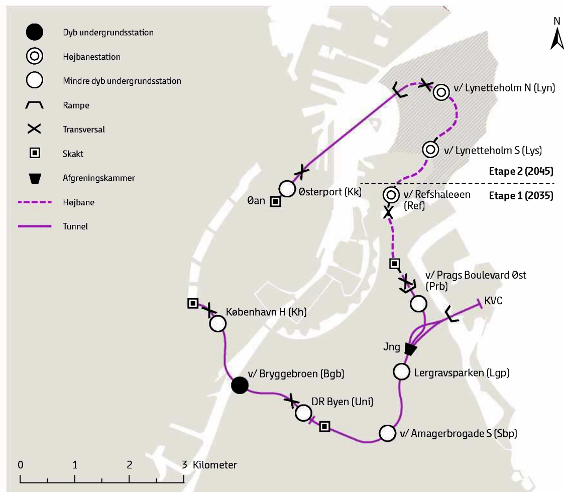
Figur 13.2 Skitse af Sydlig Løsning.
