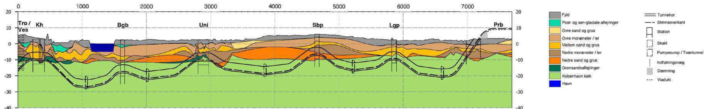
Figur 4.26 Opdateret længdeprofil mellem København H (Kh) og v/ Prags Boulevard Øst (Prb).
