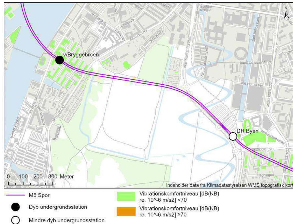
Figur B.28 Vibrationskort for vibrationskomfort ved drift af M5 på strækningen v/ Bryggebroen – DR Byen.
