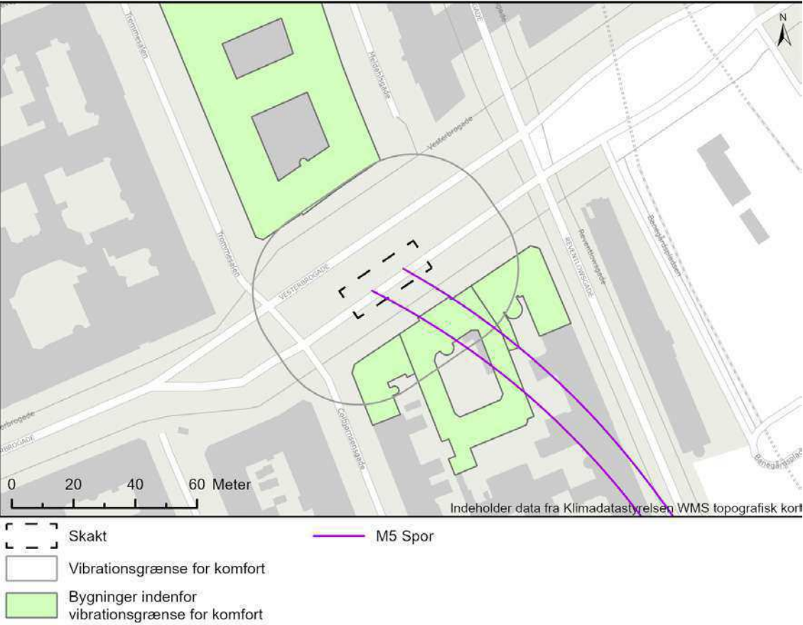
Figur B.14 Vibrationskort for vibrationskomfort ved etablering af byggegrubeindfatning ved boring af sekantpæle ved Vesterbrogade (Vbg).
