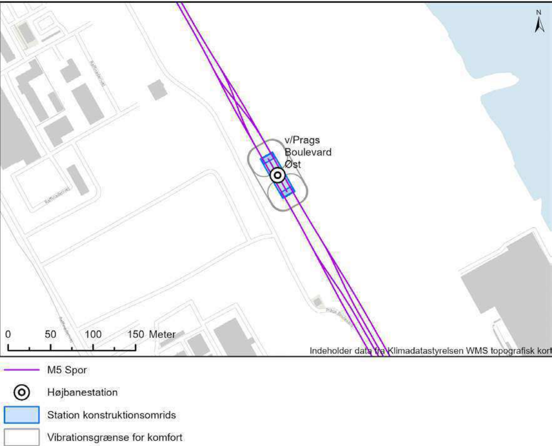
Figur B.23 Vibrationskort for vibrationskomfort ved etablering af fundament til højbanestation ved Prags Boulevard (Prb).
