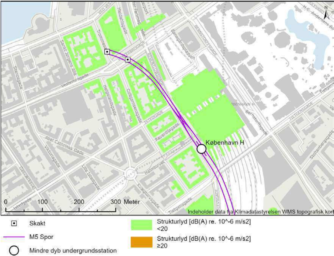
Figur B.33 Vibrationskort for strukturlyd ved drift af M5 på strækningen Trommesalen – København H.
