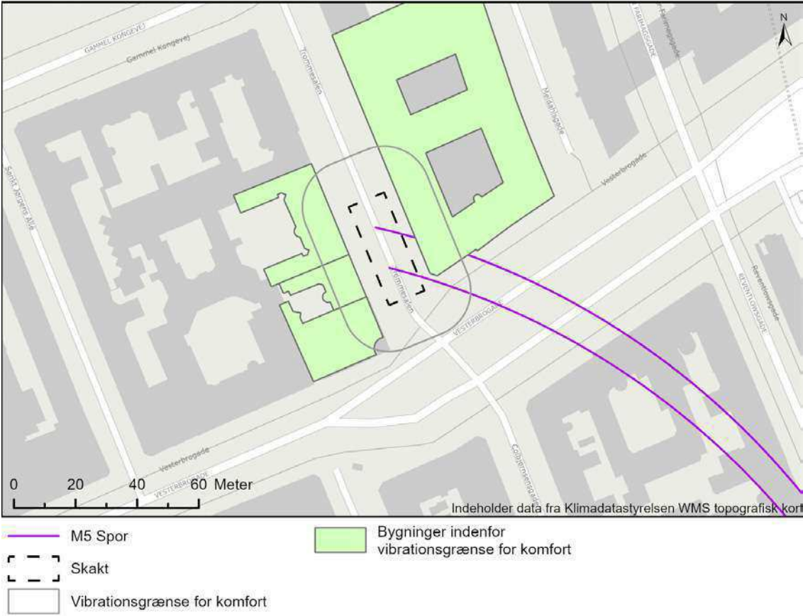
Figur B.15 Vibrationskort for vibrationskomfort ved etablering af byggegrubeindfatning ved forgravning og nedvibrering af spuns ved Trommesalen (Tro).
