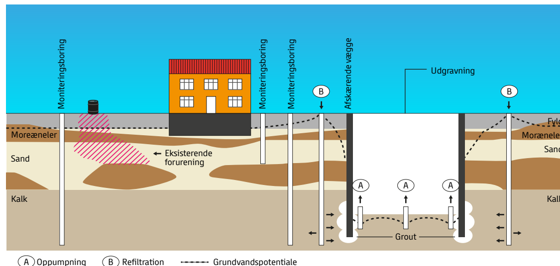
Figur 11.2 Princip for grundvandshåndtering.
