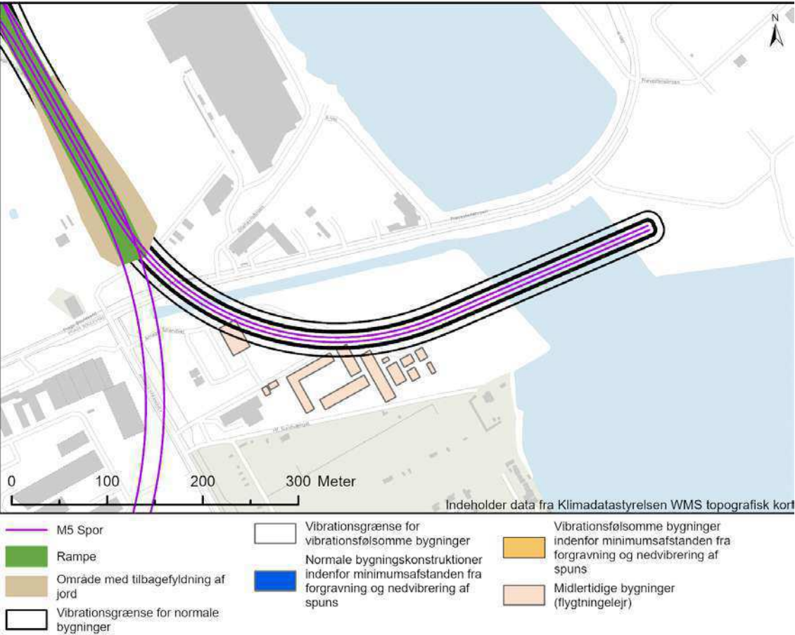
Figur B.12 Vibrationskort for bygningsskadelige vibrationer ved etablering af fundament til viadukten fra v/ Prags Boulevard Øst (Prb) til KVC på Prøvestenen.
