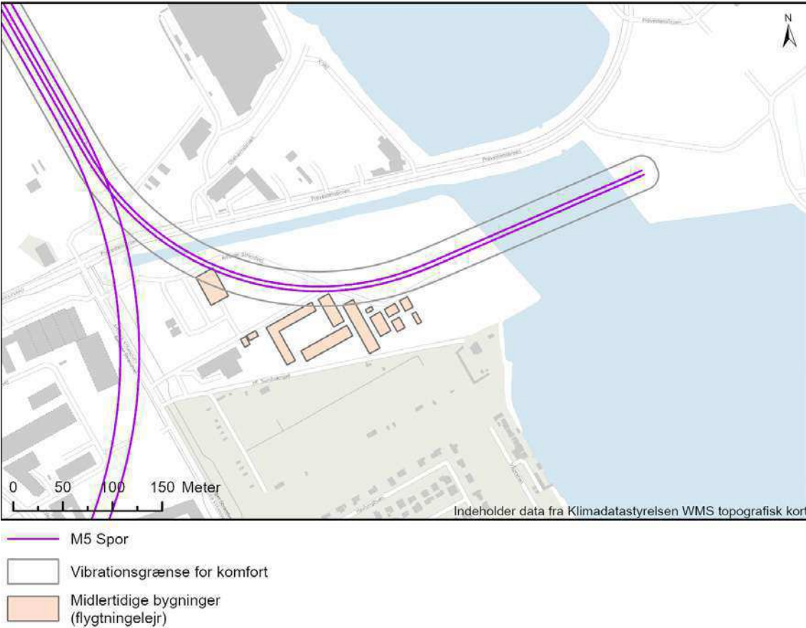
Figur B.24 Vibrationskort for vibrationskomfort ved etablering af fundament til viadukten fra Prags Boulevard (Prb) til KVC på Prøvestenen.
