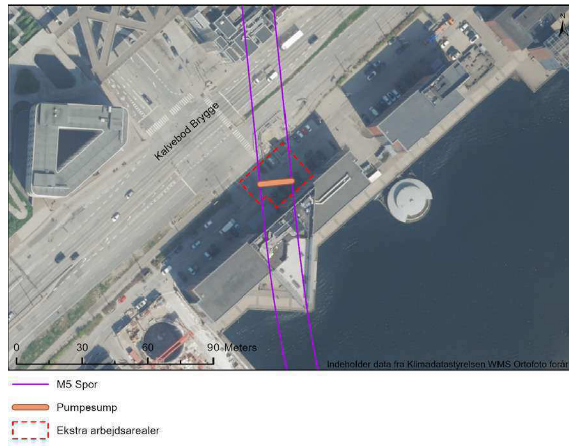
Figur 6.6 Byggeplads ved Kalvebod Brygge.
