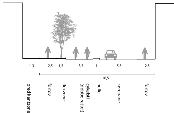
Vejtype B2 Vejbredde: 16.5 m
