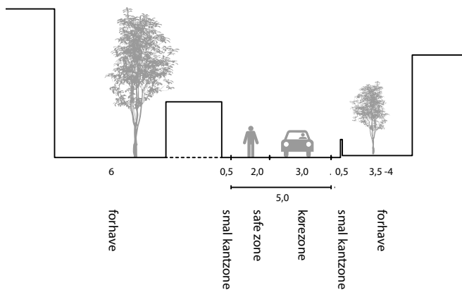
Vejtype C Vejbredde: 5 m
