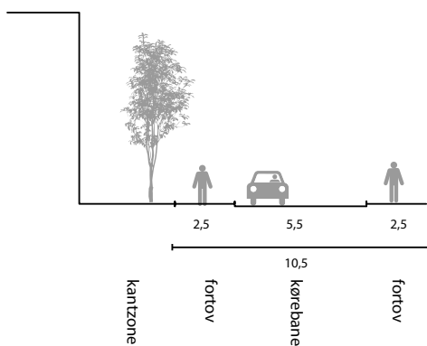
Vejtype B1 Vejbredde: 10.5 m
