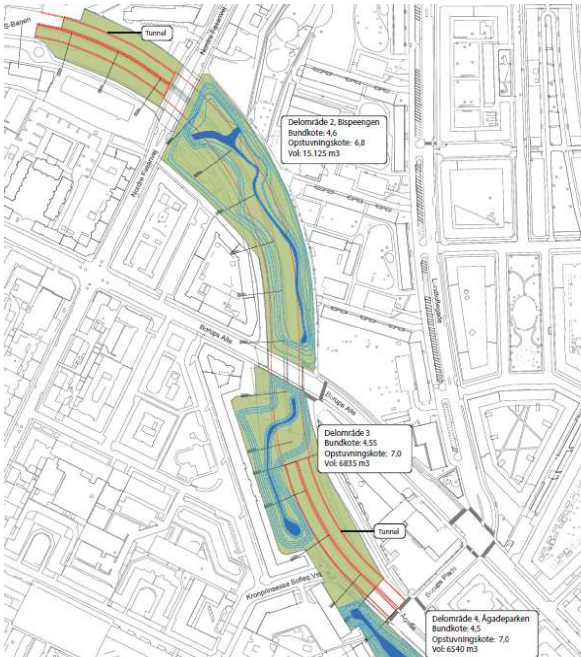
Figur 15. Mulig placering af bassinvolumen på terrænen. Kilde: Rambøll, Bilag 3 til rapport "Bispeengen – skybrudssikring, volumenanalyse", juni 2018, udført for Miljøpunkt Nørrebro.
