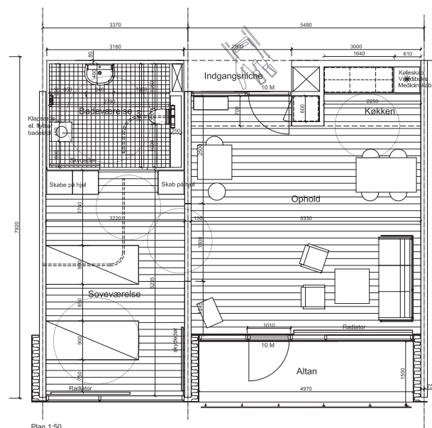
Plan 1:50 Lejlighedstype: Dobbeltbolig Bruttoareal 61,3 m 2 .
