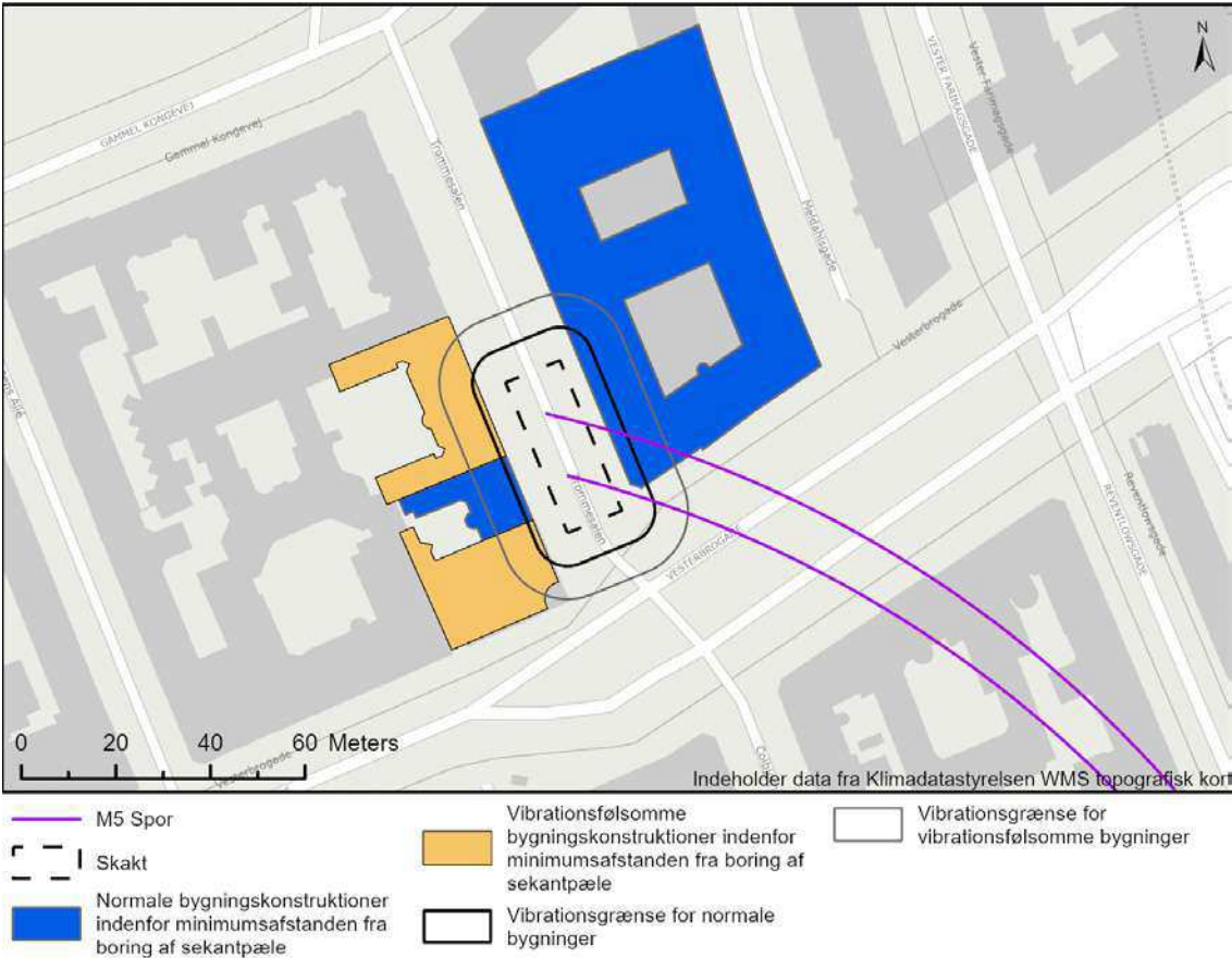
Figur B.1 Vibrationskort for bygningsskadelige vibrationer ved etablering af byggegrubeindfatning ved boring af sekantpæle ved Trommesalen (Tro).
