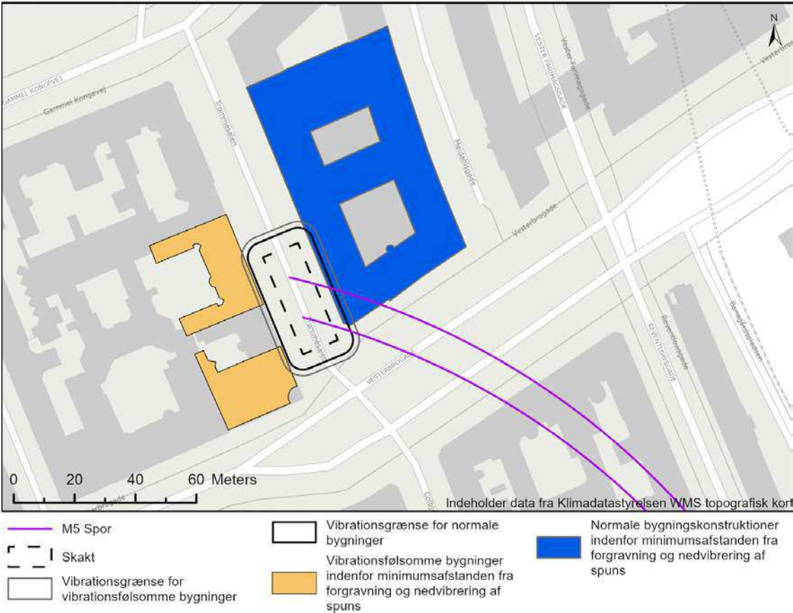
Figur B.3 Vibrationskort for bygningsskadelige vibrationer ved etablering af byggegrubeindfatning ved forgravning og nedvibrering af spuns ved Trommesalen (Tro).
