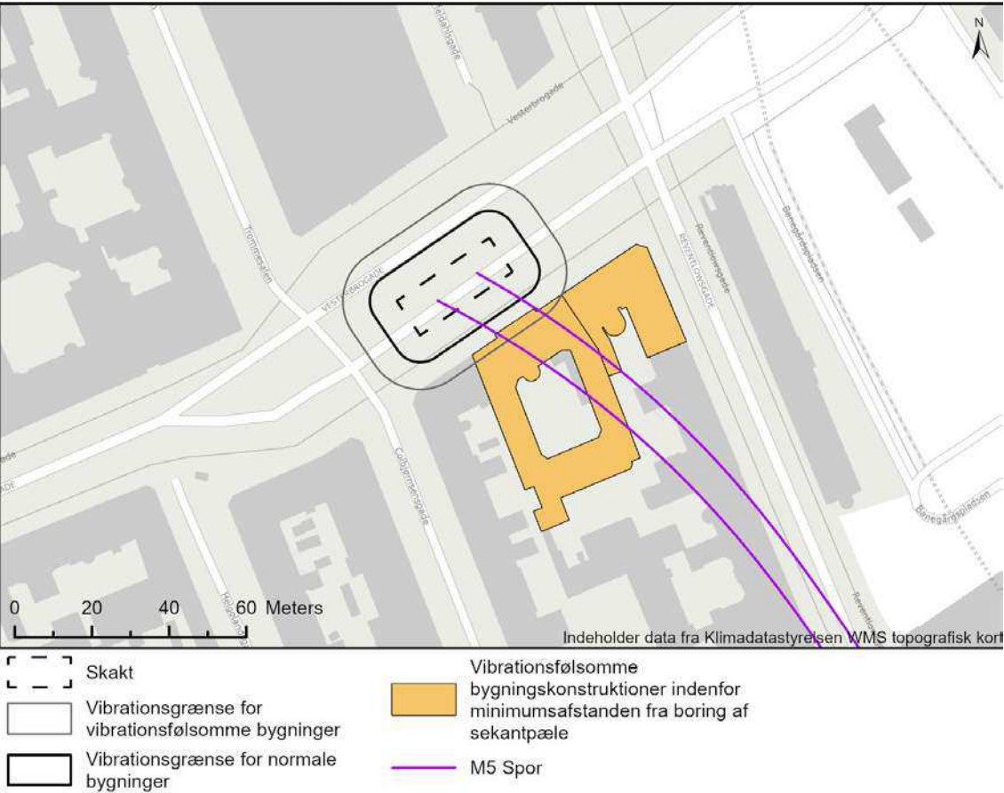
Figur B.2 Vibrationskort for bygningsskadelige vibrationer ved etablering af byggegrubeindfatning ved boring af sekantpæle ved Vesterbrogade (Vbg).
