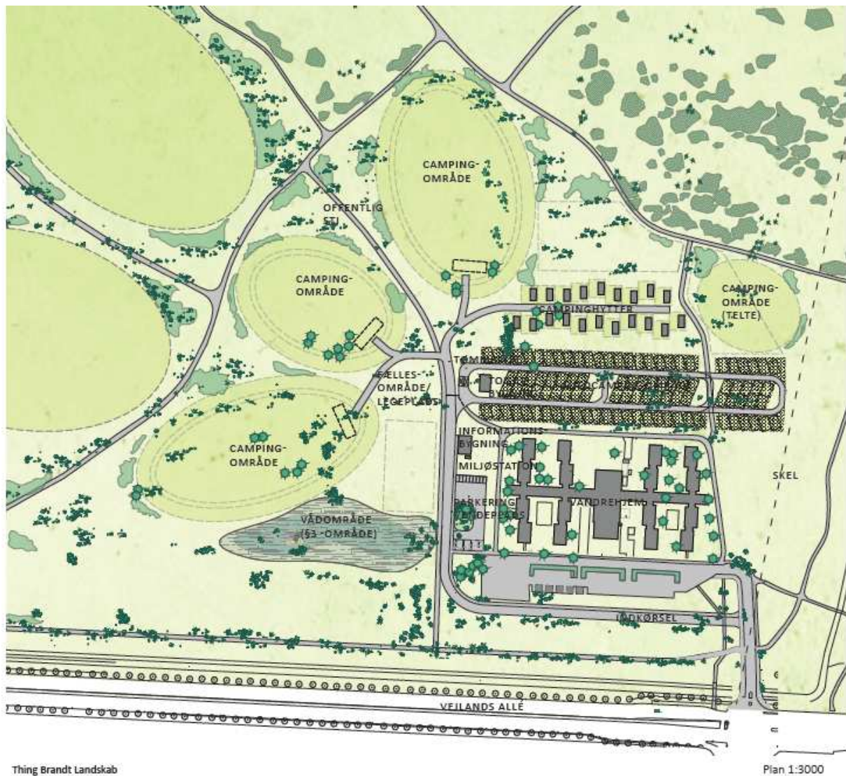
Figur 1: Lokalplanområdets indretning.
