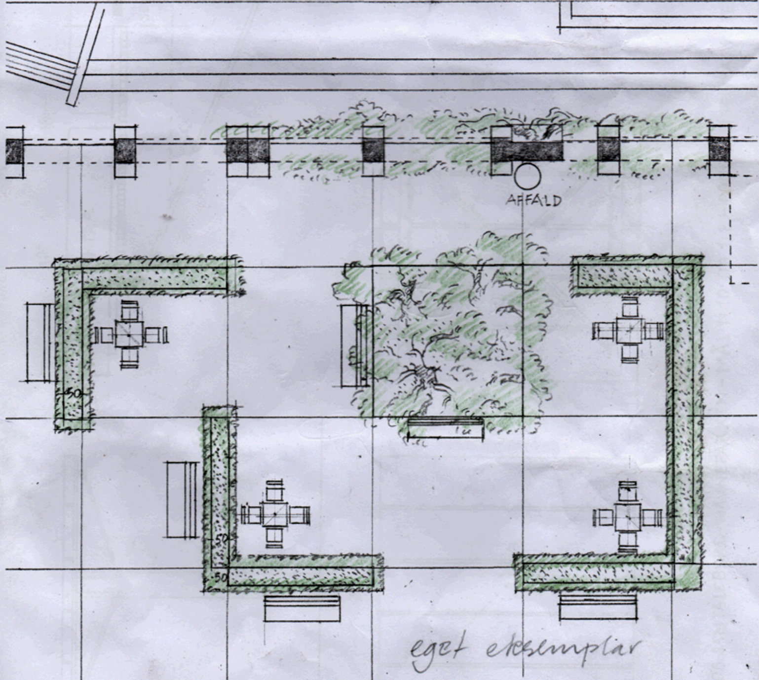
OMRÅDEPLAN 1:500
